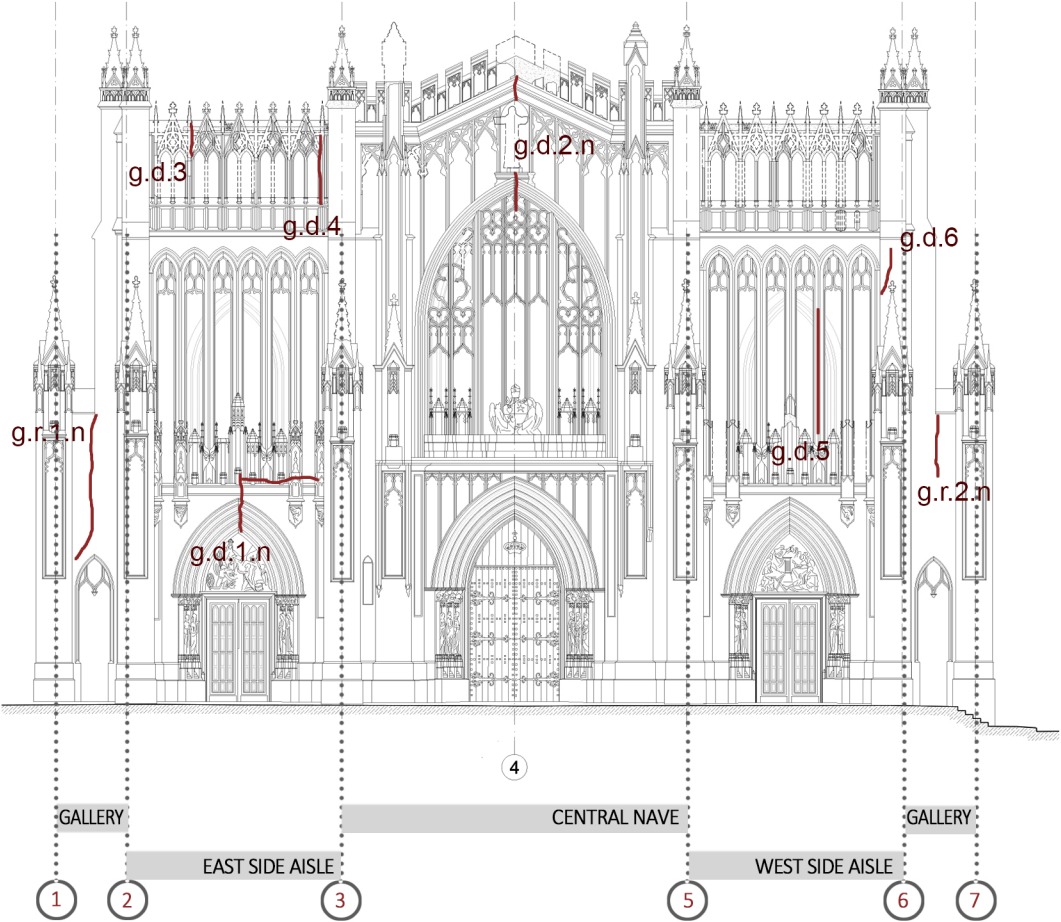
ELEVACIÓN LADO NORTE, EJE B
