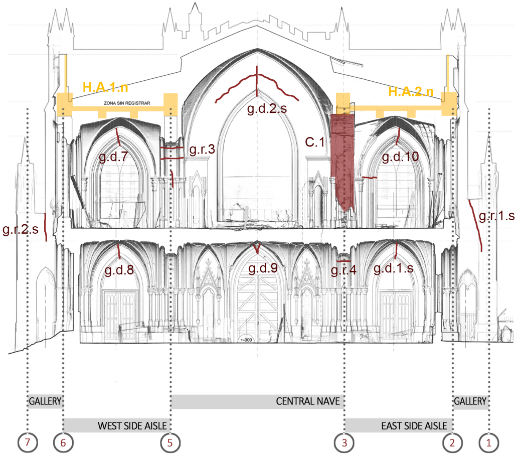
ELEVACIÓN LADO SUR, EJE B
