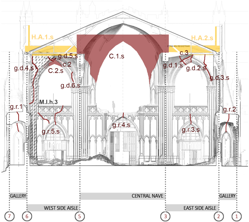
ELEVACIÓN LADO SUR, EJE C
