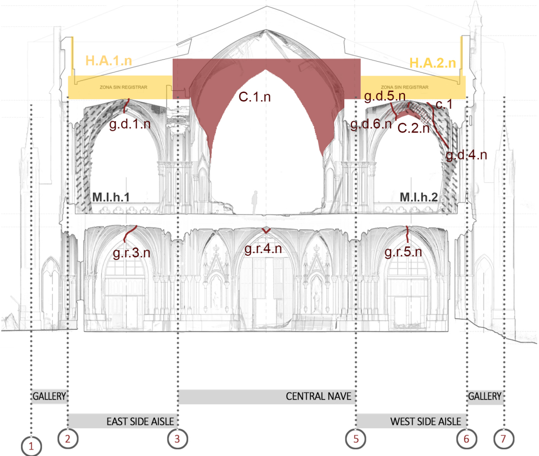
ELEVACIÓN LADO NORTE, EJE C
