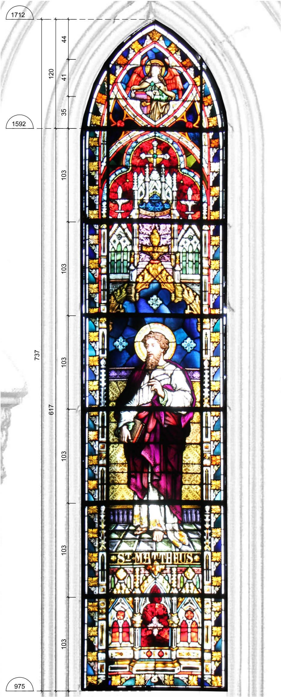
Elevación Esc. 1/25
