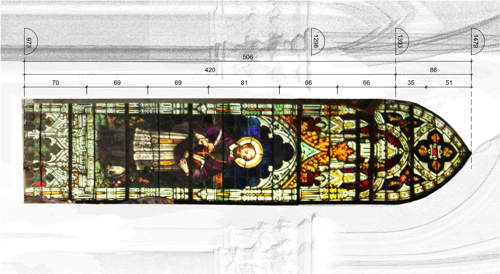
Elevación Esc. 1/25
