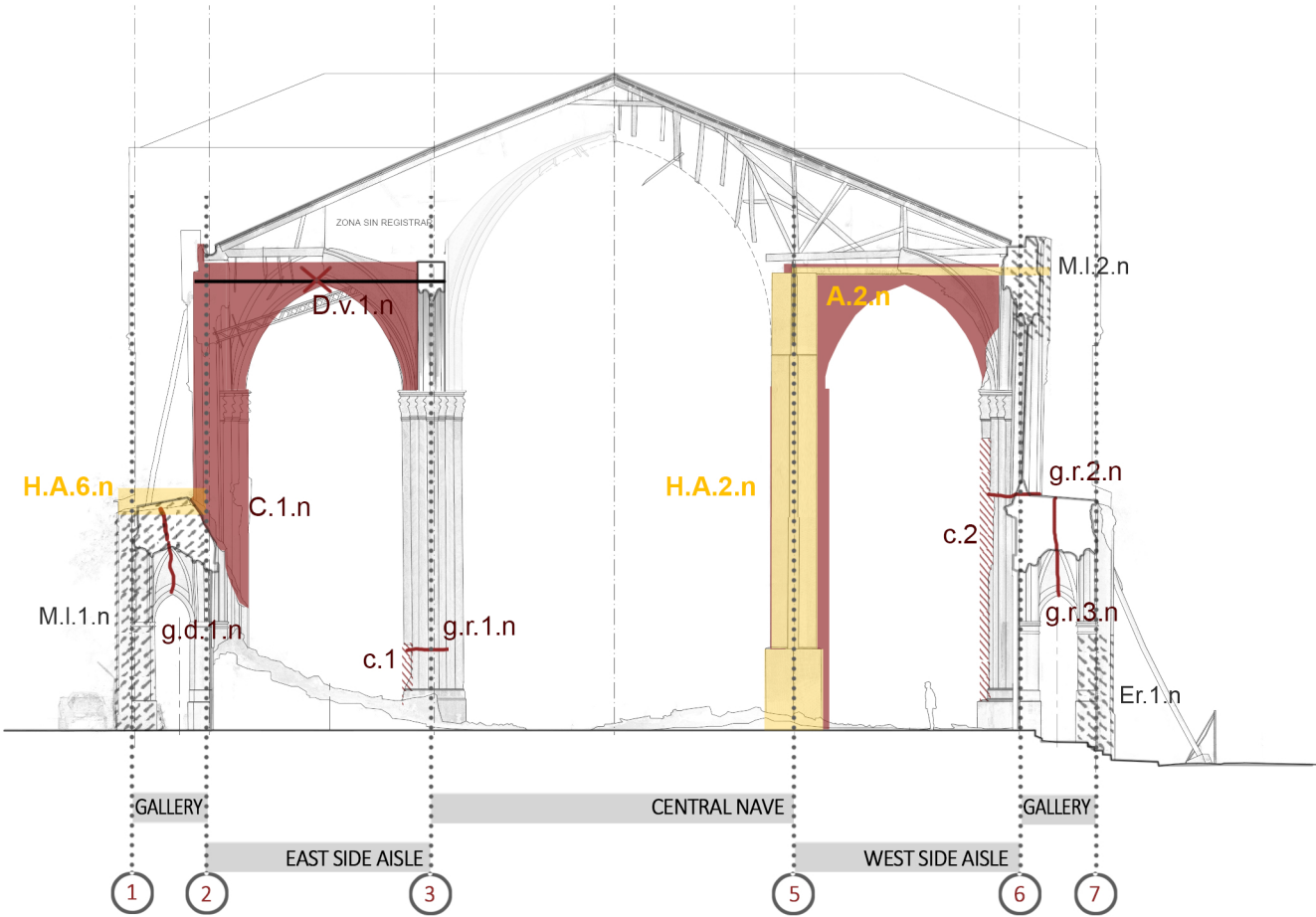
ELEVACIÓN LADO NORTE, EJE F
