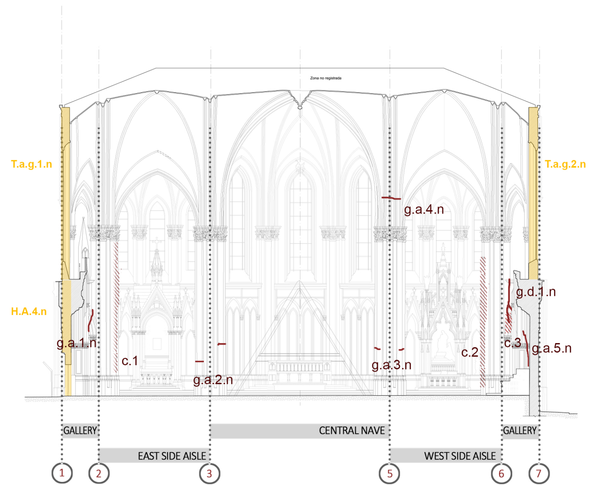
ELEVACIÓN LADO NORTE, EJE I
