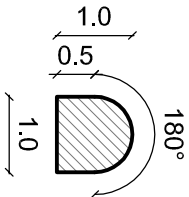
DETALLE MOLDURA #3 Esc. 1/1
