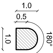
DETALLE MOLDURA #3 Esc. 1/1
