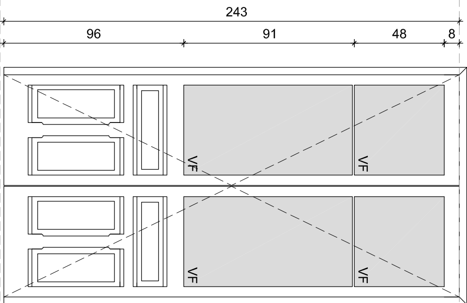
Pu 09 - INTERIOR Esc. 1/20
