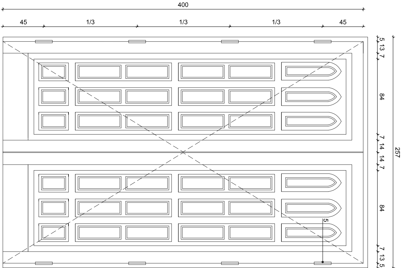
ELEVACIÓN EXTERIOR Esc. 1/25
