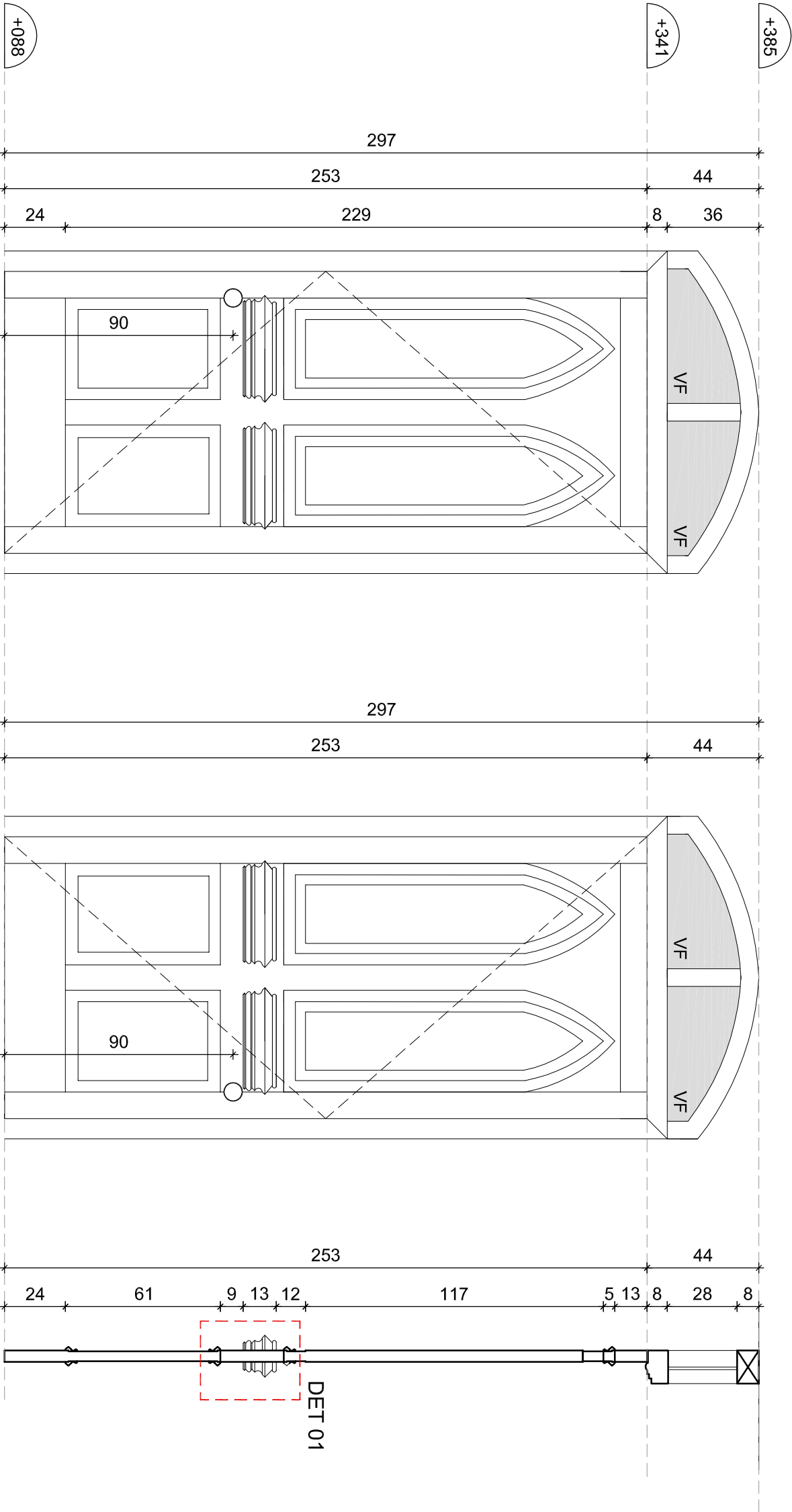
ELEVACIÓN INT. Esc. 1/20
