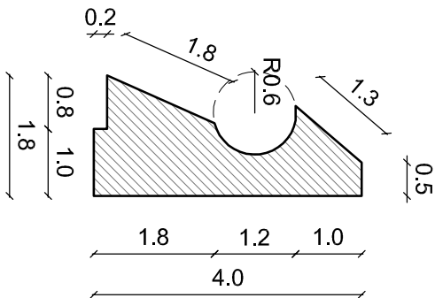
DETALLE MOLDURA #xx Esc. 1/1
