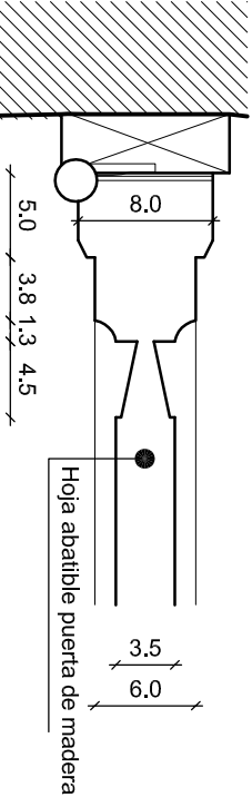
DETALLE 1 Esc. 1/5
