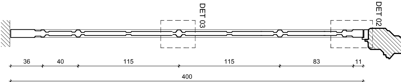
CORTE Esc. 1/25
