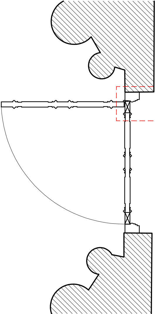
PLANTA Esc. 1/20
