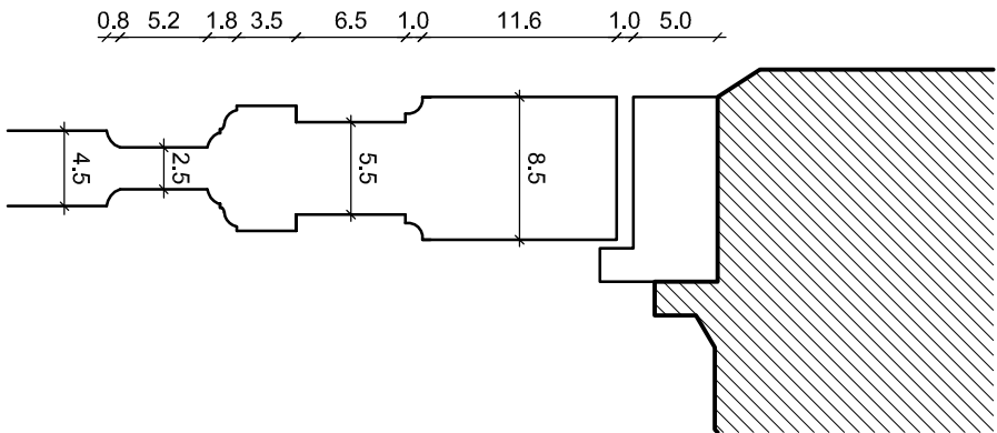
DETALLE 03 Esc. 1/5
