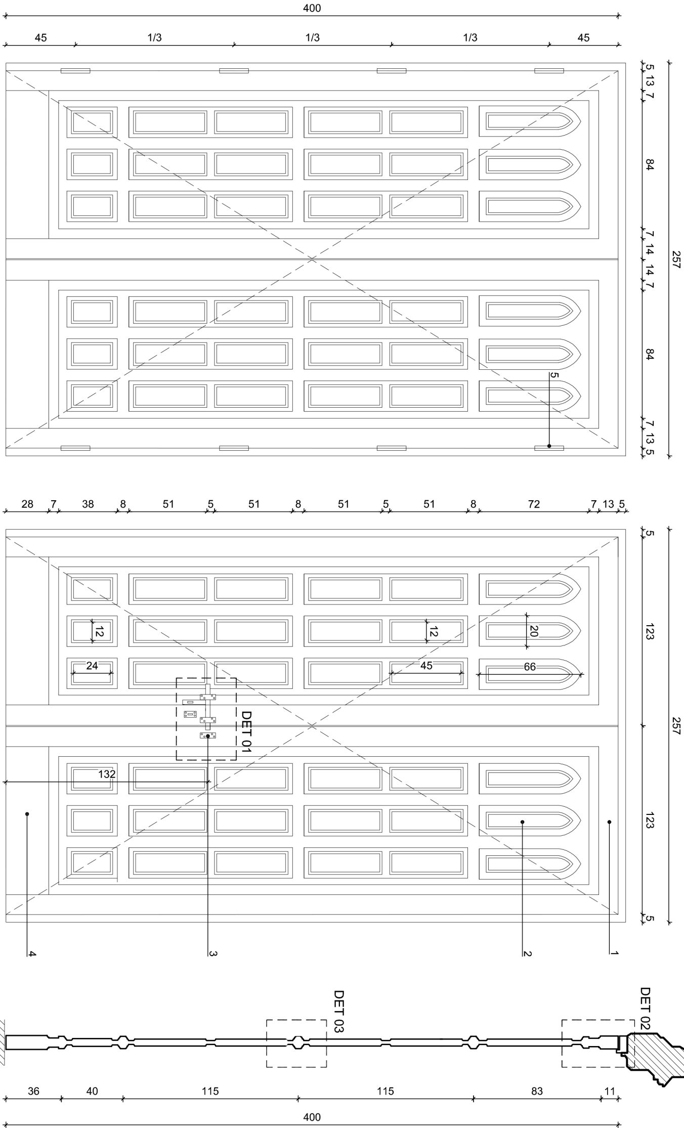
ELEVACIÓN EXTERIOR Esc. 1/25
