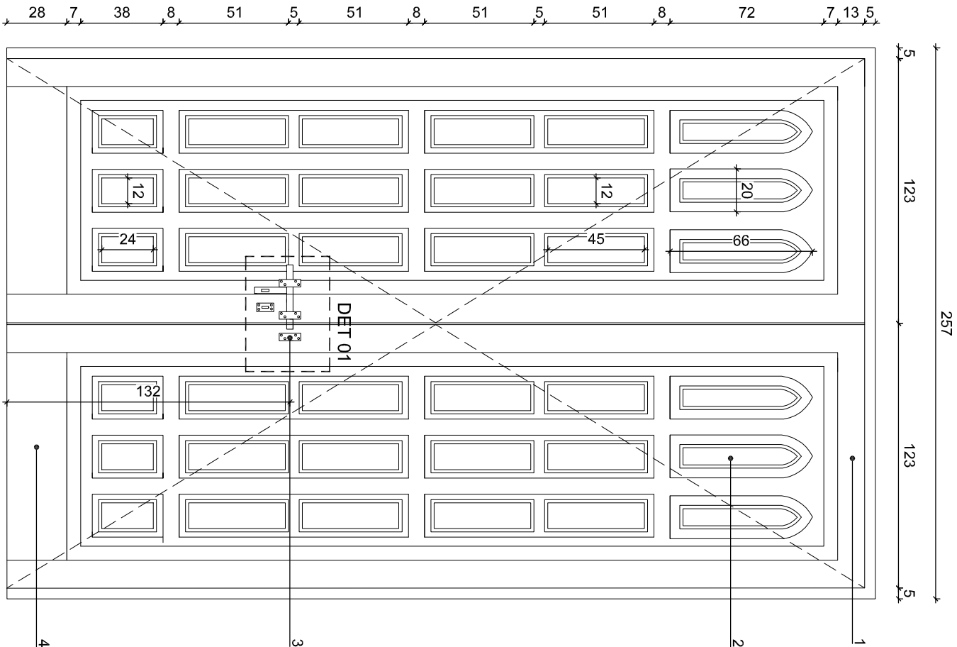
ELEVACIÓN INTERIOR Esc. 1/25
