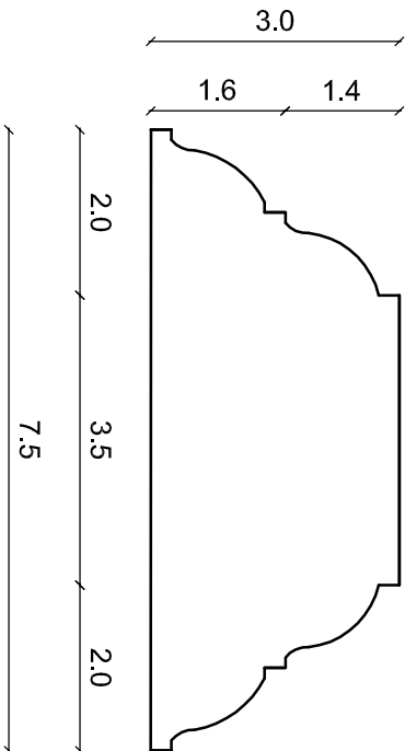
DETALLE 04 Esc. 1/1
