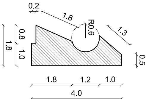
DETALLE MOLDURA Esc. 1/1
