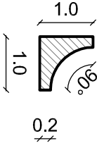
DETALLE MOLDURA #1 Esc. 1/1
