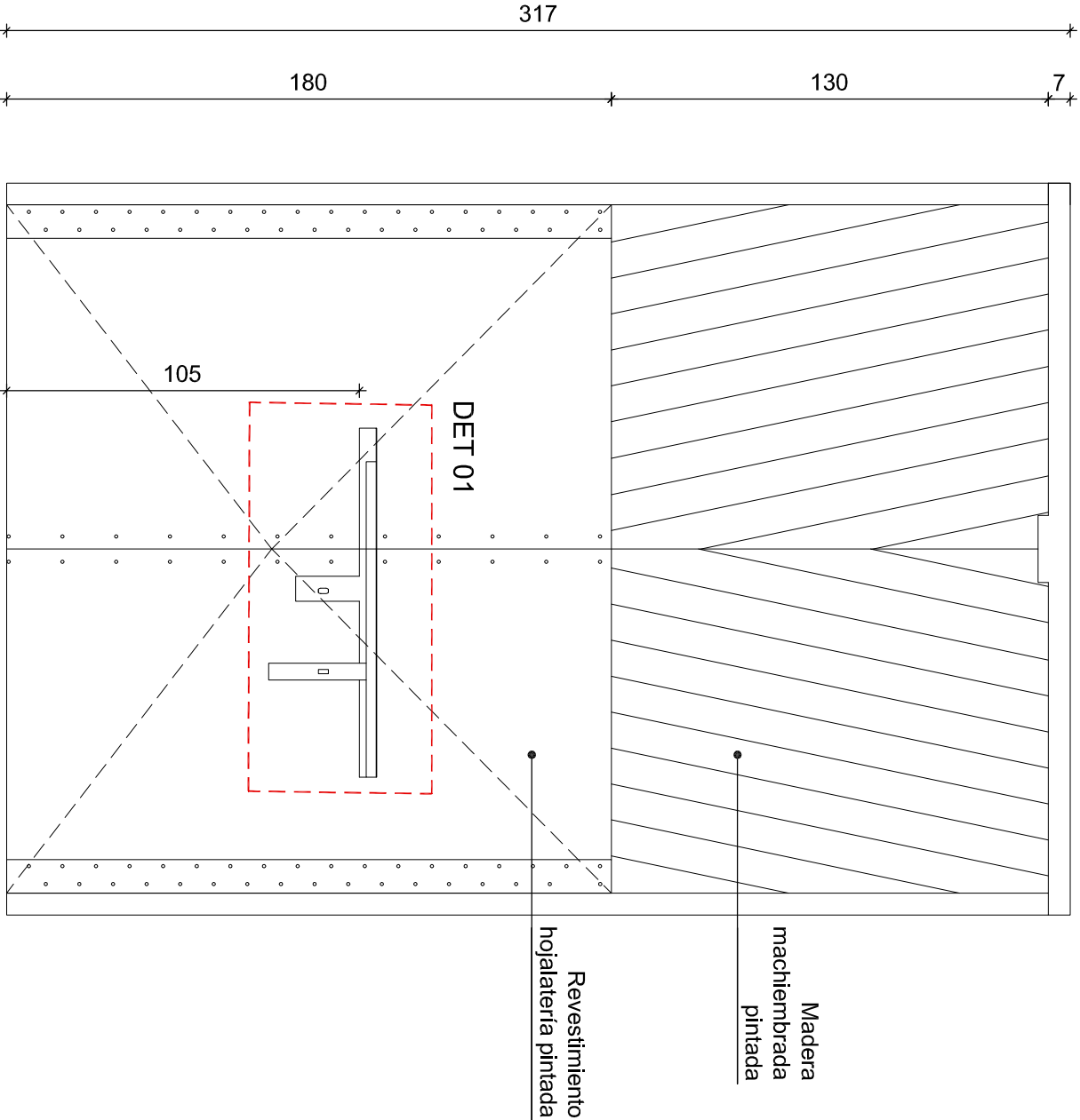
CORTE Esc. 1/20
