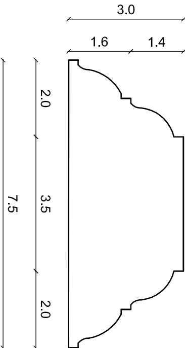
DETALLE 04 Esc. 1/1
