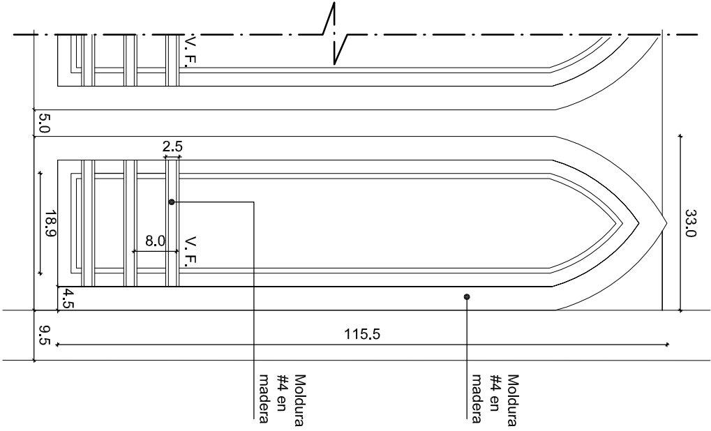
DETALLE 01 Esc. 1/2
