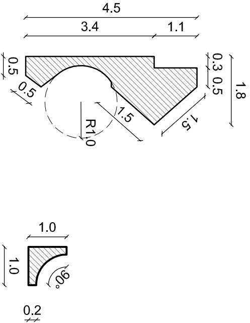
DETALLE MOLDURA #1 Esc. 1/1
