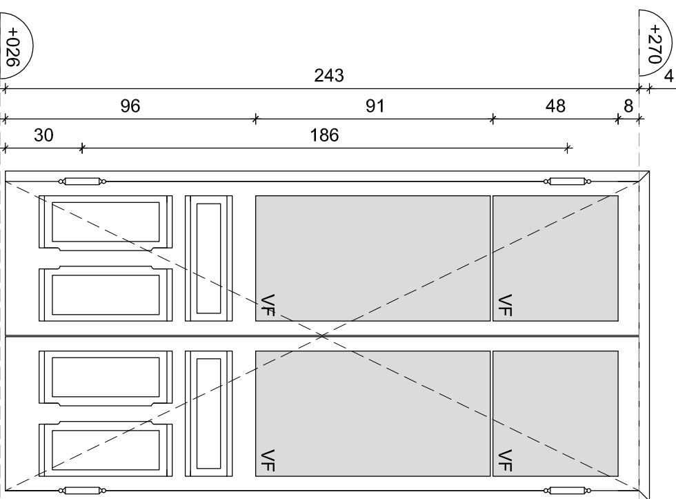
Pu 08 - EXT. Esc. 1/20
