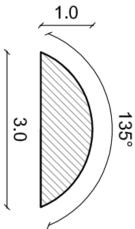
DETALLE MOLDURA Esc. 1/1
