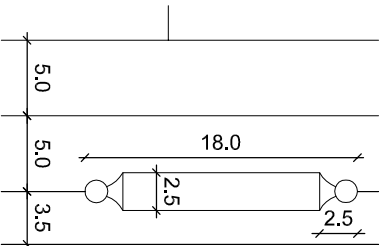
DETALLE 1 Esc. 1/5
