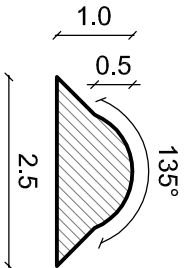
DETALLE MOLDURA #4 Esc. 1/1
