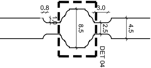
DETALLE 02 Esc. 1/5
