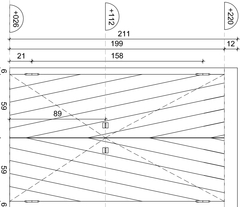
Pu 08 - EXT. Esc. 1/20
