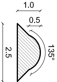
DETALLE MOLDURA #4 Esc. 1/1
