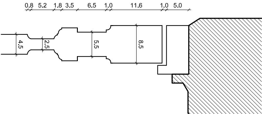
DETALLE 03 Esc. 1/5
