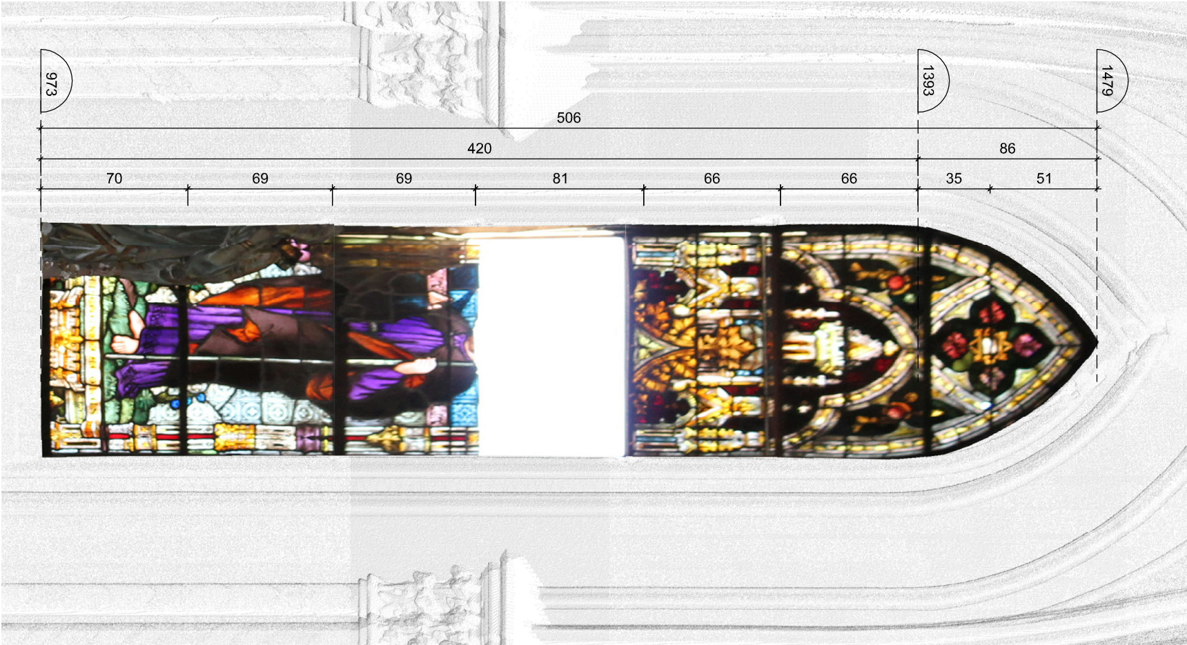
Elevación Esc. 1/25
