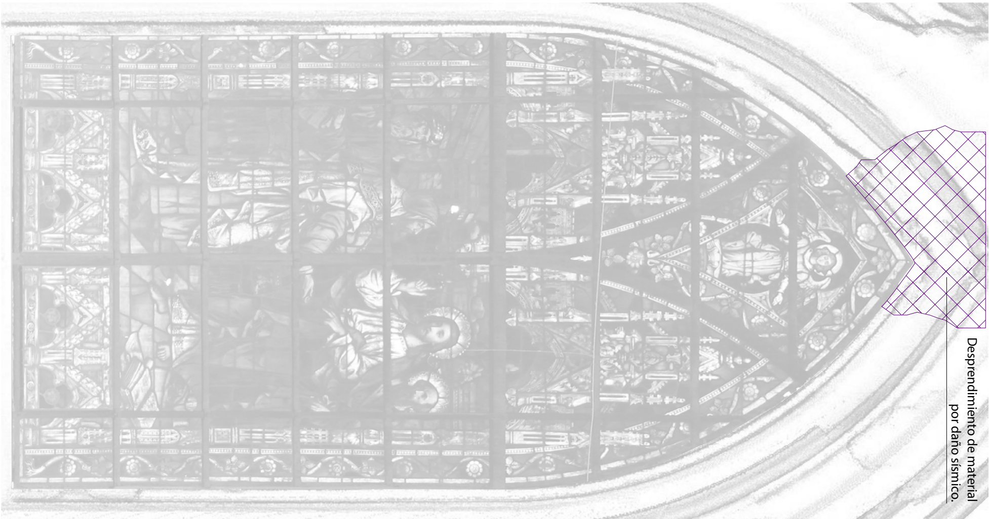
Levantamiento de Daños - Esc. 1/25
