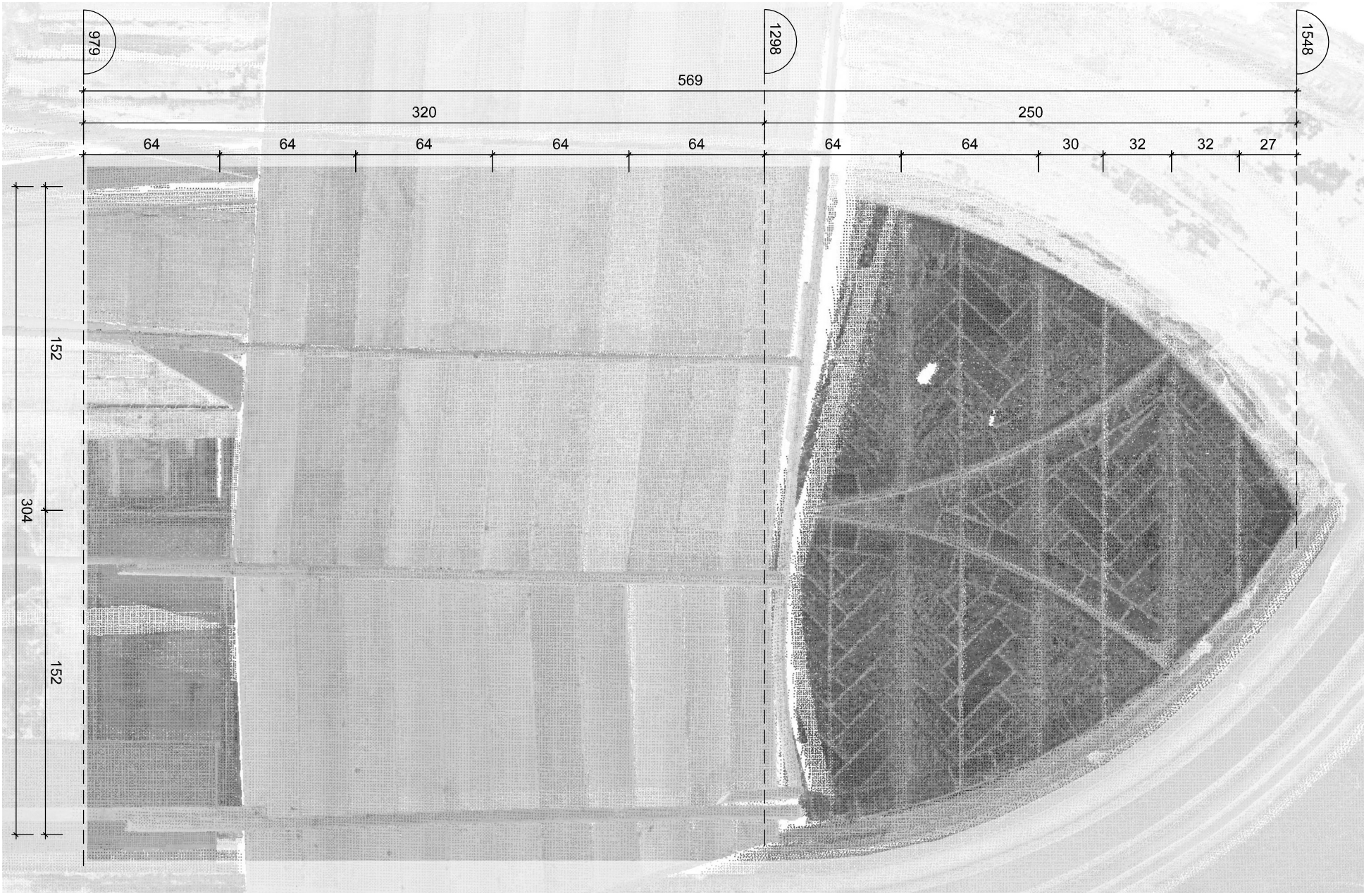
Elevación - Esc. 1/25
