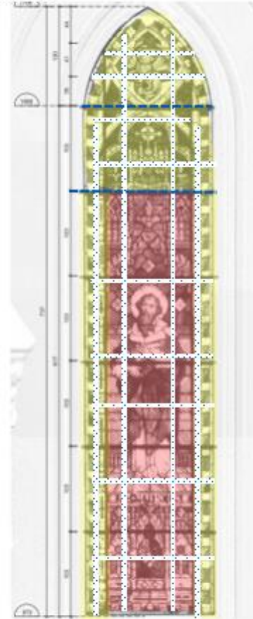
Registro esquemático de la intervención durante las faenas de Restauración y reforzamiento.
