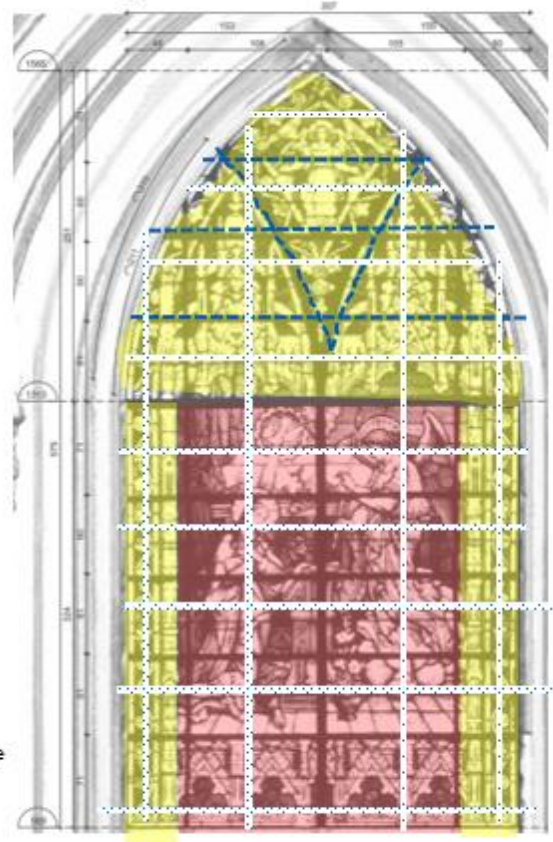
Registro esquemático de la intervención durante las faenas de Restauración y reforzamiento.
