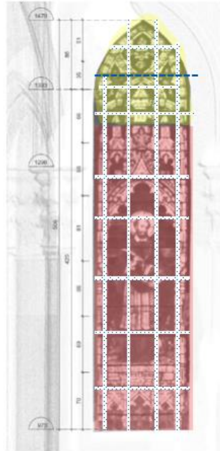
Registro esquemático de la intervención durante las faenas de Restauración y reforzamiento.
