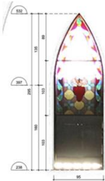
Registro fotográfico Vitral 2.
