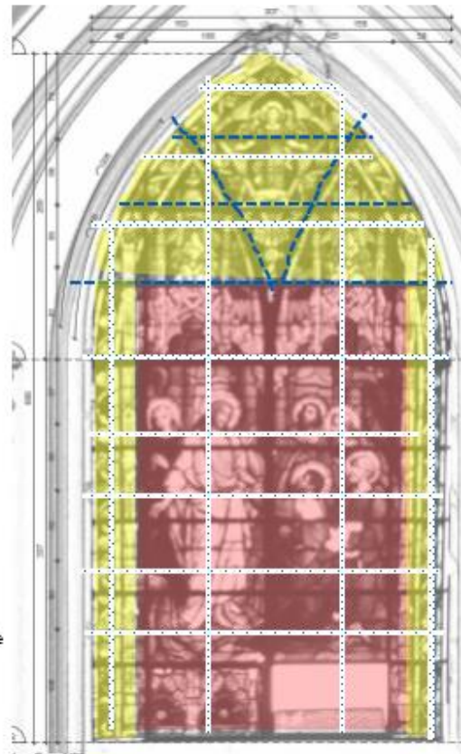
Registro esquemático de la intervención durante las faenas de Restauración y reforzamiento.
