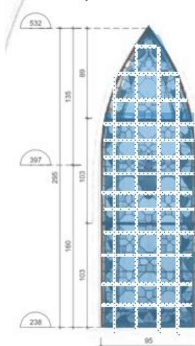
Registro esquemático de la intervención durante las faenas de Restauración y reforzamiento.
