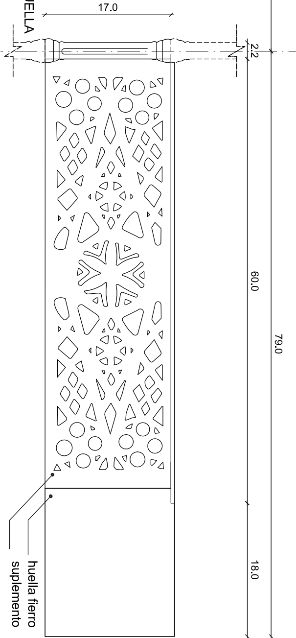
DETALLE APOYO HUELLO TIPO Esc. 1/5
