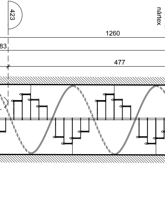
DETALLE HUELLO TIPO Esc. 1/10
