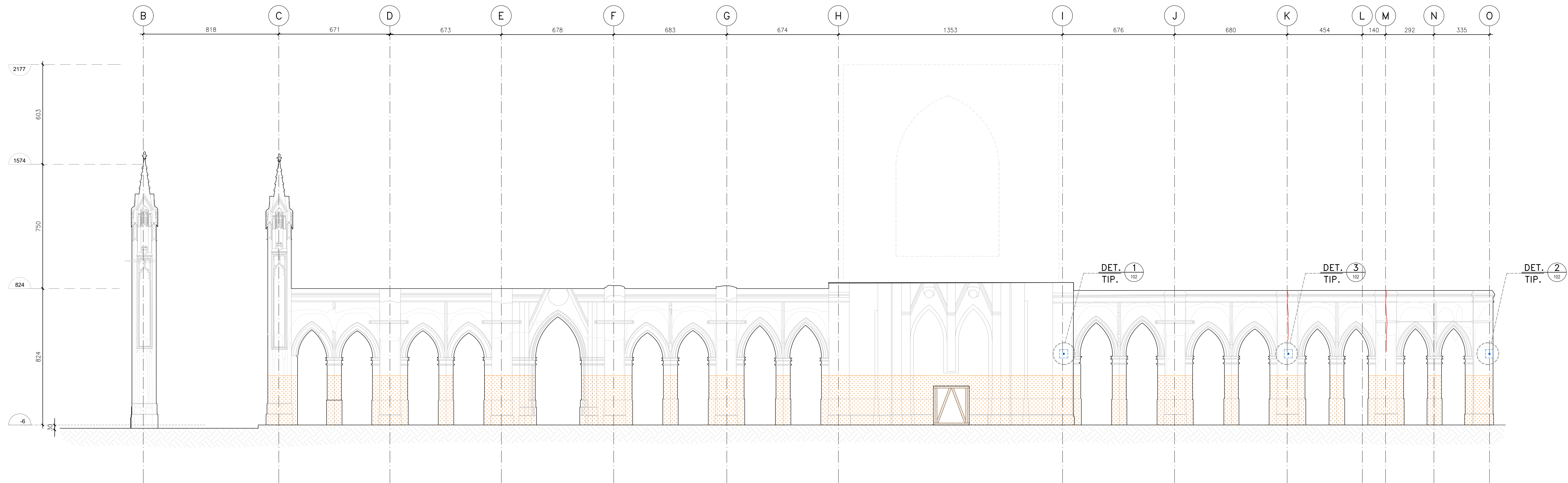
ELEVACION EJE 1 ESCALA 1:100
