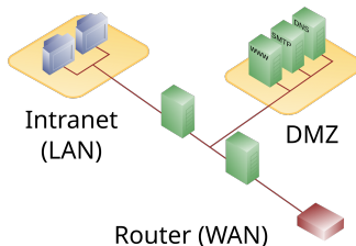
zweistufige DMZ
