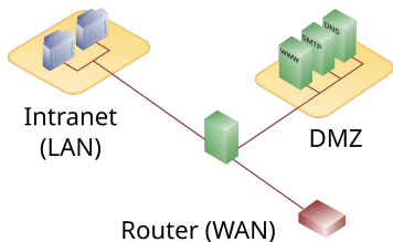
einstufige DMZ
