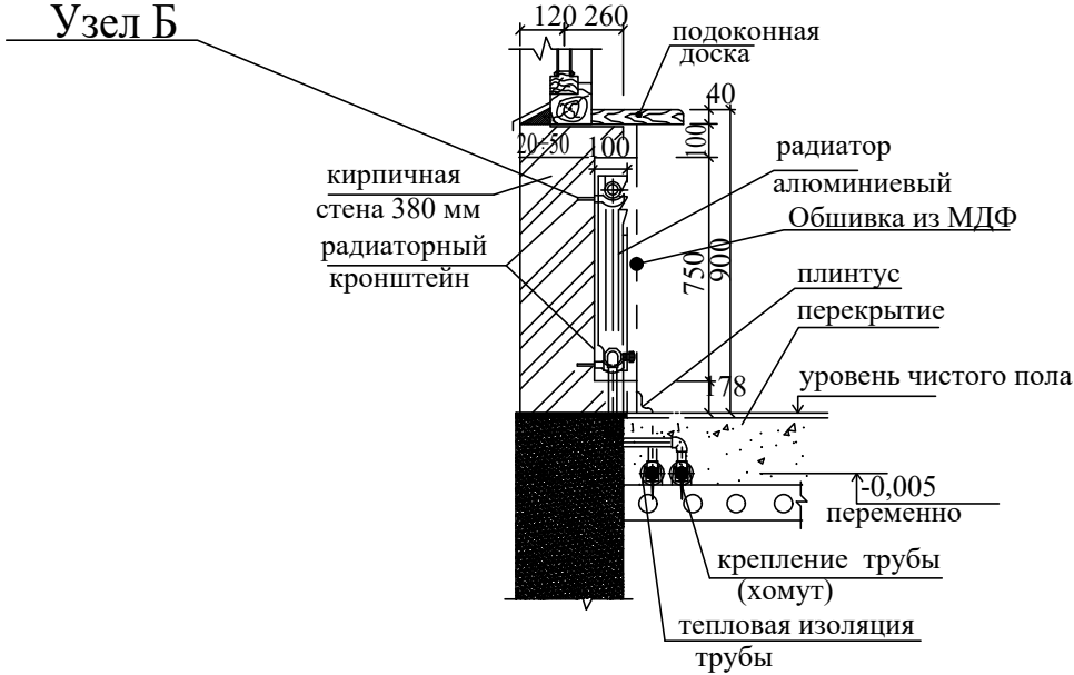
Схема прокладки труб в конструкции пола
