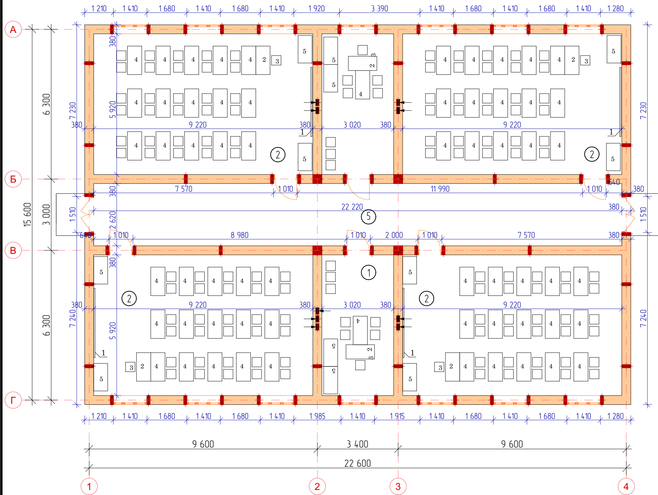
План расположения технологического оборудования
