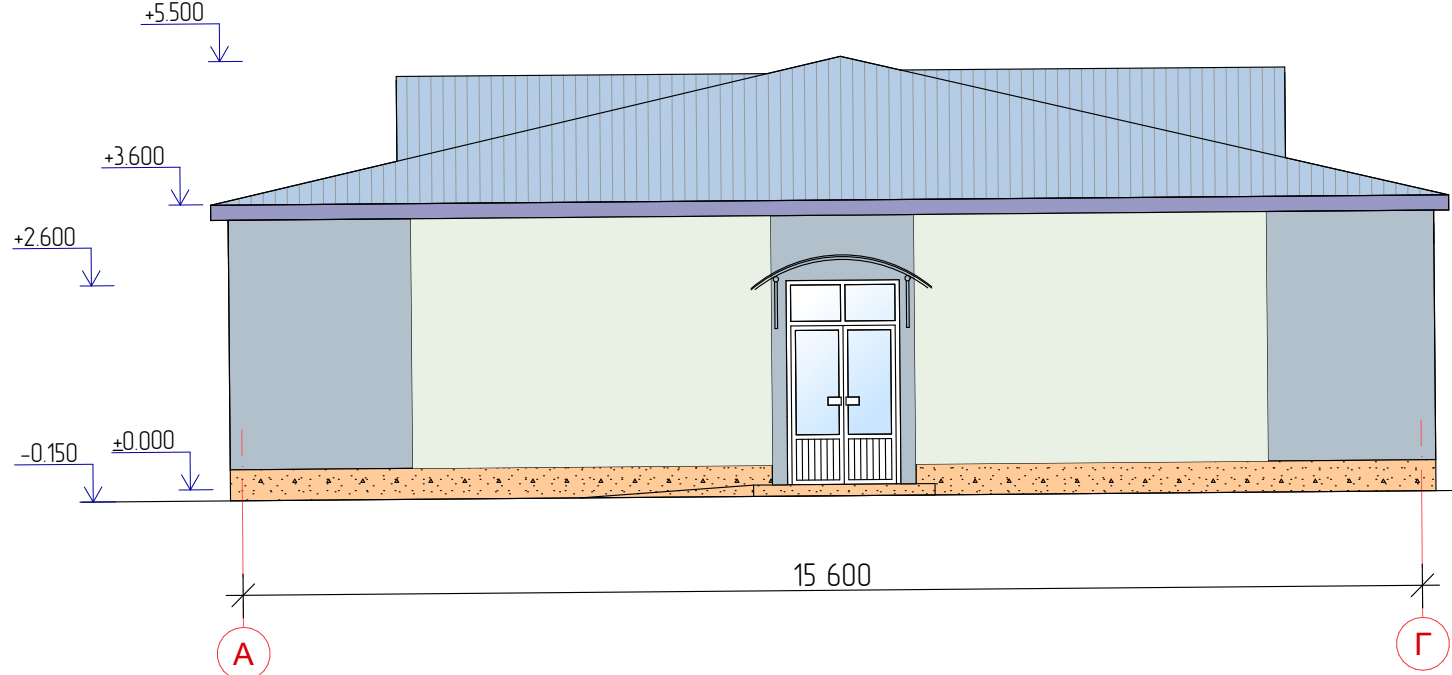
Фасад в осях "А"-Г по оси „1"
