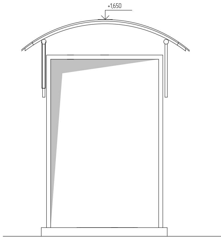
Козырек крыльца КЗ-1
