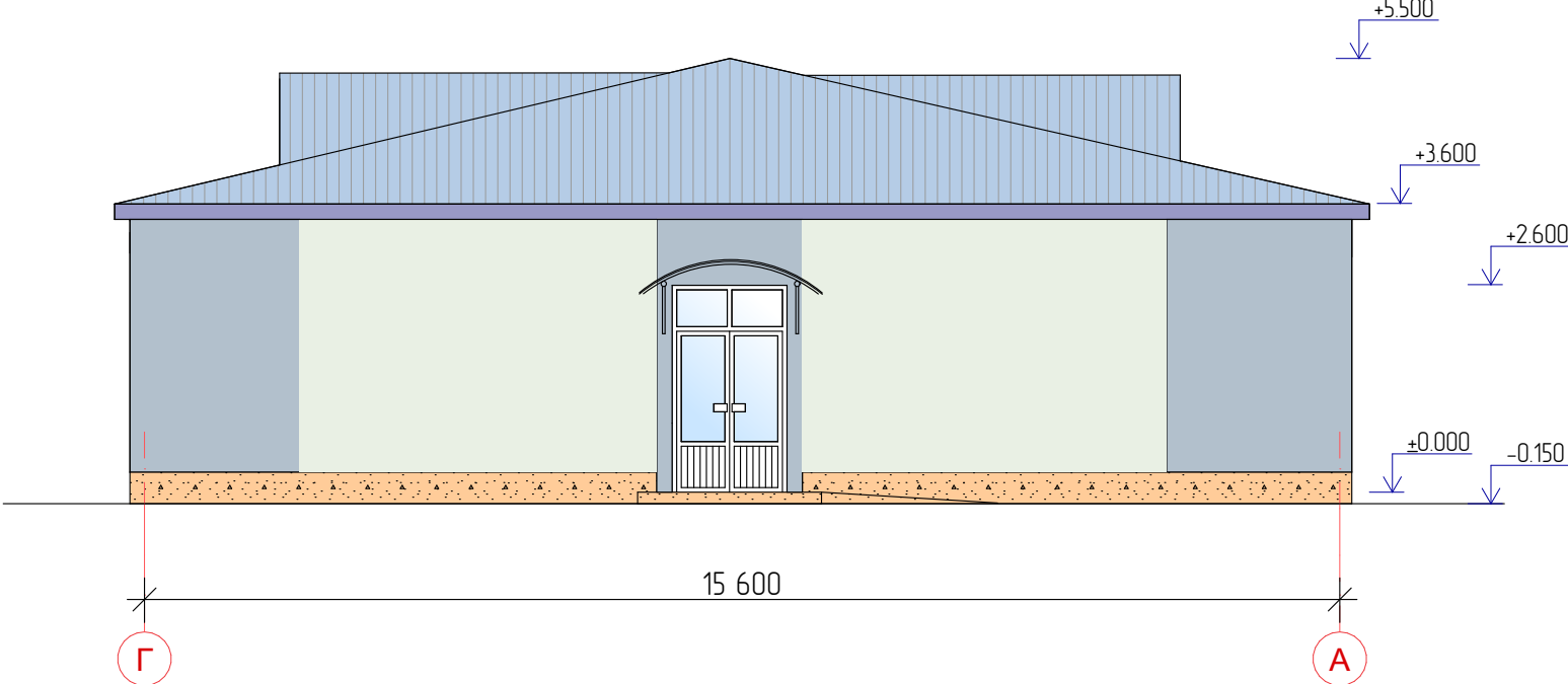
Фасад в осях "Г"-А по оси „4"
