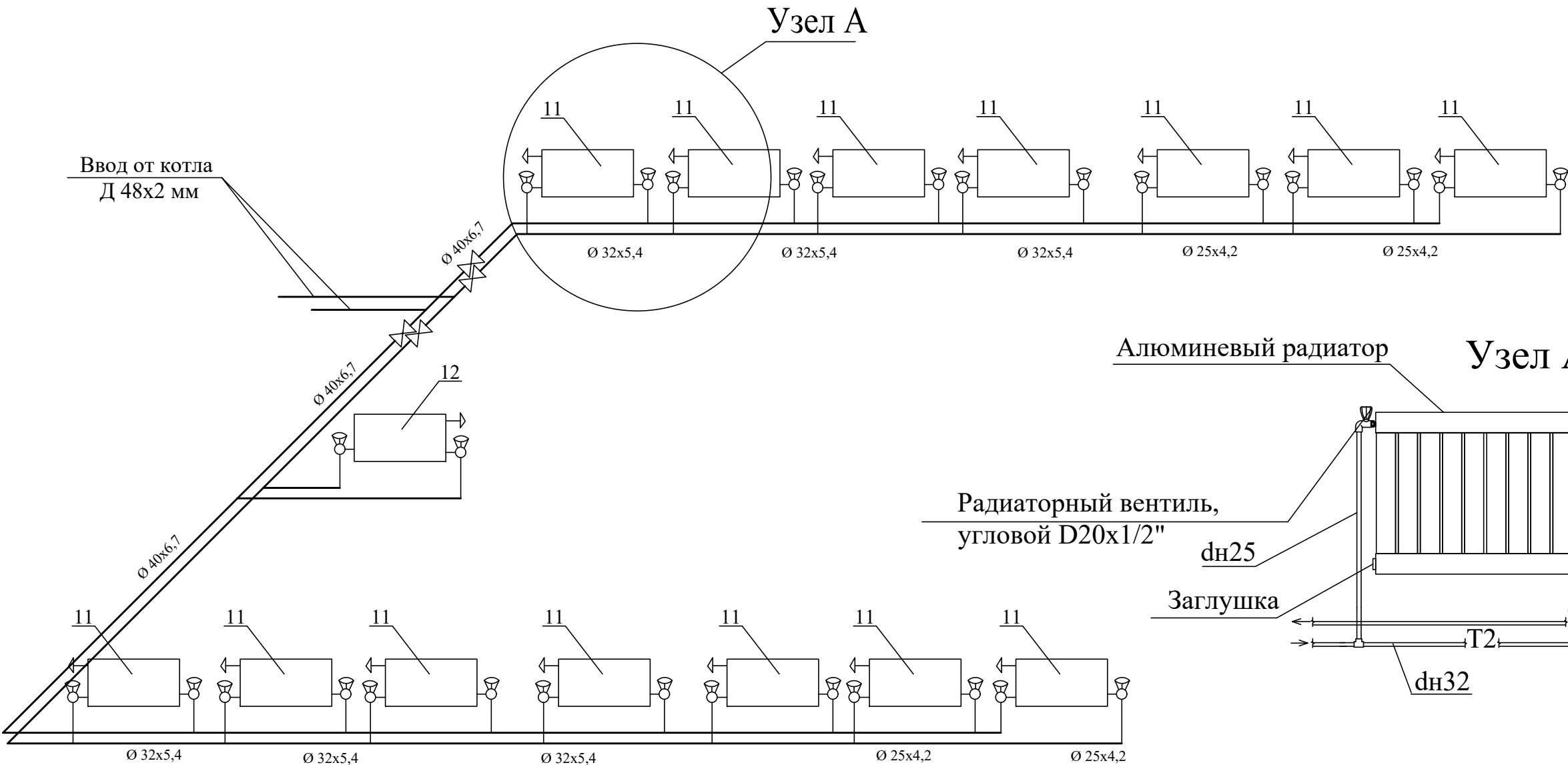
Схема прокладки труб в конструкции пола
