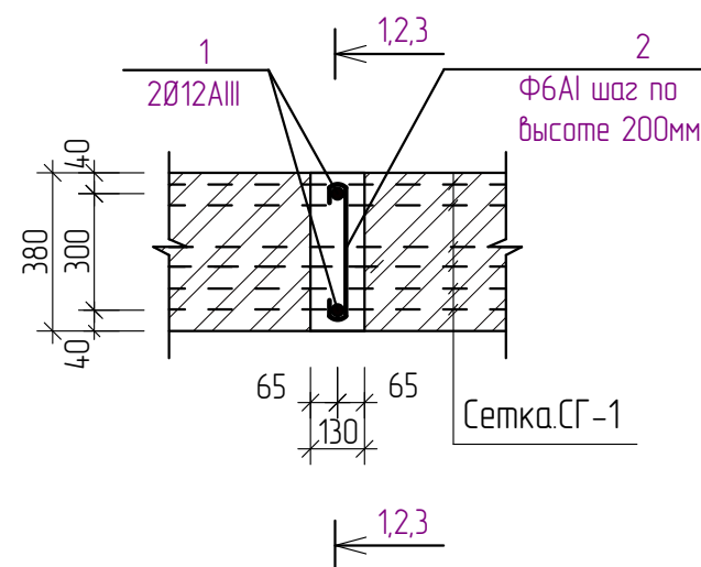
Монолитный сердечник СМ-2
