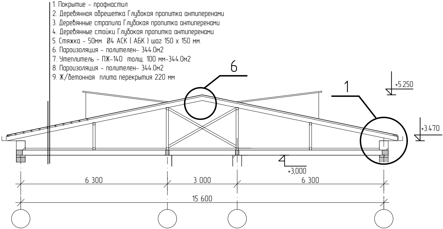
Разрез 1-1
