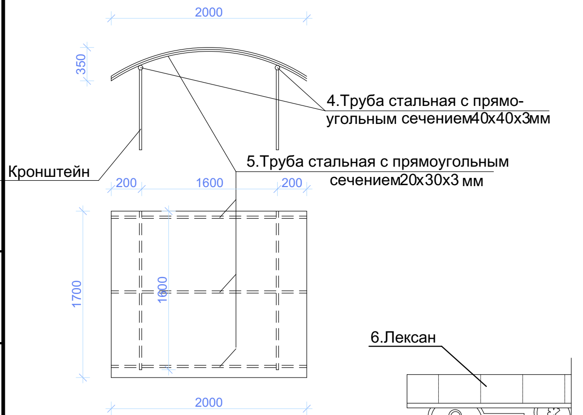
Козырек крыльца КЗ-1
