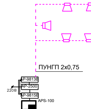
Схема оповещения о пожаре
