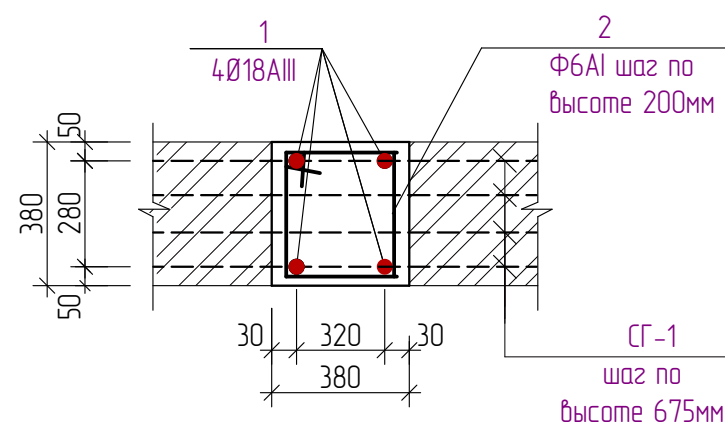
Монолитный сердечник СМ-1
