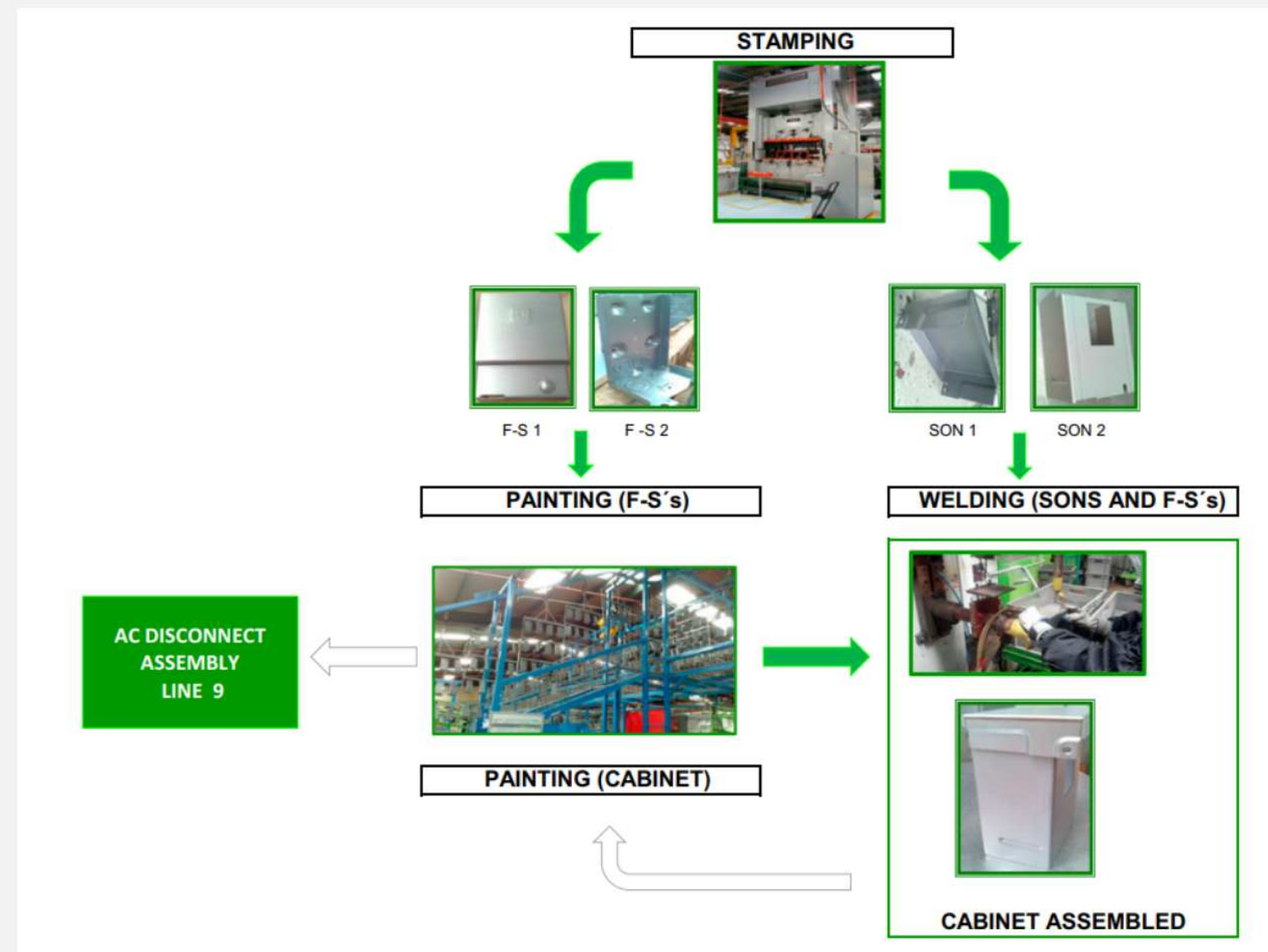
실제 공정 흐름 (캐비닛 제조)
