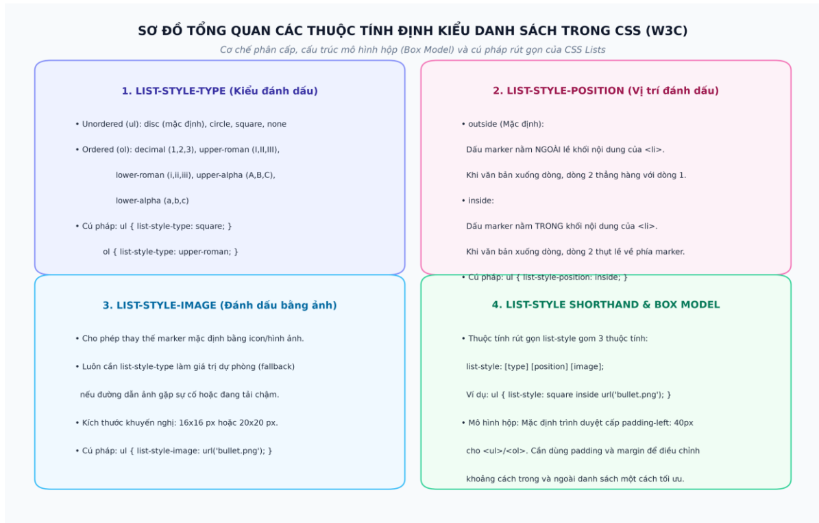
Hình 1: Sơ đồ kiến trúc và cơ chế phân cấp các thuộc tính CSS List theo chuẩn W3C
