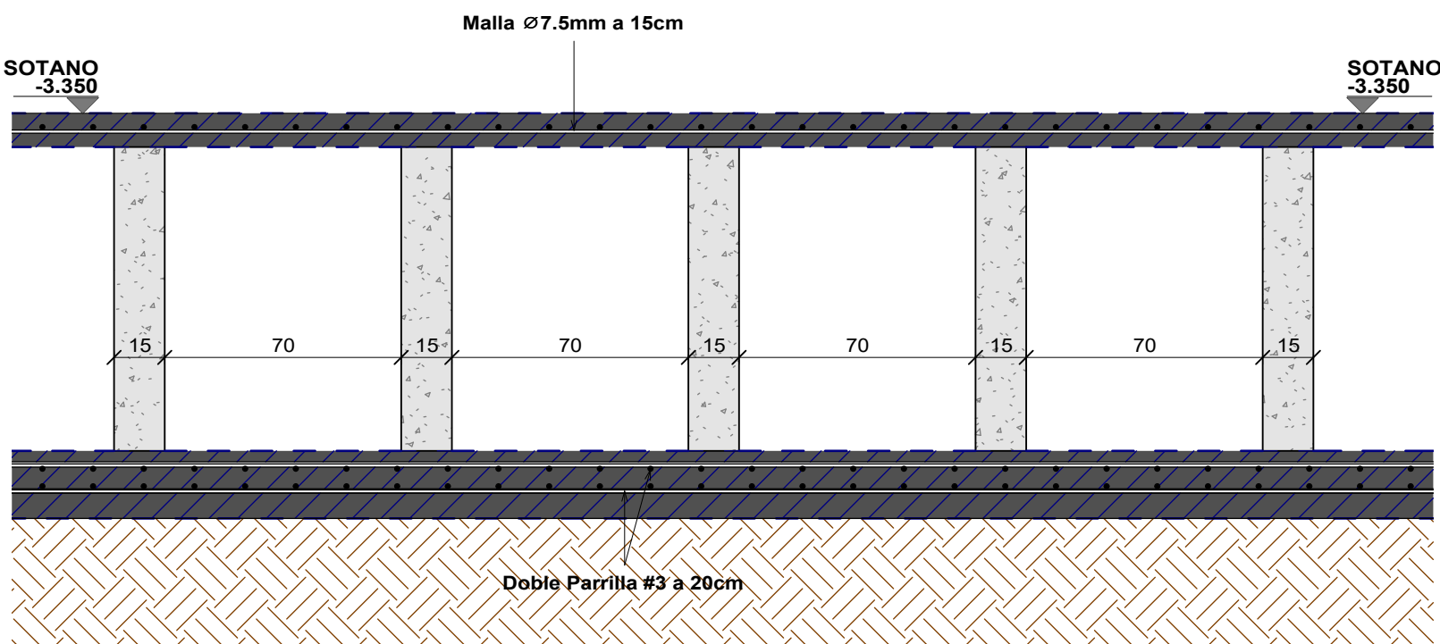
3 Sección 5 1 : 20
