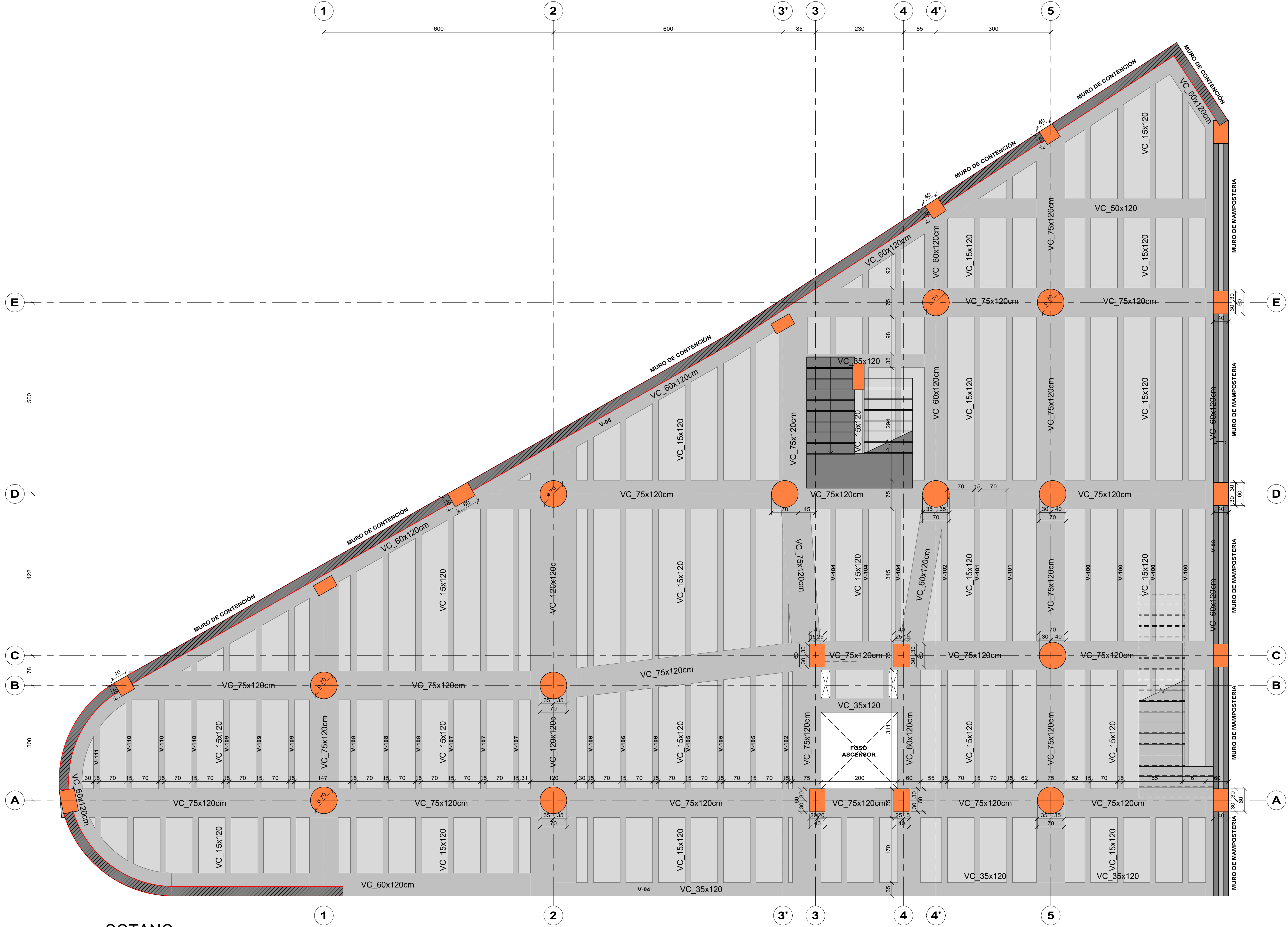
1 SOTANO 1 : 50
