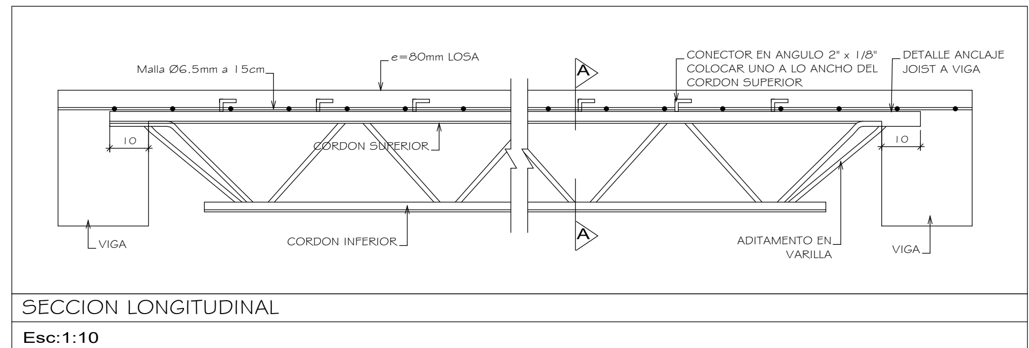
2 Detalle tipo 1 : 10
