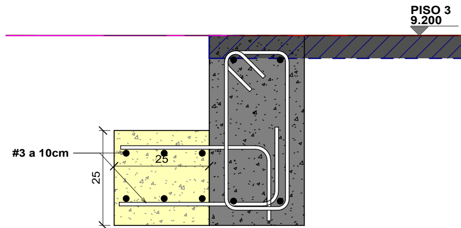
2 Detalle tipo 1 : 10
