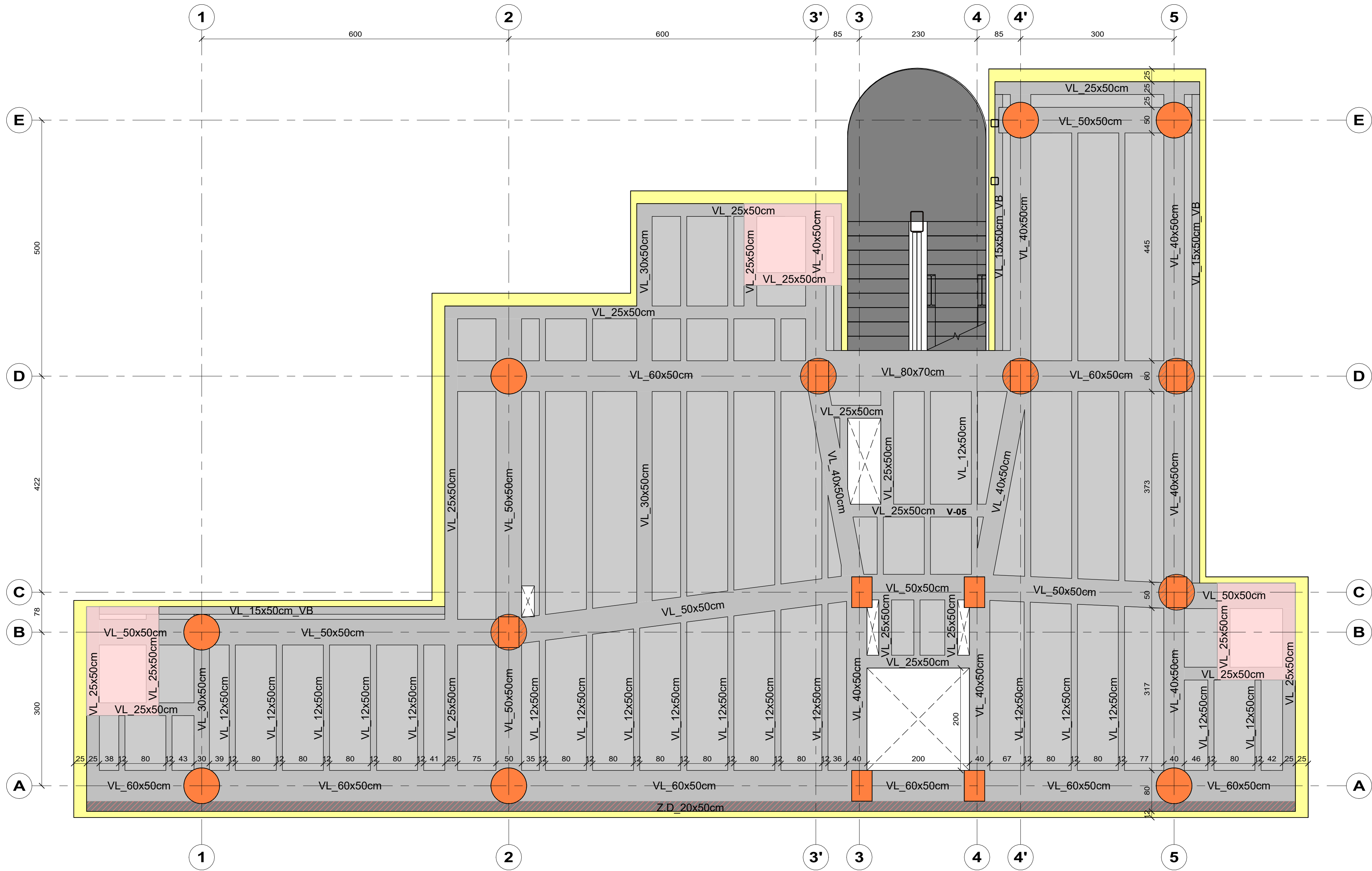
1 PISO 3 1 : 50
