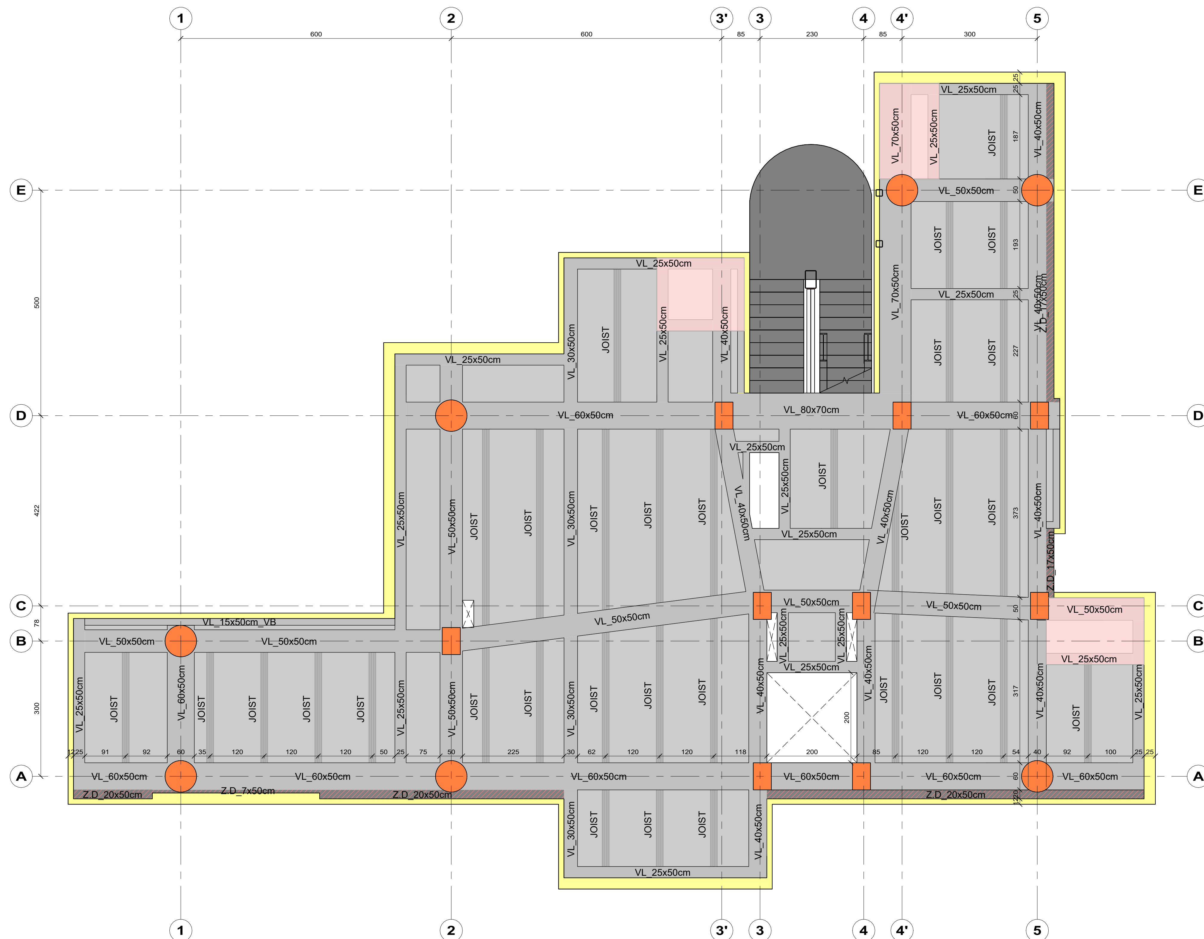
1 PISO 4 1 : 50
