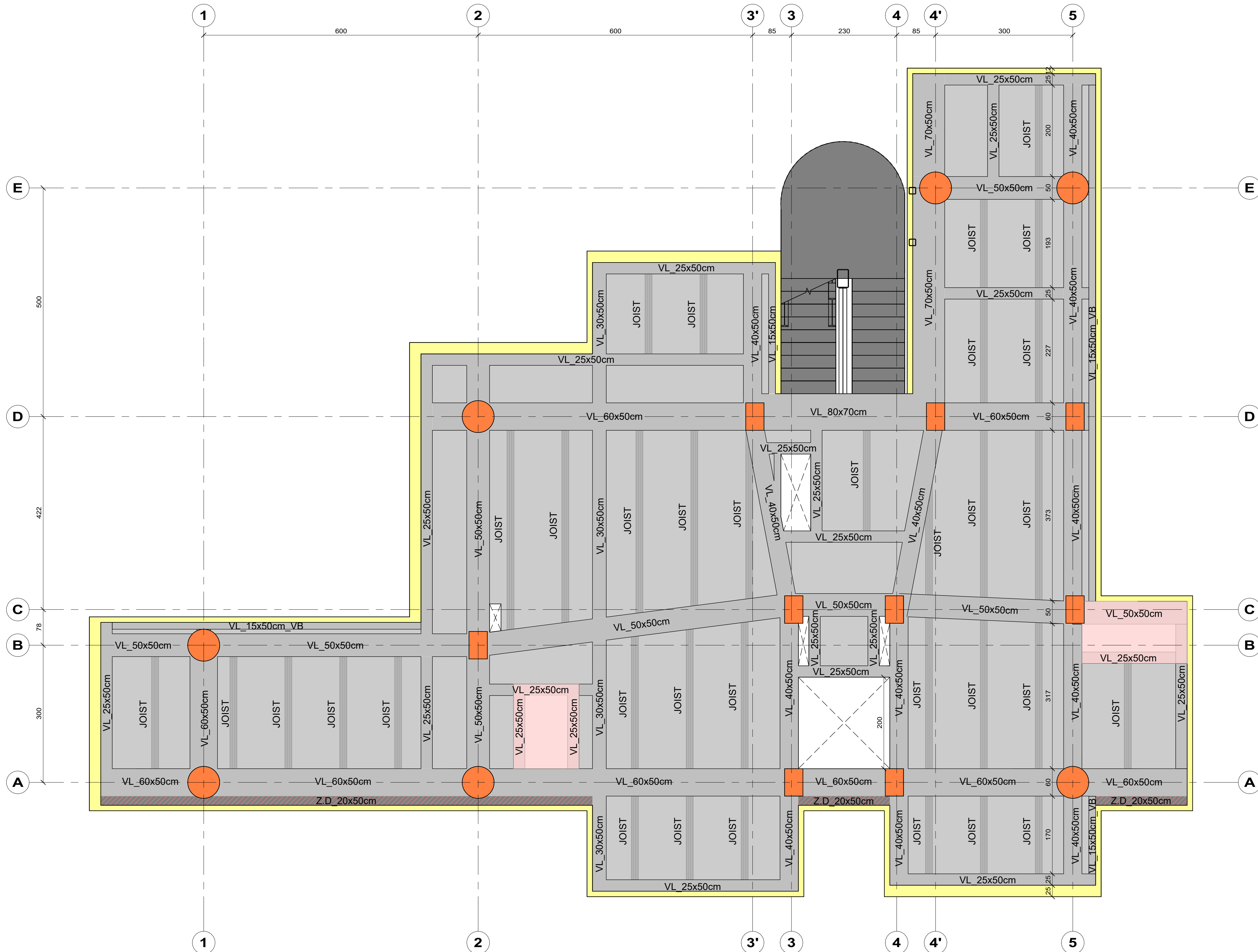
1 PISO 5 1 : 50
