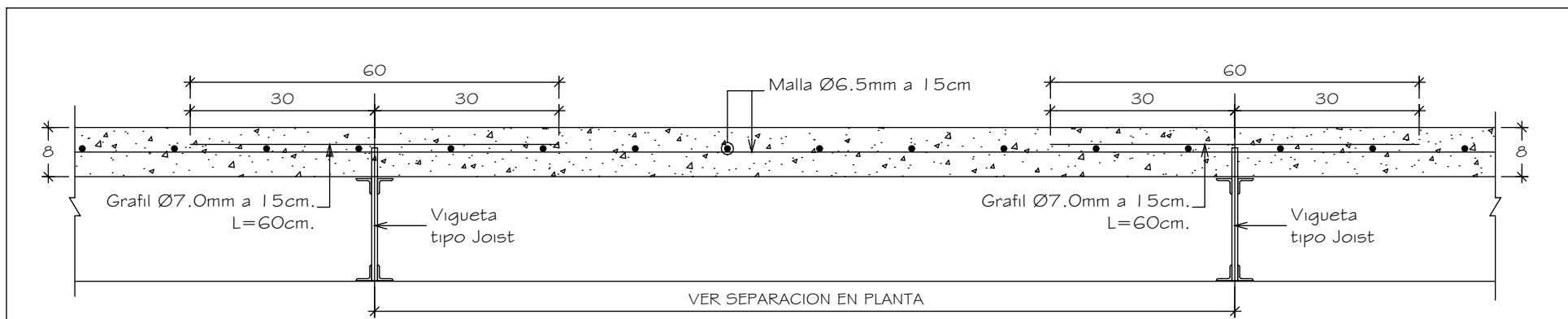
DETALLE TÍPICO DE LOSA Esc:1:10
