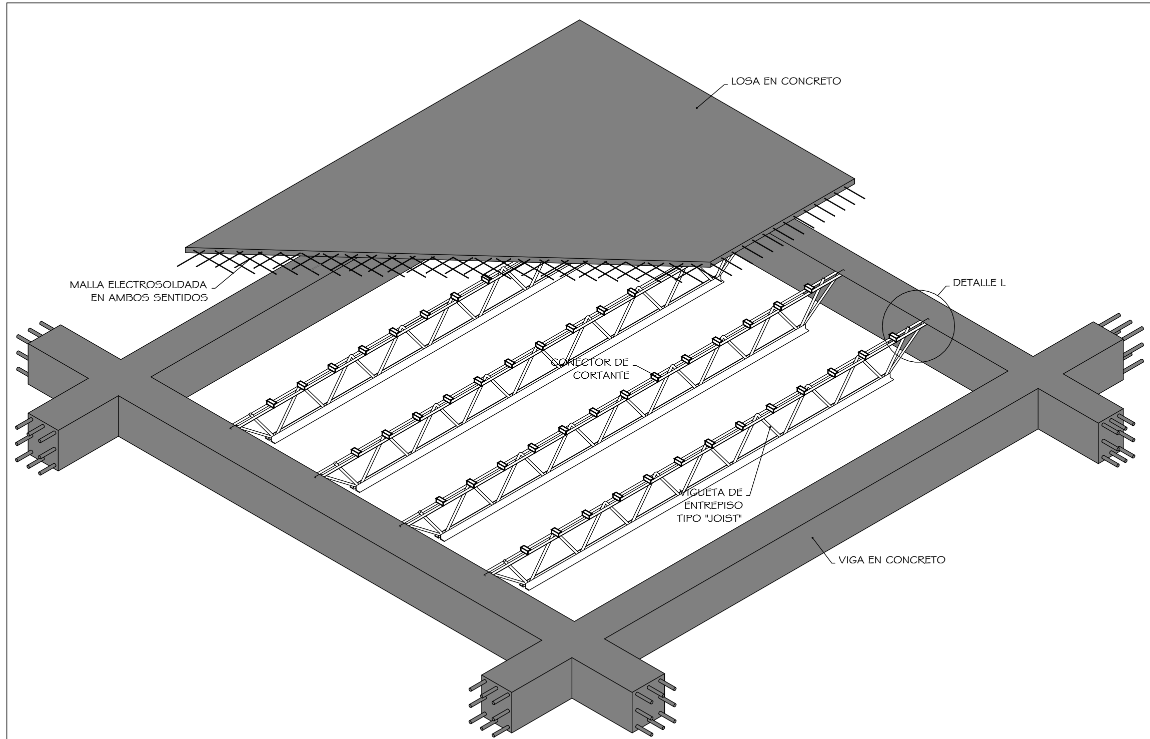
ISOMETRIA LOSA MACIZA SOPORTADA CON JOIST Esc:1:50
