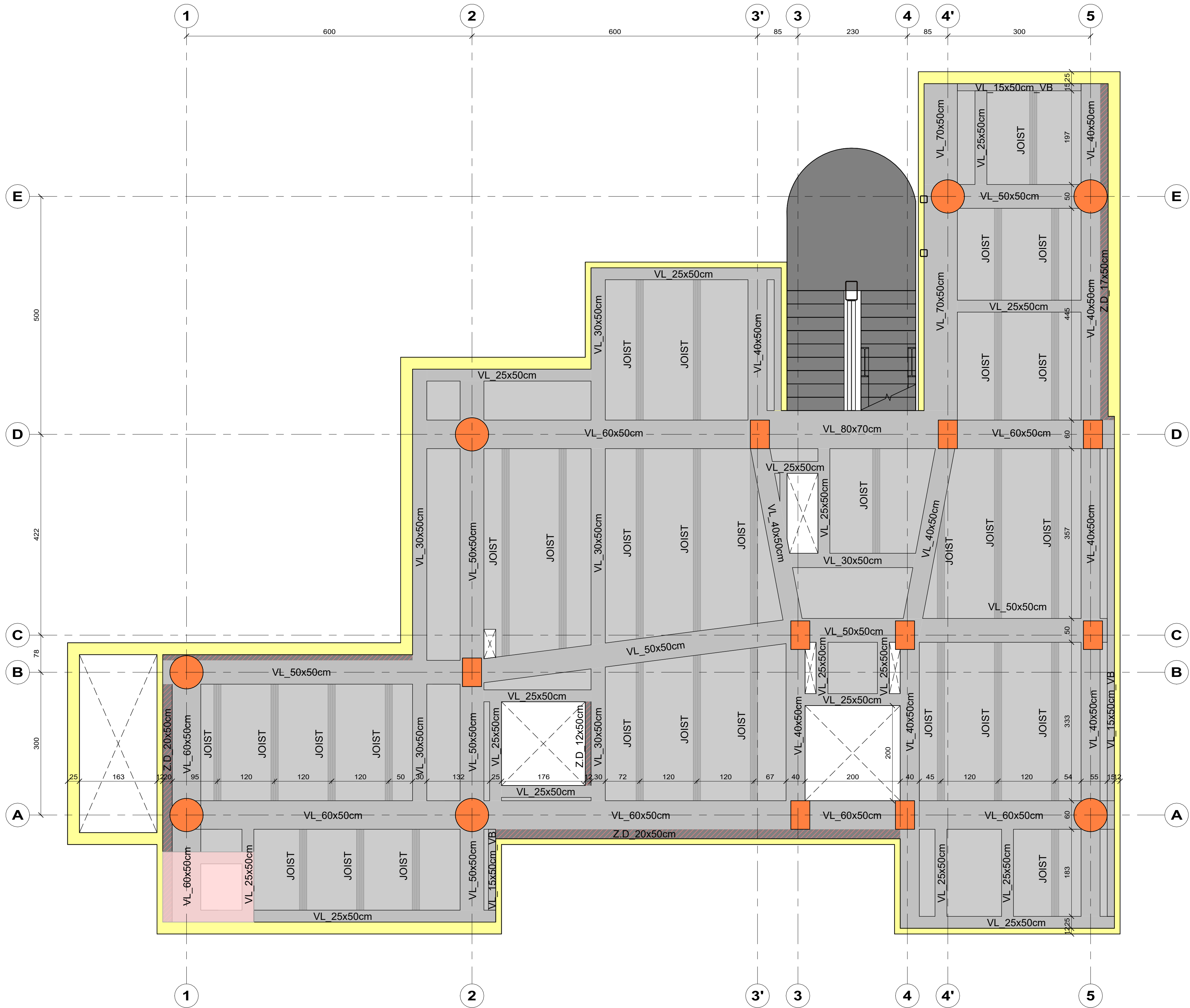
1 PISO 6 1 : 50
