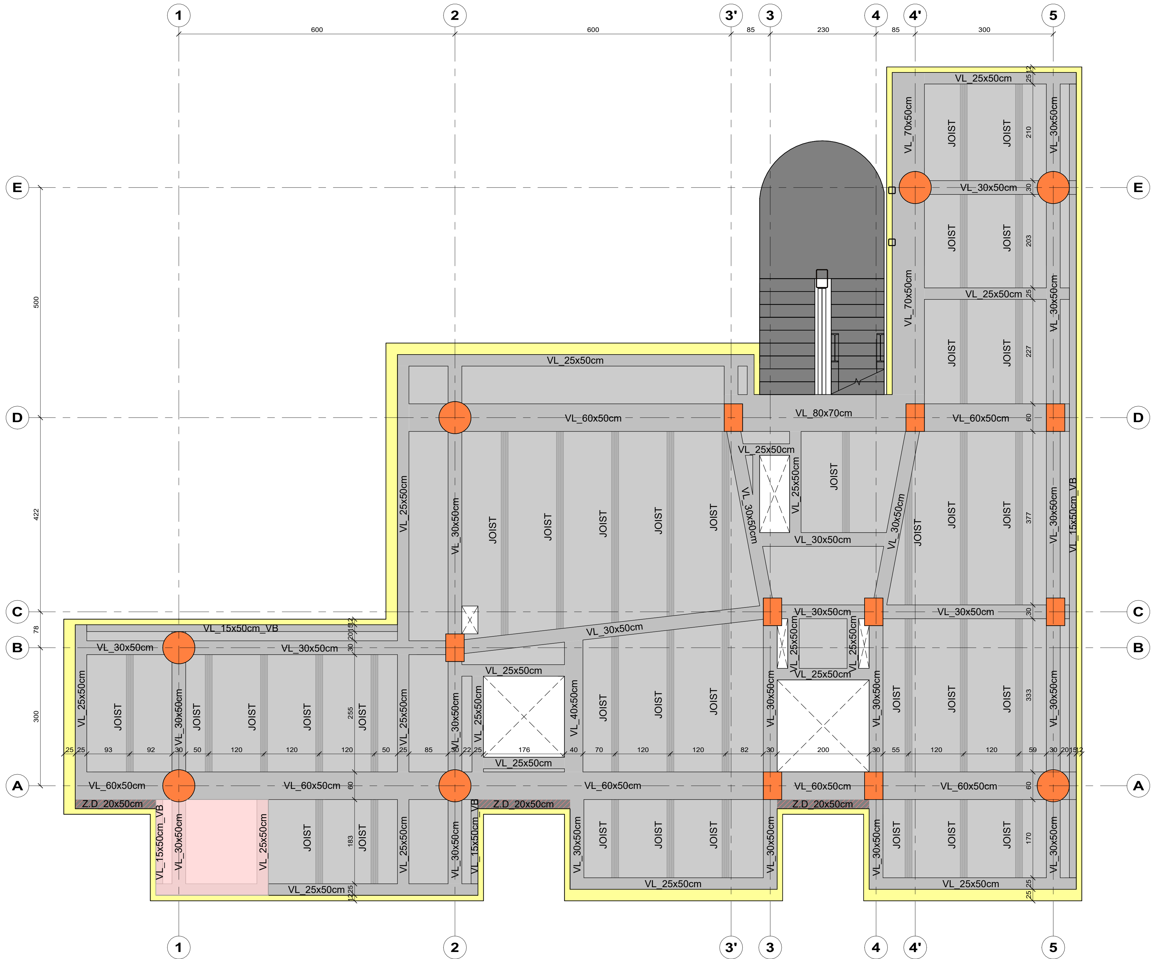
PISO 7 1 : 50
