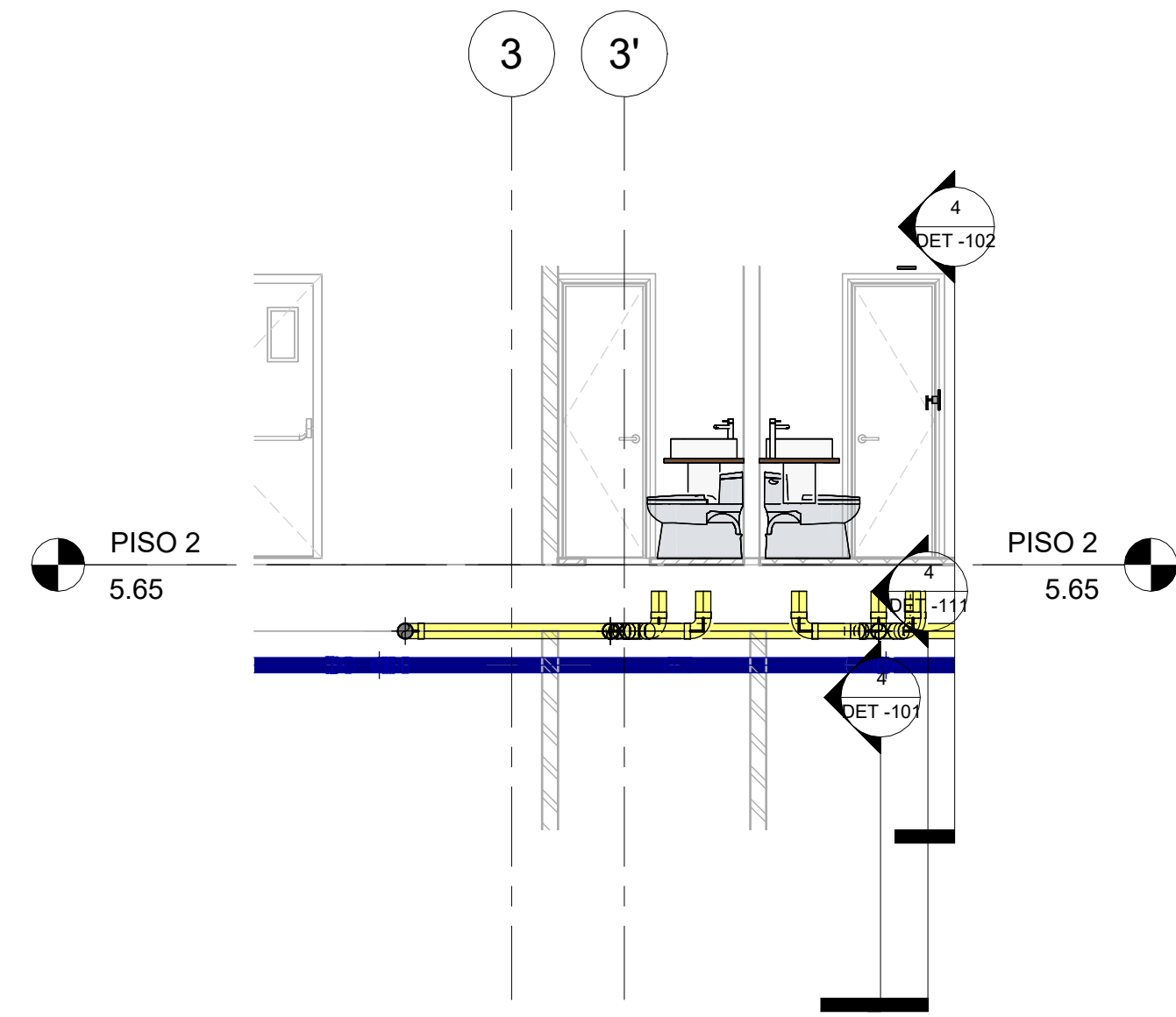
3 SEC_Long_CL_PISO 2 - SANITARIO 1 : 50
