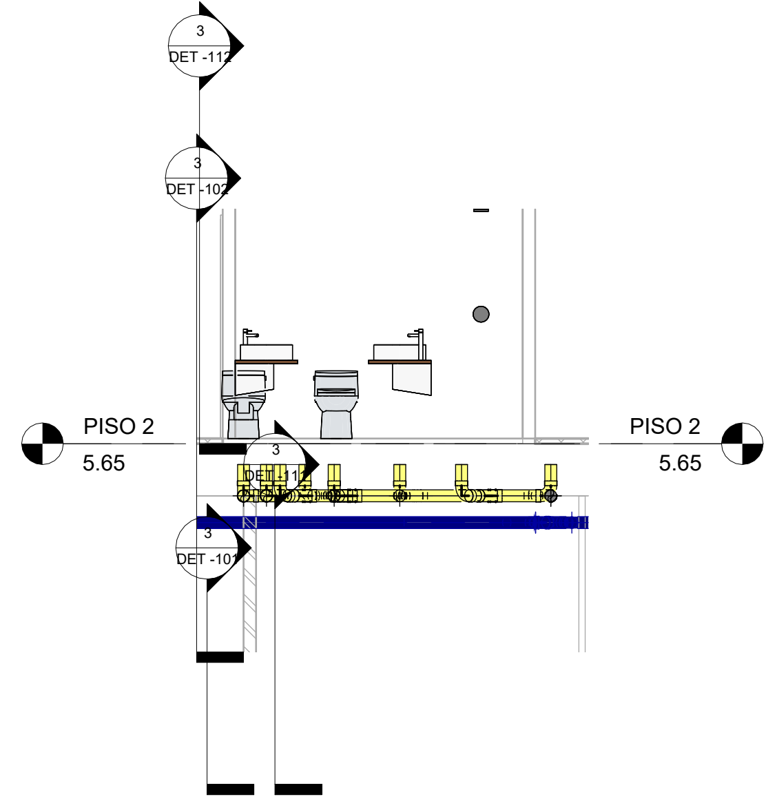
4 SEC_Trans_CL_PISO 2 - SANITARIO 1 : 50
