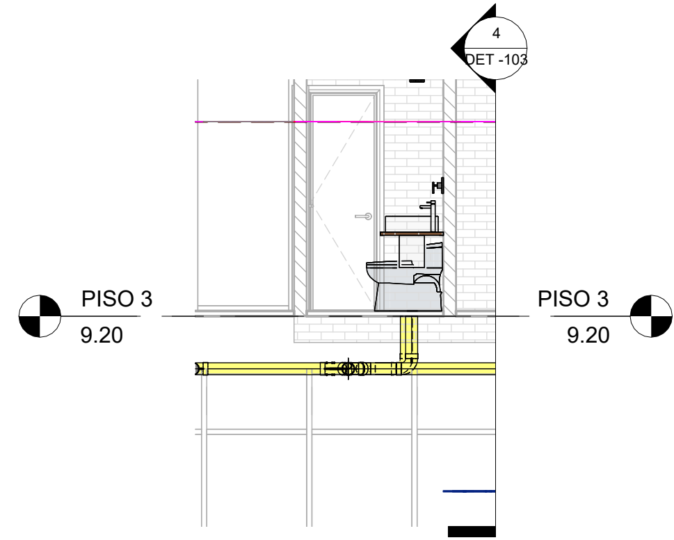
3 SEC_Long_CL_PISO 3 - SANITARIO 1 : 50
