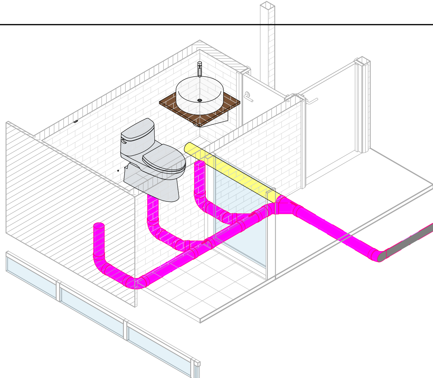
2 3D_CL_PISO 3 - SANITARIO
