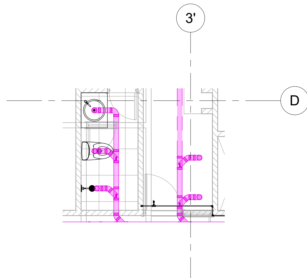
5 CL_PISO 3 - SANITARIO_2 1 : 50
