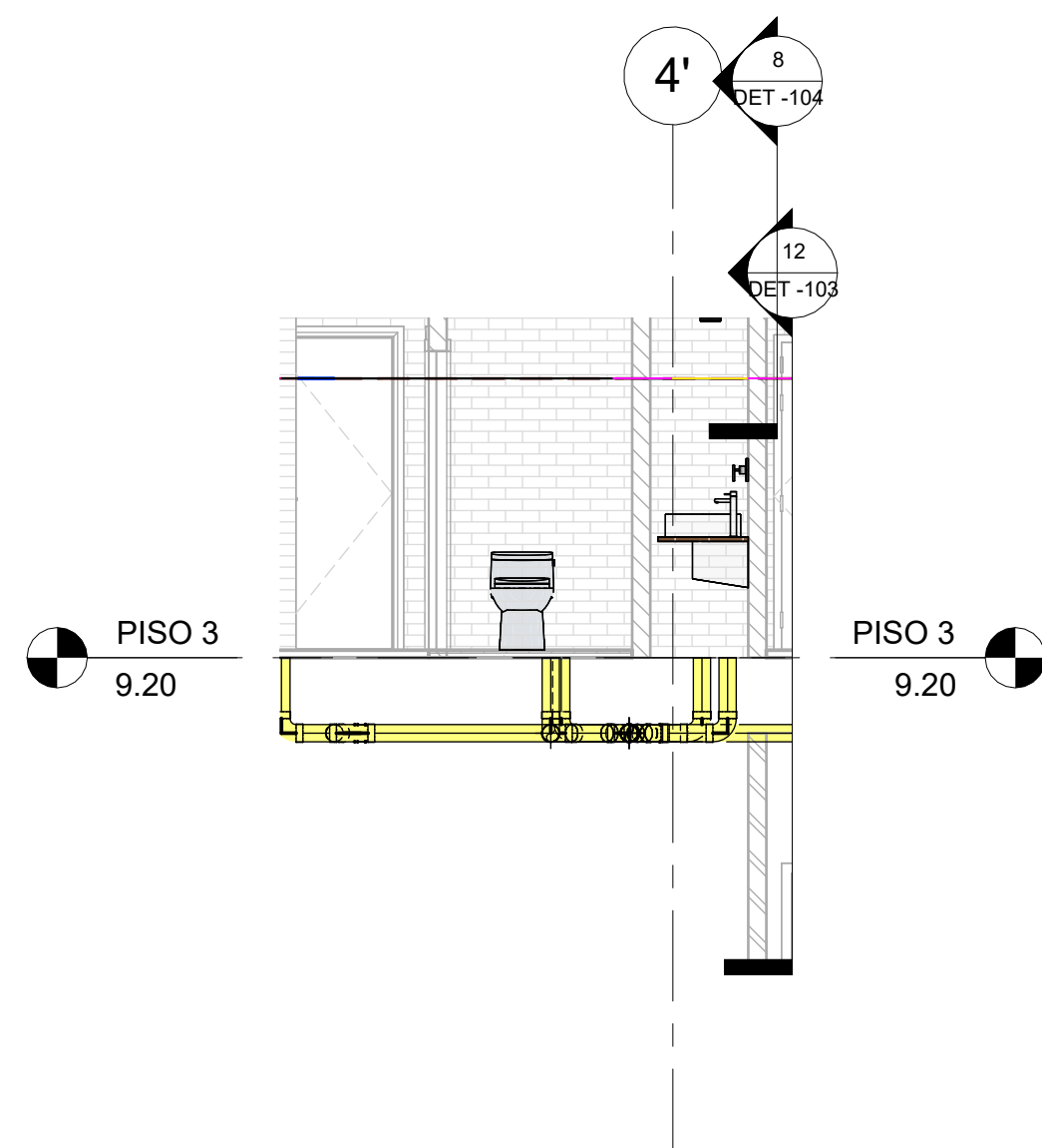
11 SEC_Long_CL_PISO 3 - SANITARIO_3 1 : 50
