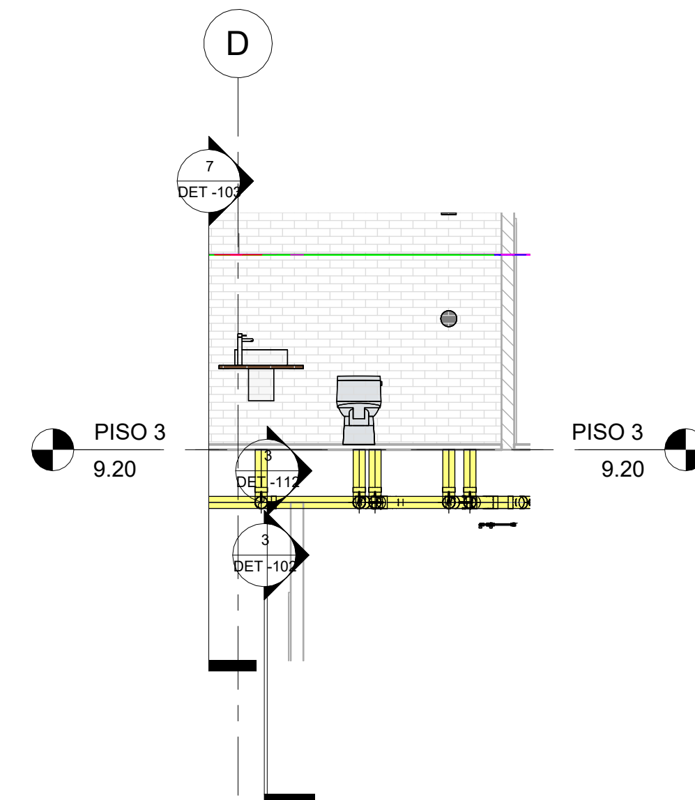
8 SEC_Trans_CL_PISO 3 - SANITARIO_2 1 : 50
