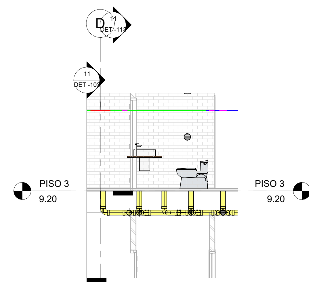
12 SEC_Trans_CL_PISO 3 - SANITARIO_3 1 : 50
