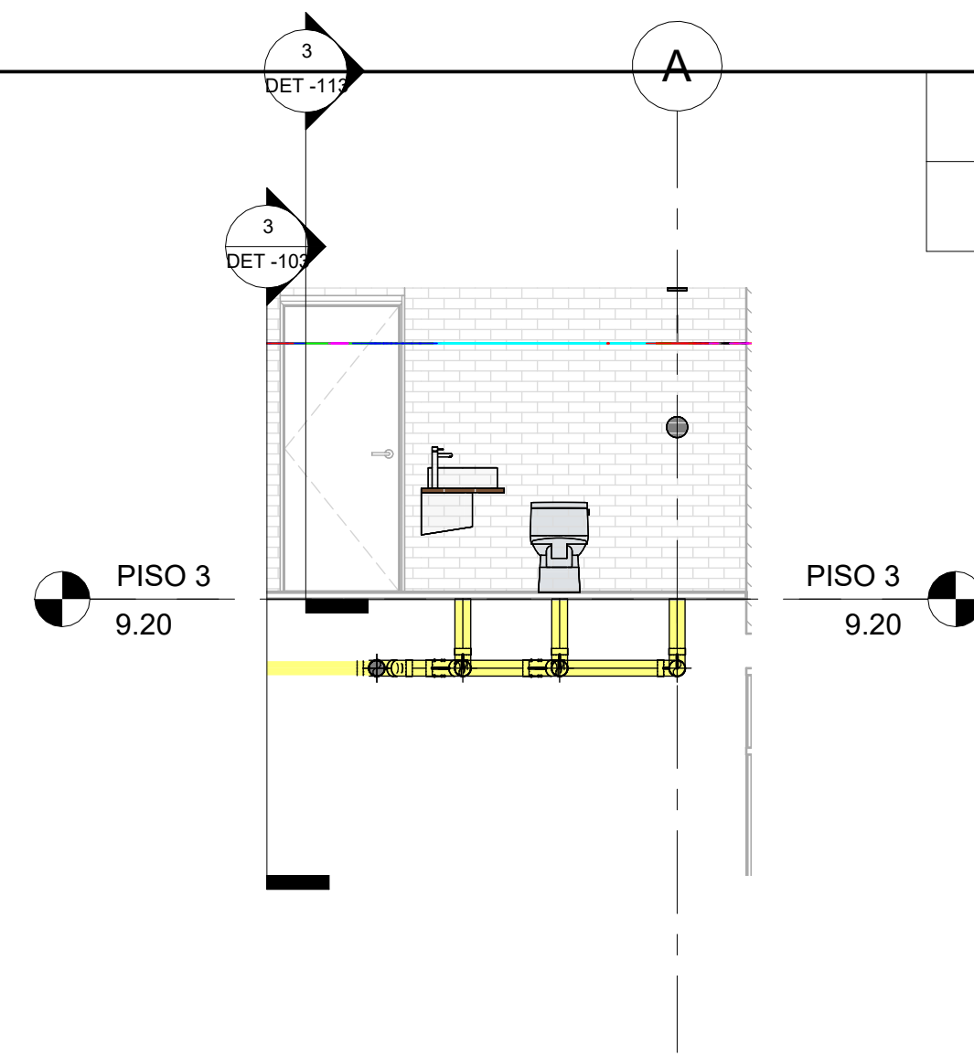
4 SEC_Trans_CL_PISO 3 - SANITARIO 1 : 50
