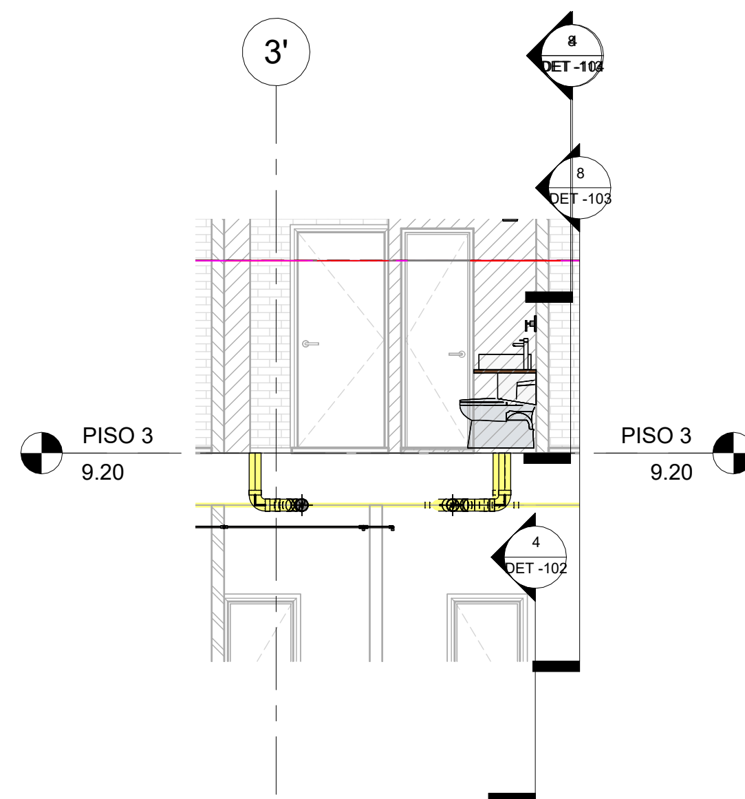
7 SEC_Long_CL_PISO 3 - SANITARIO_2 1 : 50
