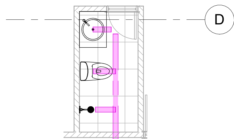
1 CL_PISO 4 - SANITARIO 1 : 50
