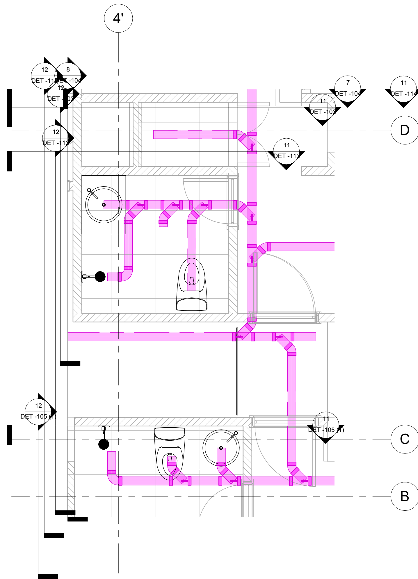
5 CL_PISO 4 - SANITARIO_2 1 : 30
