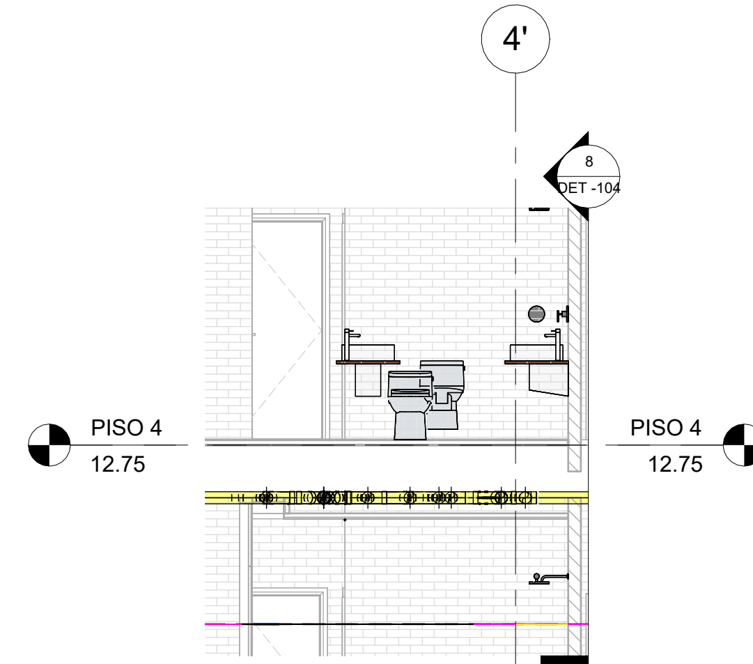
8 SEC_Trans_CL_PISO 4 - SANITARIO_2 1 : 50
