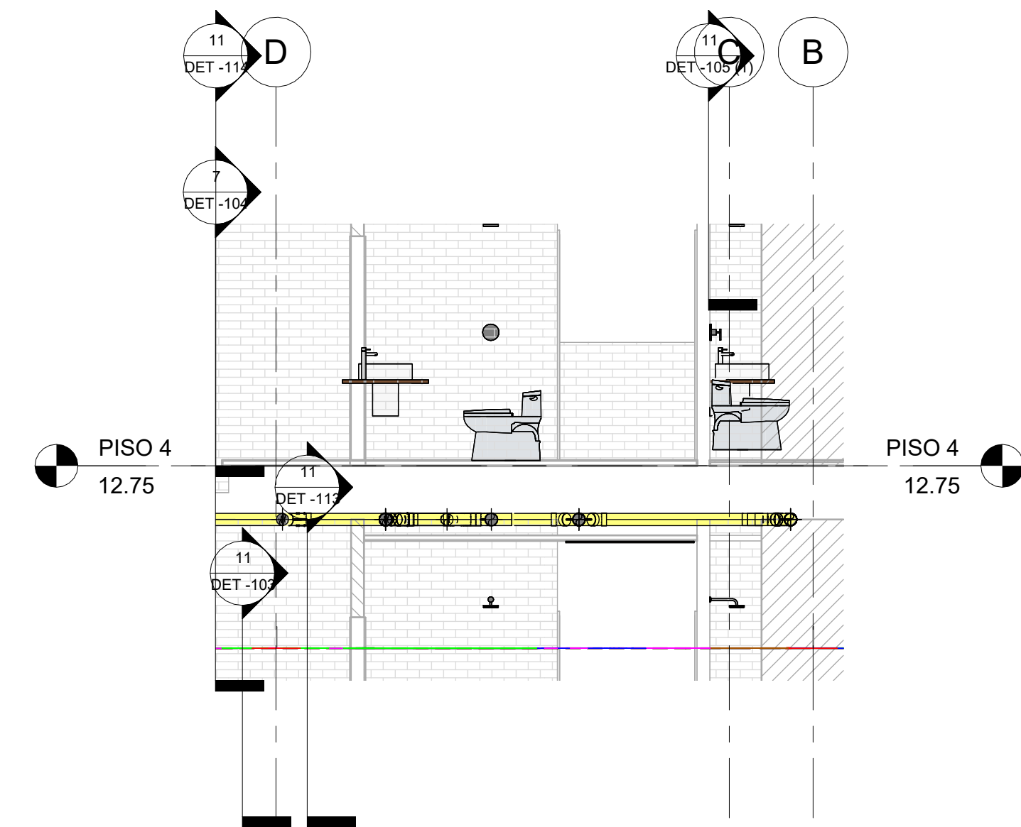
8 SEC_Trans_CL_PISO 4 - SANITARIO_2 1 : 50
