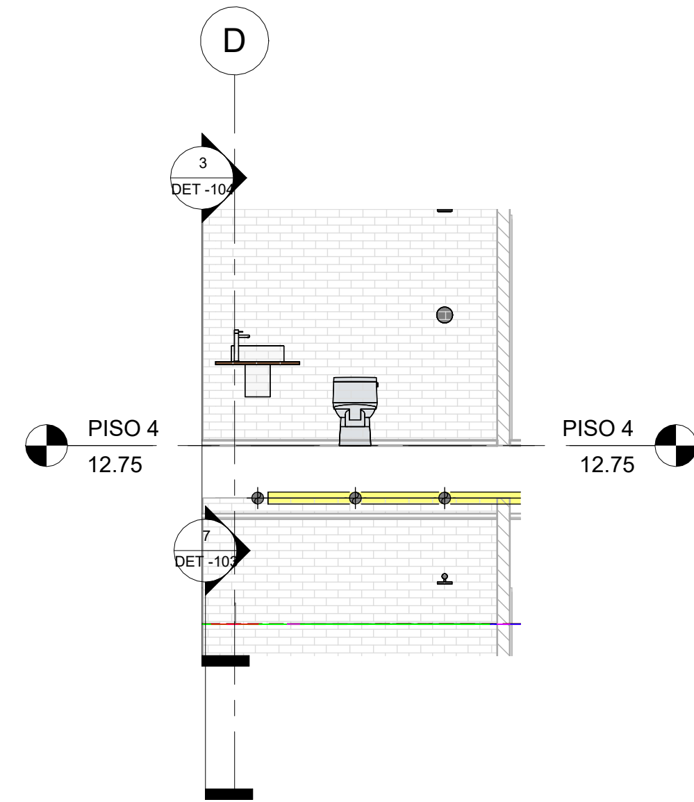
4 SEC_Trans_CL_PISO 4 - SANITARIO 1 : 50
