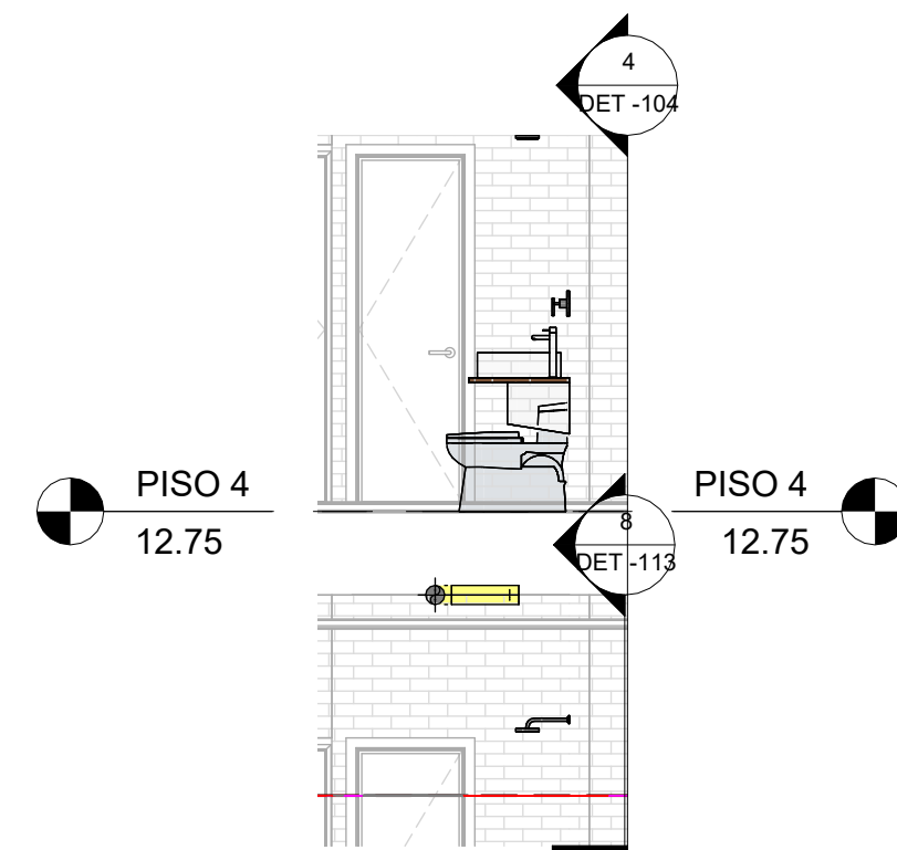
3 SEC_Long_CL_PISO 4 - SANITARIO 1 : 50
