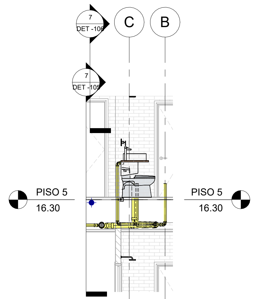
8 SEC_Trans_CL_PISO 5 - SANITARIO_2 1 : 50
