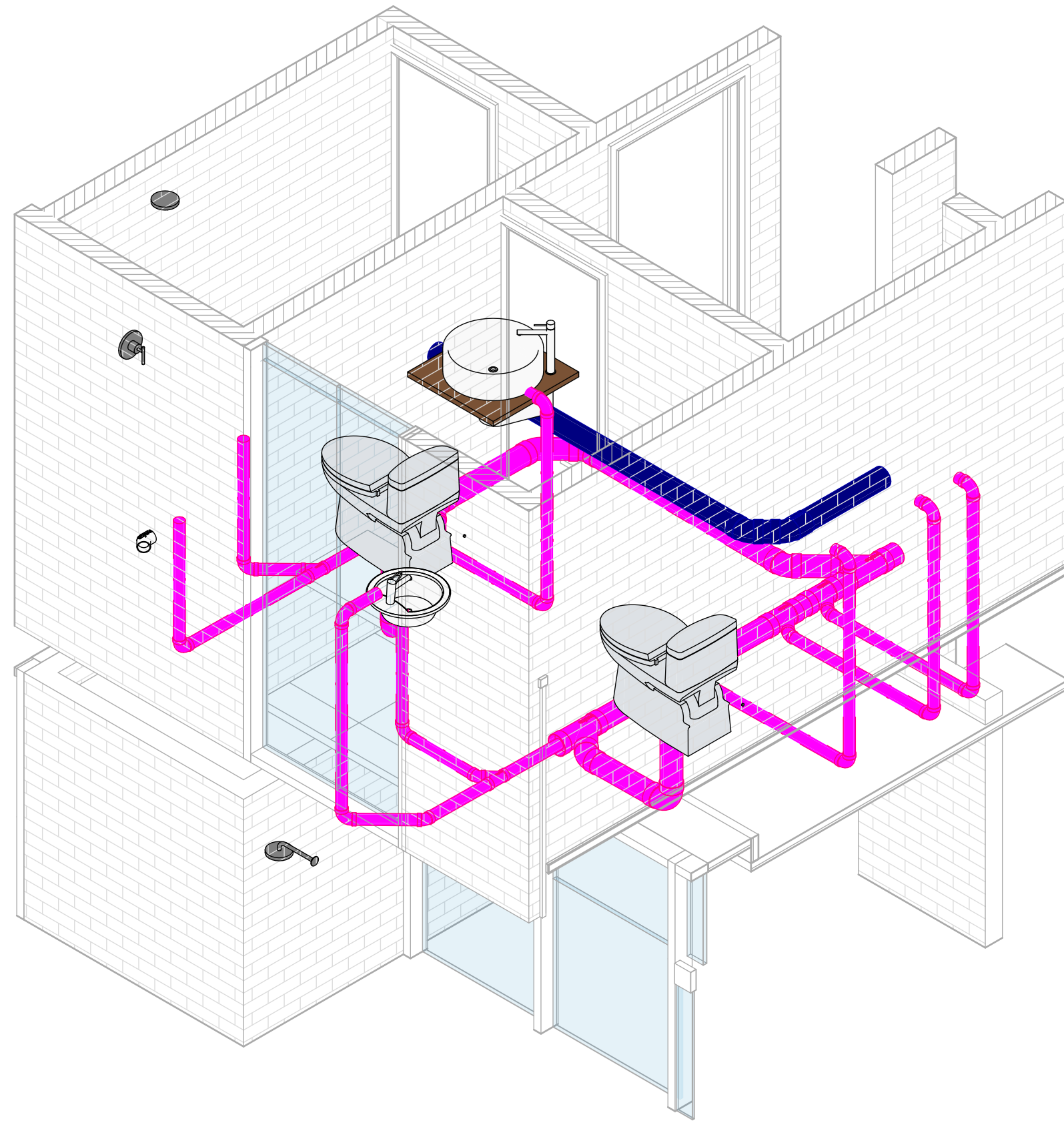
2 3D_CL_PISO 5 - SANITARIO
