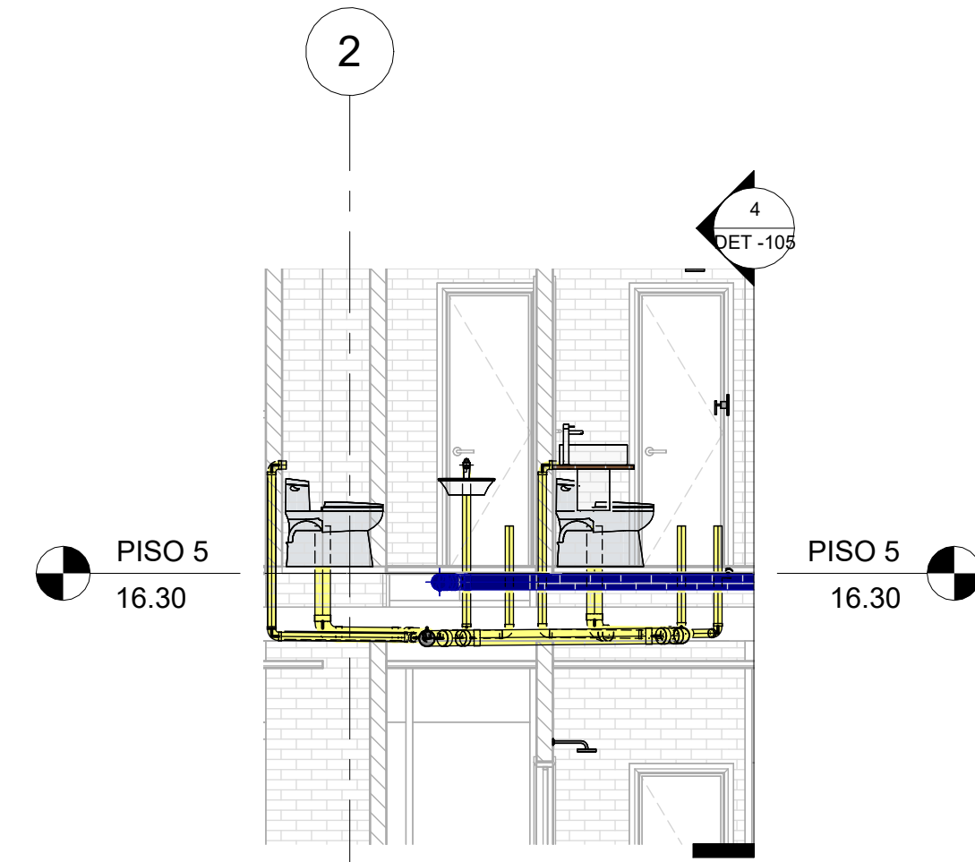
3 SEC_Long_CL_PISO 5 - SANITARIO 1 : 50
