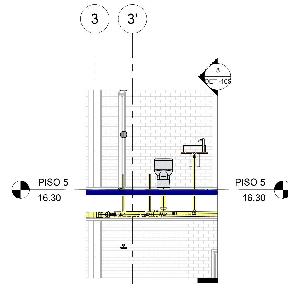
7 SEC_Long_CL_PISO 5 - SANITARIO_2 1 : 50
