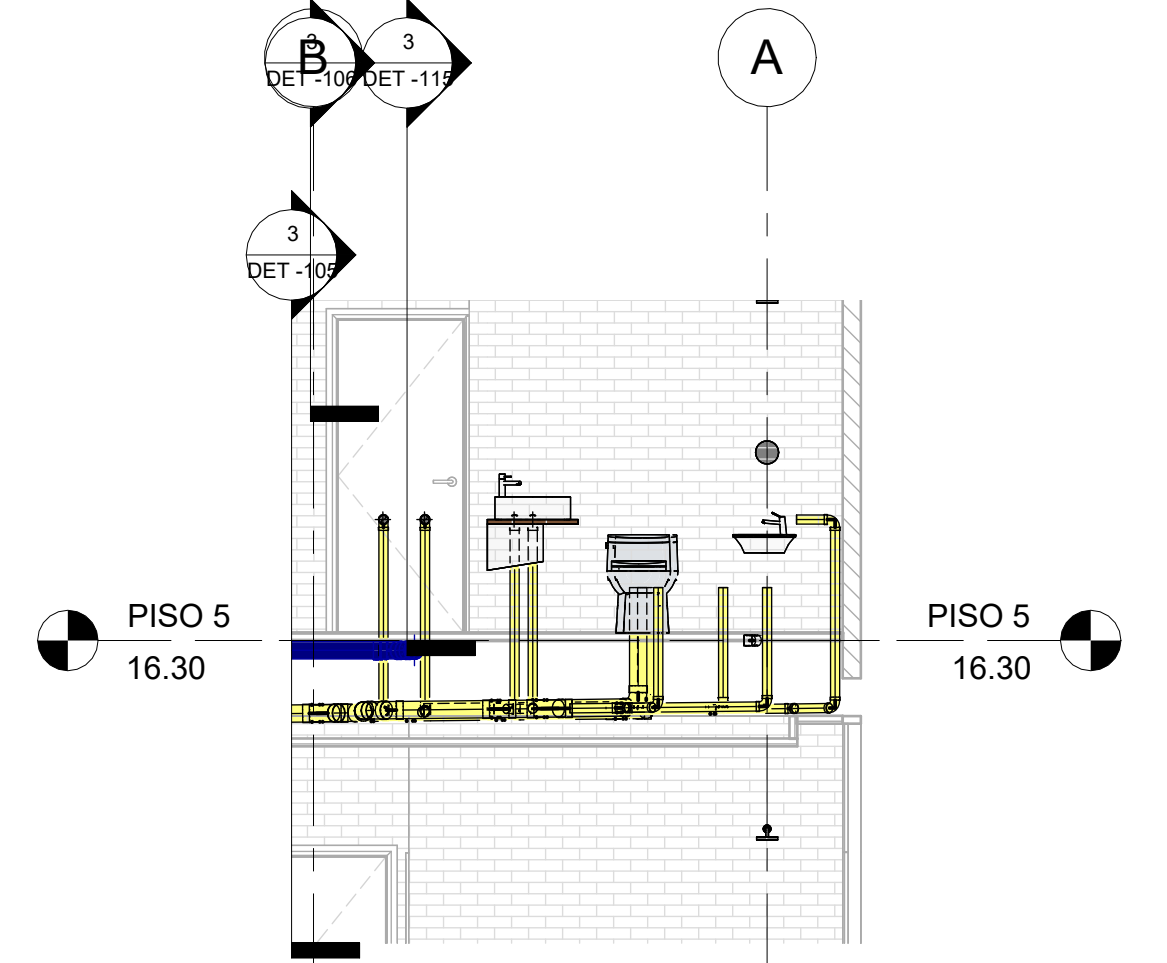
4 SEC_Trans_CL_PISO 5 - SANITARIO 1 : 50
