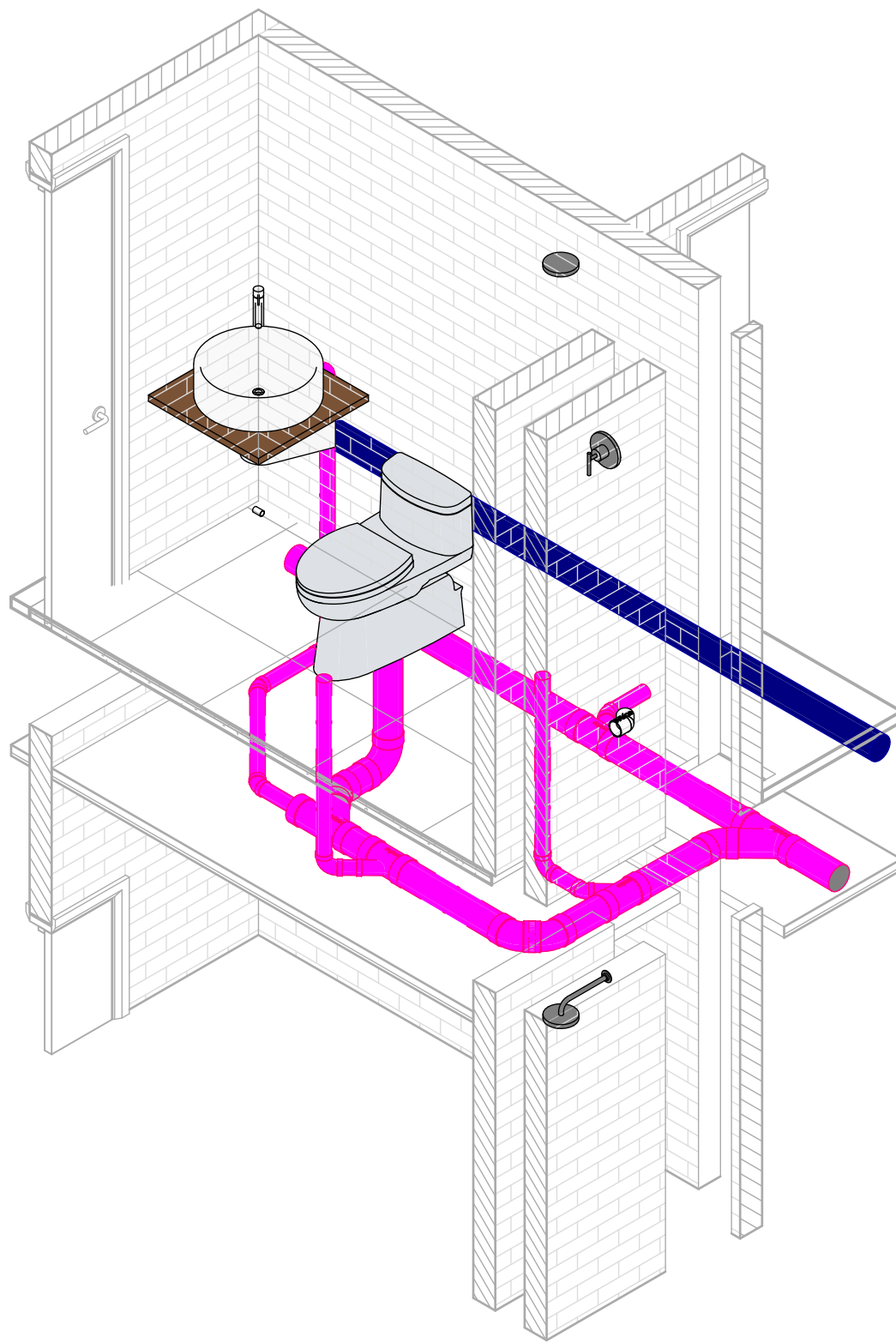
6 3D_CL_PISO 5 - SANITARIO_2
