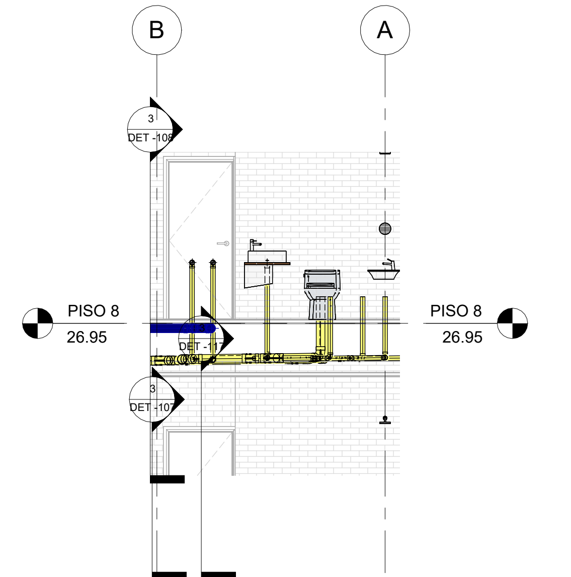
4 SEC_Trans_CL_PISO 8 - SANITARIO 1:50
