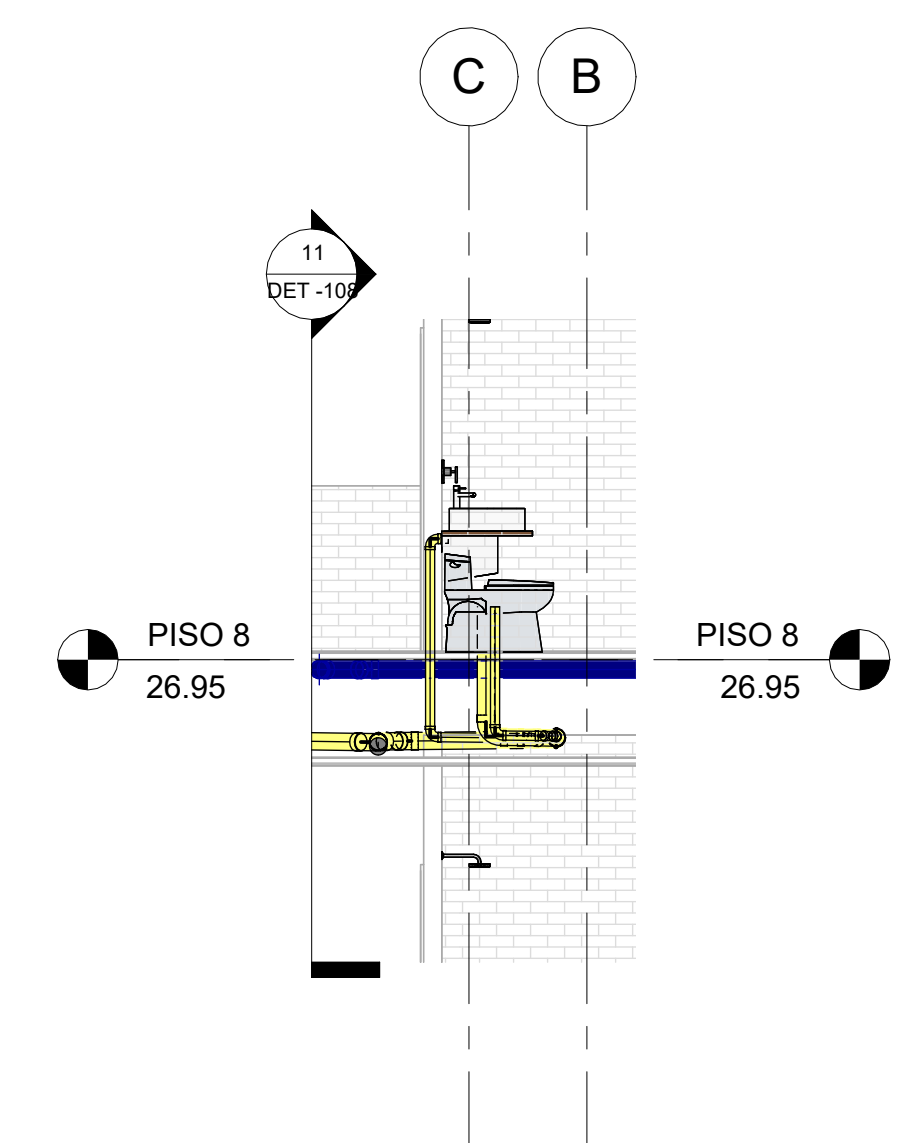
12 SEC_Trans_CL_PISO 8 - SANITARIO_3 Presupuesto No. Designación 1:50
