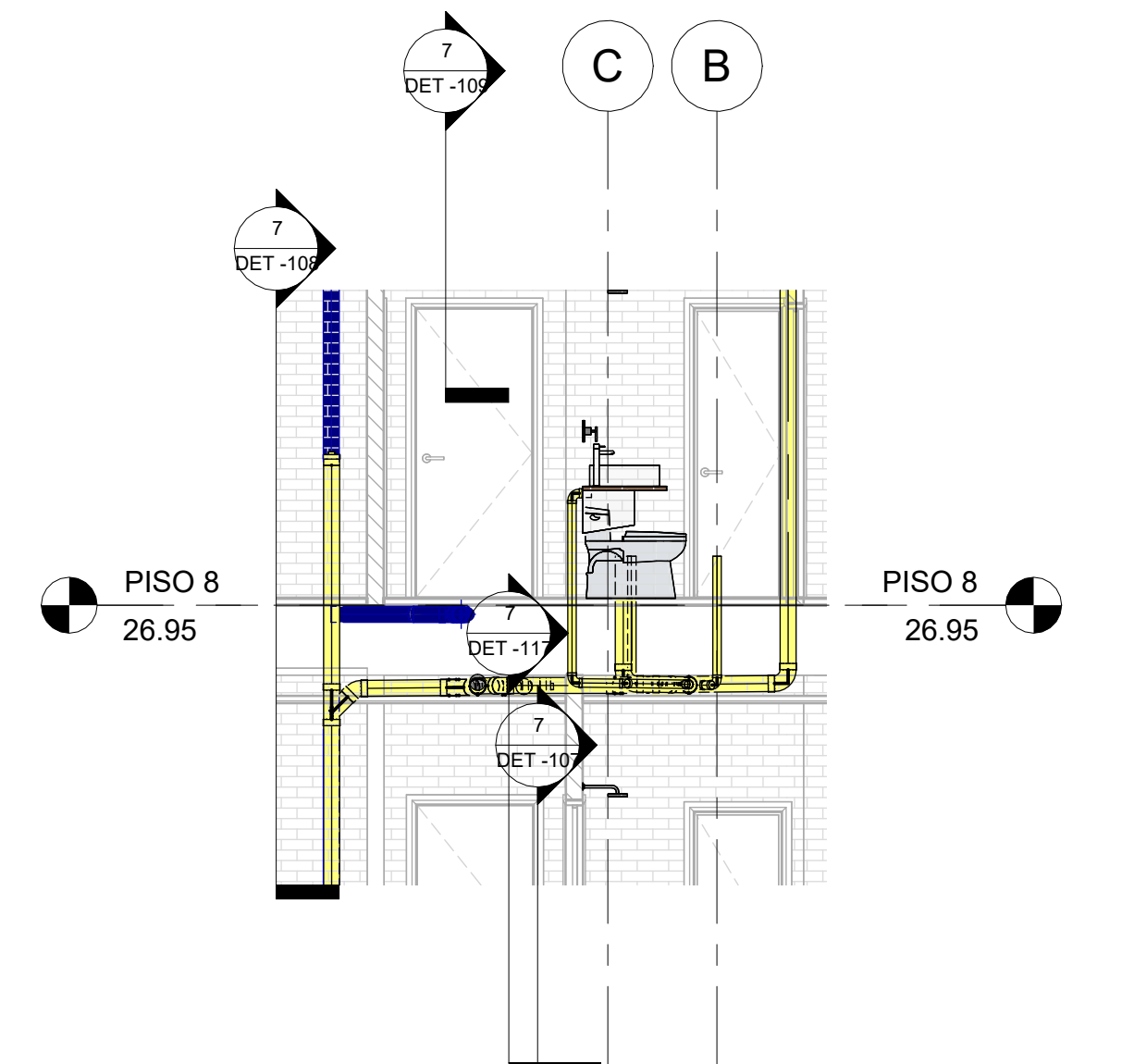
4 SEC_Trans_CL_PISO 8 - SANITARIO 1:50
