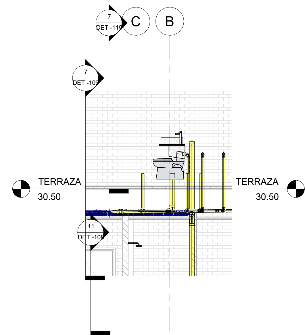
8 SEC_Trans_CL_TERRAZA - SANITARIO_2 1 : 50
