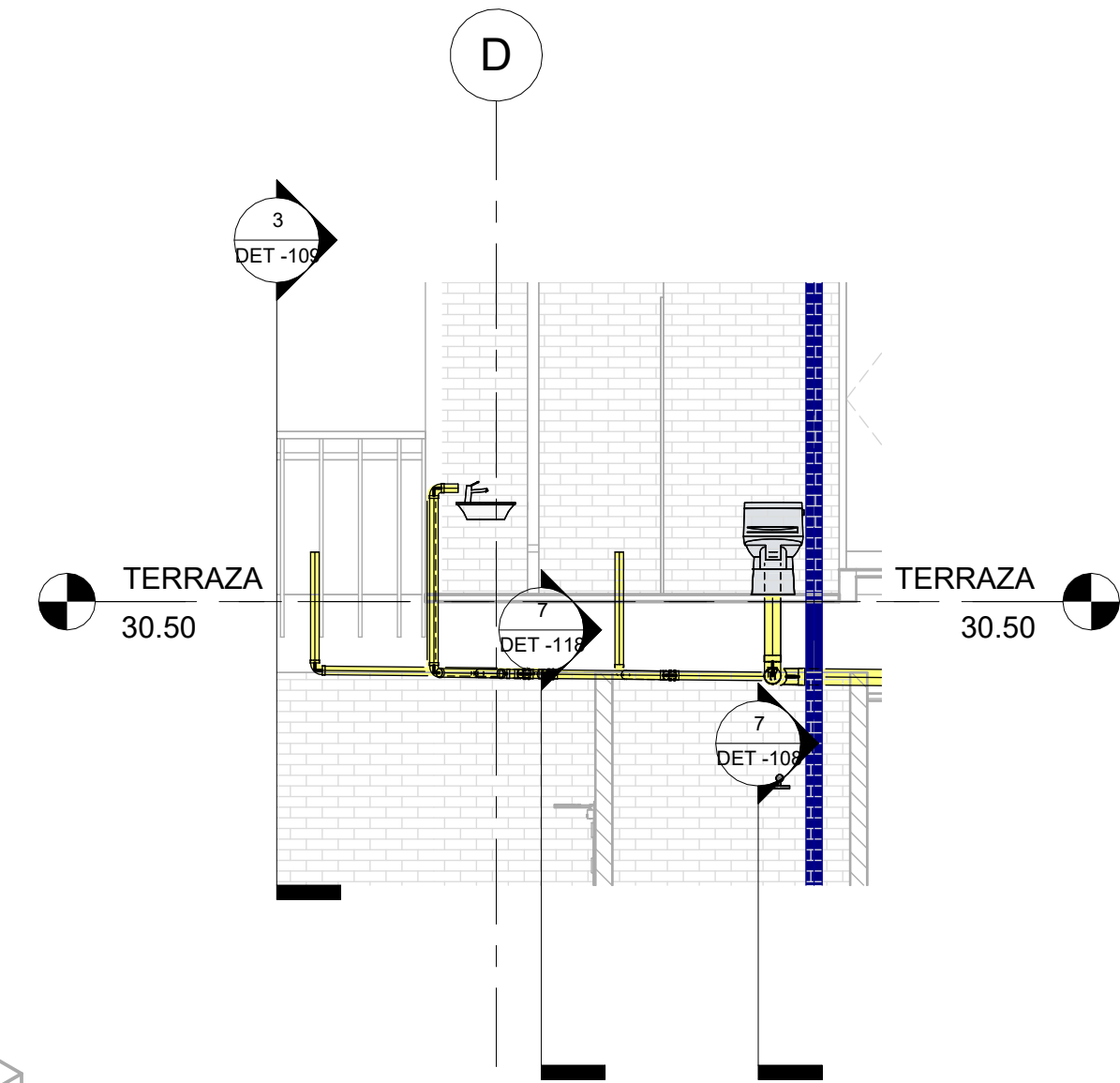
4 SEC_Trans_CL_TERRAZA - SANITARIO 1 : 50
