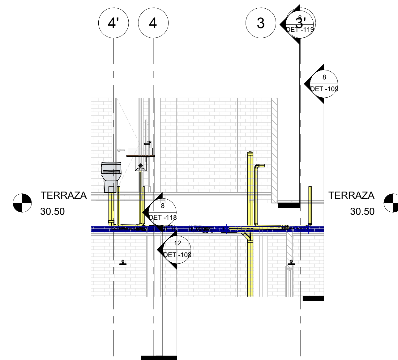
7 SEC_Long_CL_TERRAZA - SANITARIO_2 1 : 50
