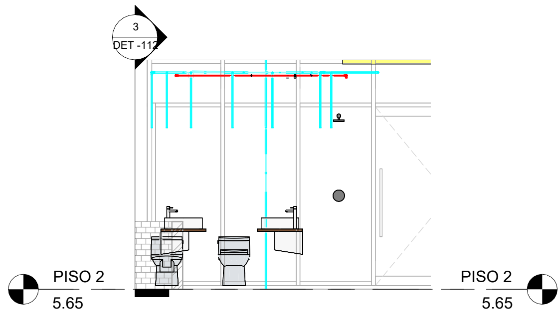
4 SEC_Trans_CL_PISO 2 - HIDRAULICO 1 : 50
