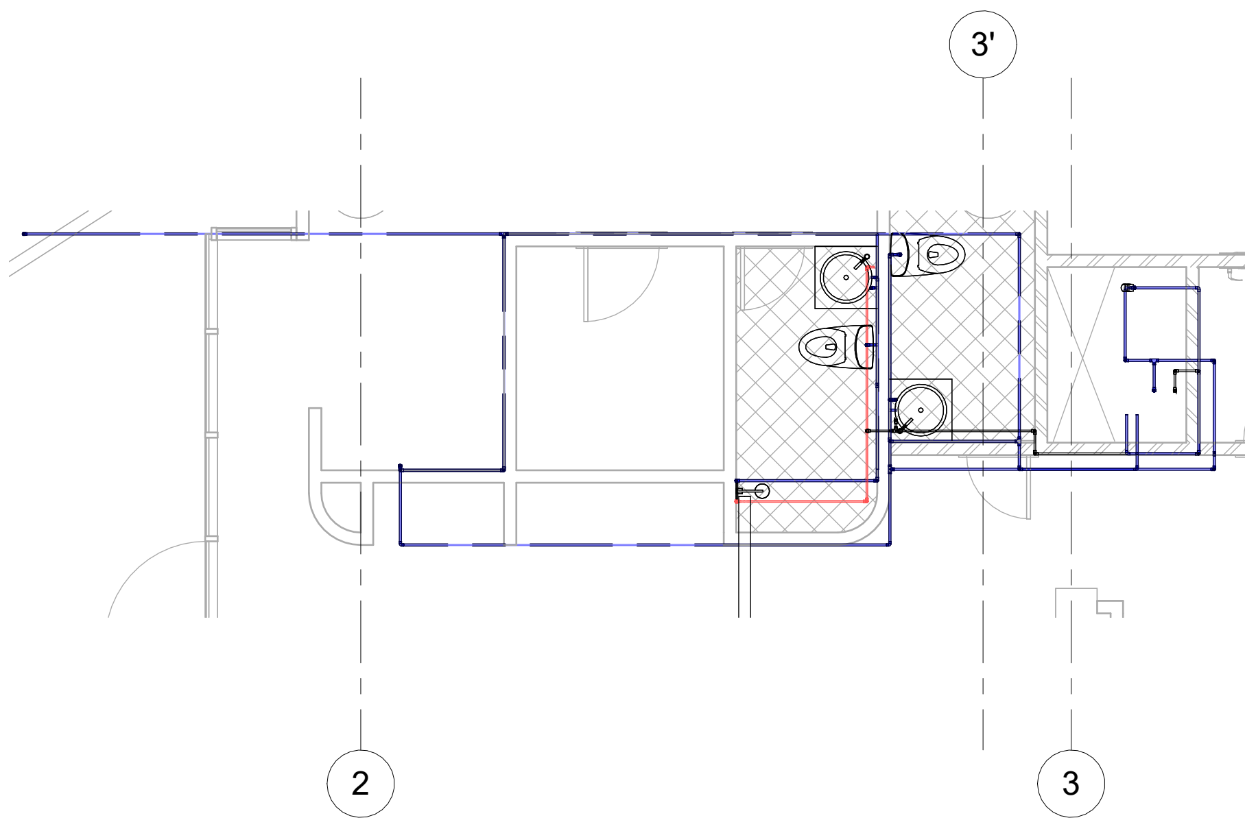
1 CL_PISO 2 - HIDRAULICO 1 : 50
