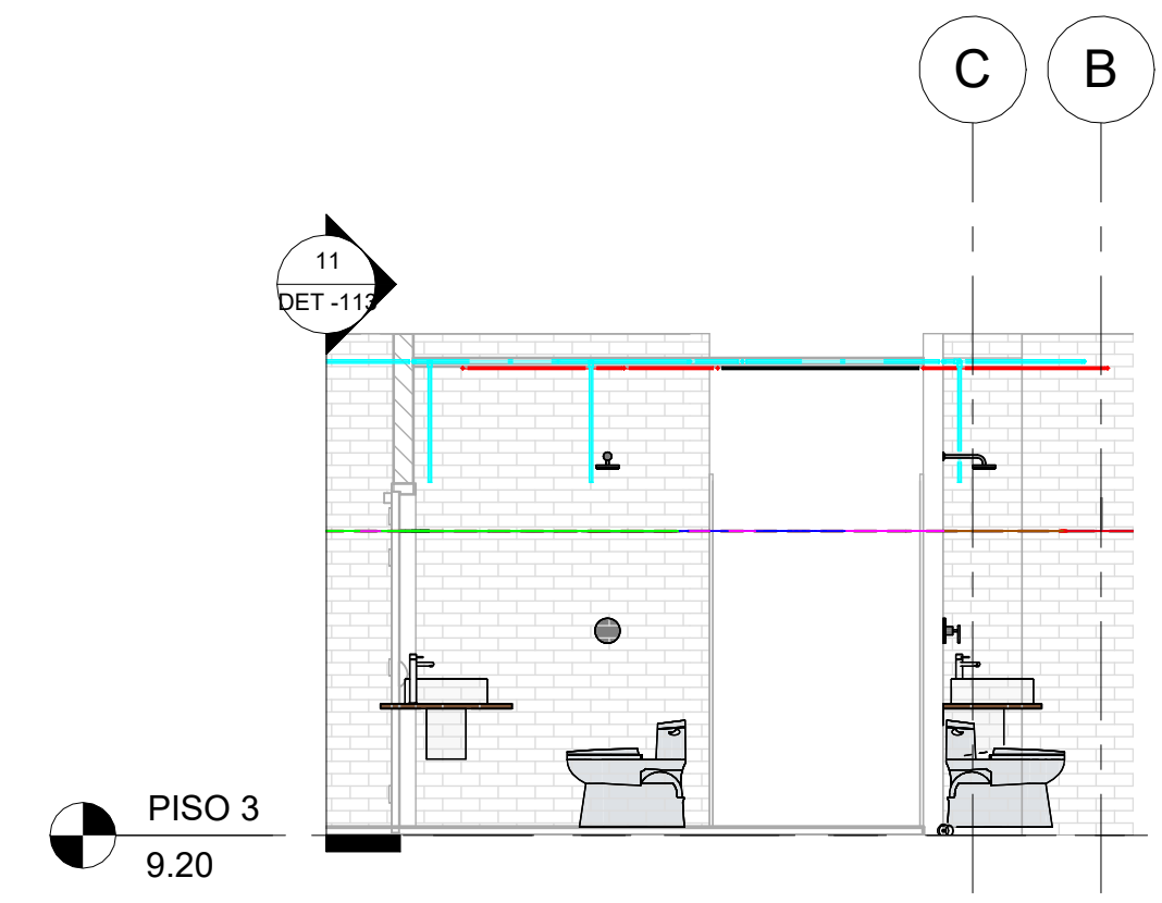
12 SEC_Trans_CL_PISO 3 - HIDRAULICO_3 1 : 50
