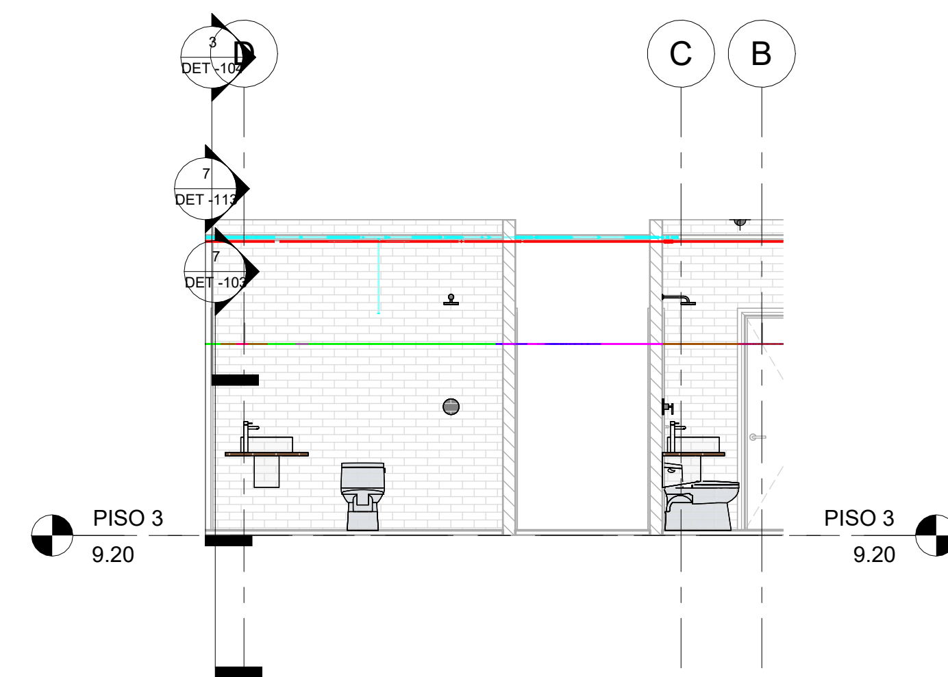
8 SEC_Trans_CL_PISO 3 - HIDRAULICO_2 1 : 50
