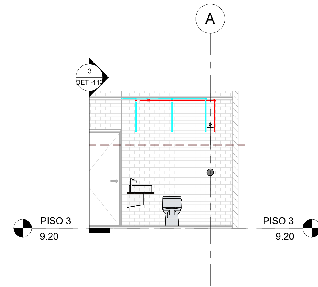
4 SEC_Trans_CL_PISO 3 - HIDRAULICO 1 : 50
