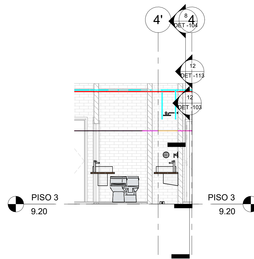
11 SEC_Long_CL_PISO 3 - HIDRAULICO_3 1 : 50
