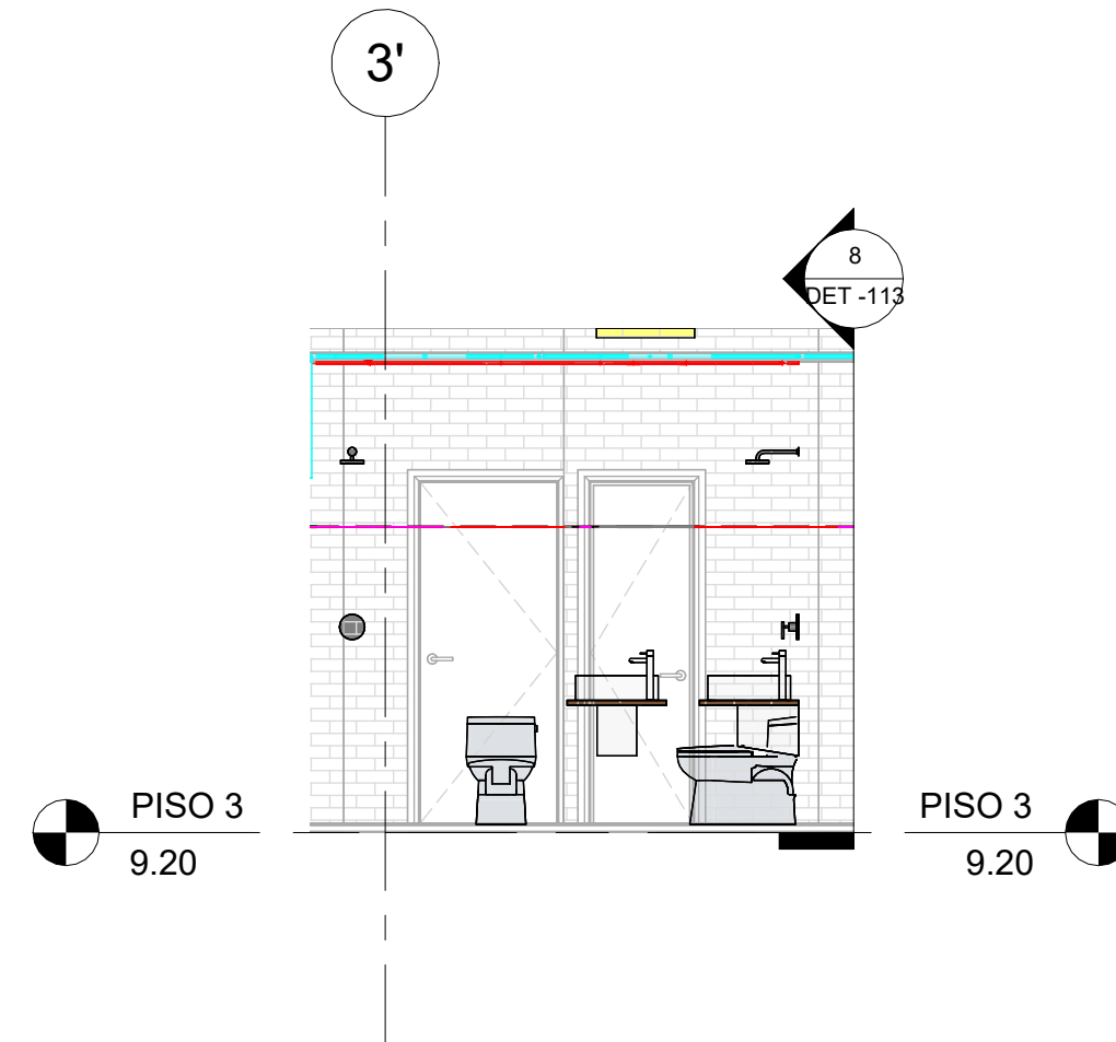
7 SEC_Long_CL_PISO 3 - HIDRAULICO_2 1 : 50
