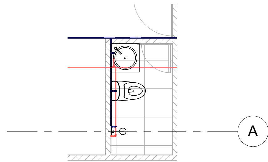
1 CL_PISO 3 - HIDRAULICO 1 : 50
