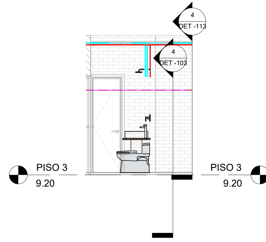
3 SEC_Long_CL_PISO 3 - HIDRAULICO 1 : 50
