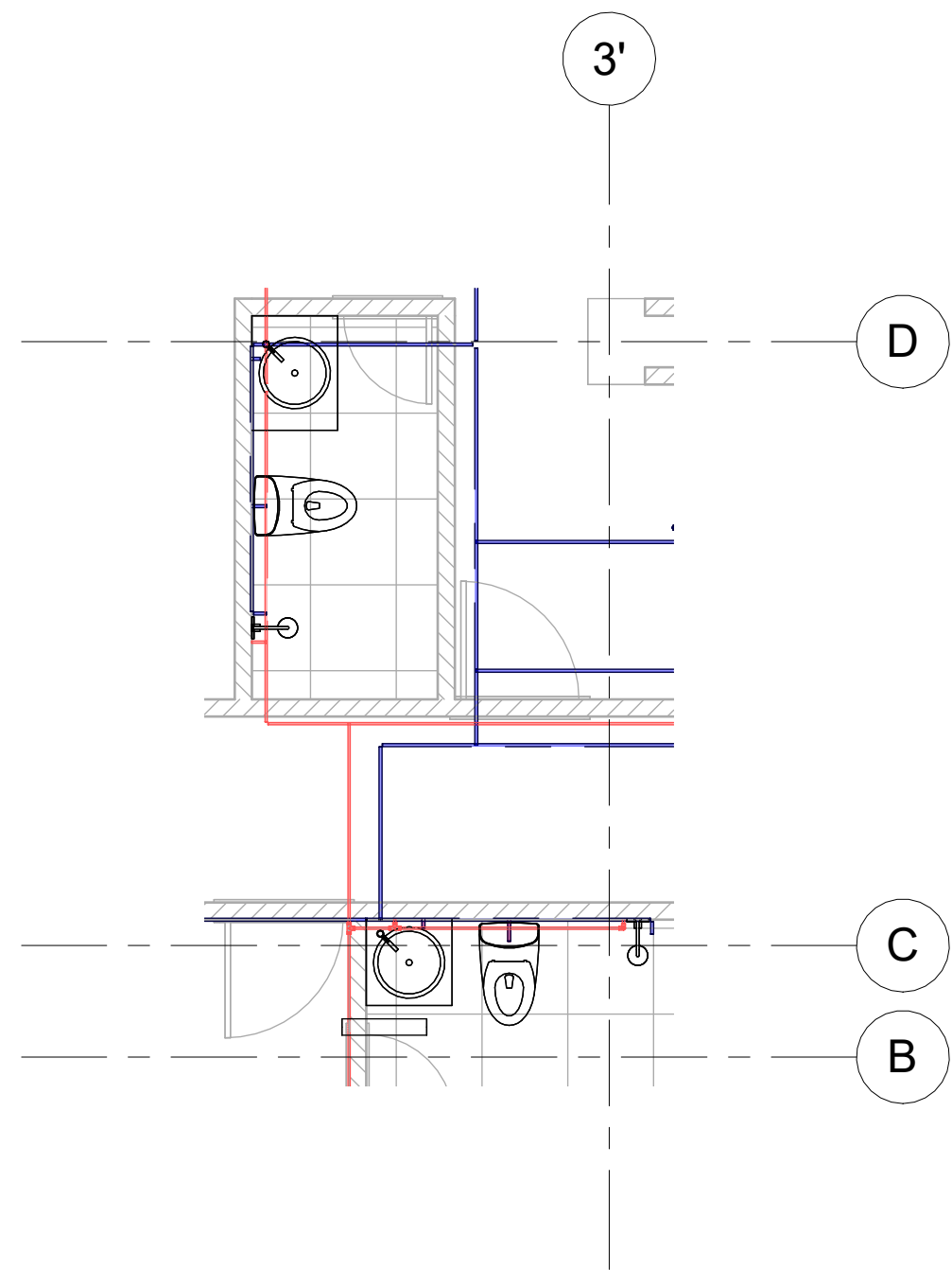
5 CL_PISO 3 - HIDRAULICO_2 1 : 50
