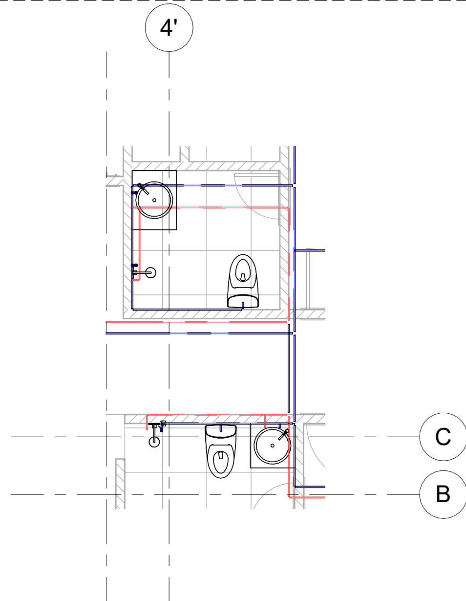
9 CL_PISO 3 - HIDRAULICO_3 1 : 50
