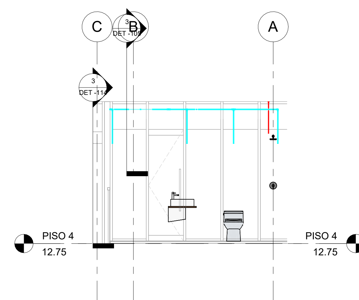
4 SEC_Trans_CL_PISO 4 - HIDRAULICO 1 : 50
