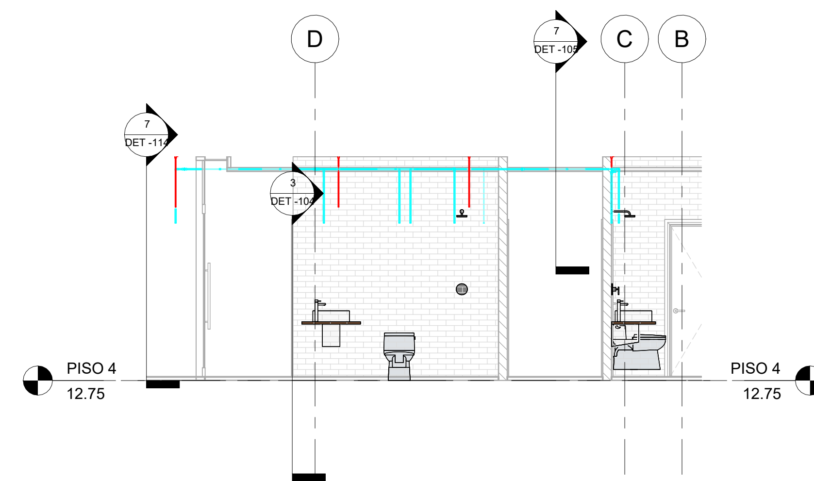
8 SEC_Trans_CL_PISO 4 - HIDRAULICO_2 1 : 50
