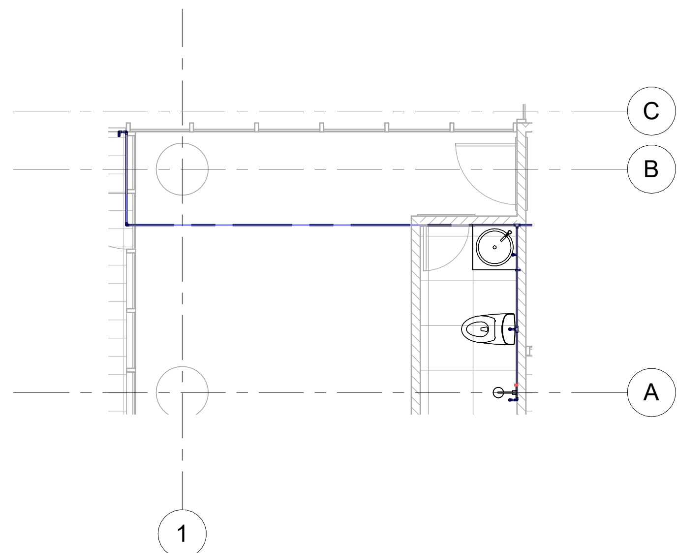
1 CL_PISO 4 - HIDRAULICO 1 : 50
