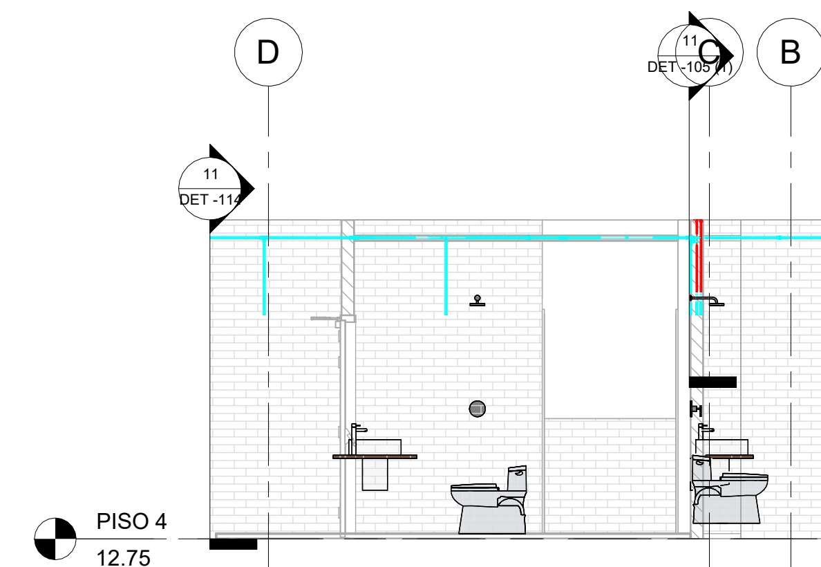
12 SEC_Trans_CL_PISO 4 - HIDRAULICO_3 1 : 50
