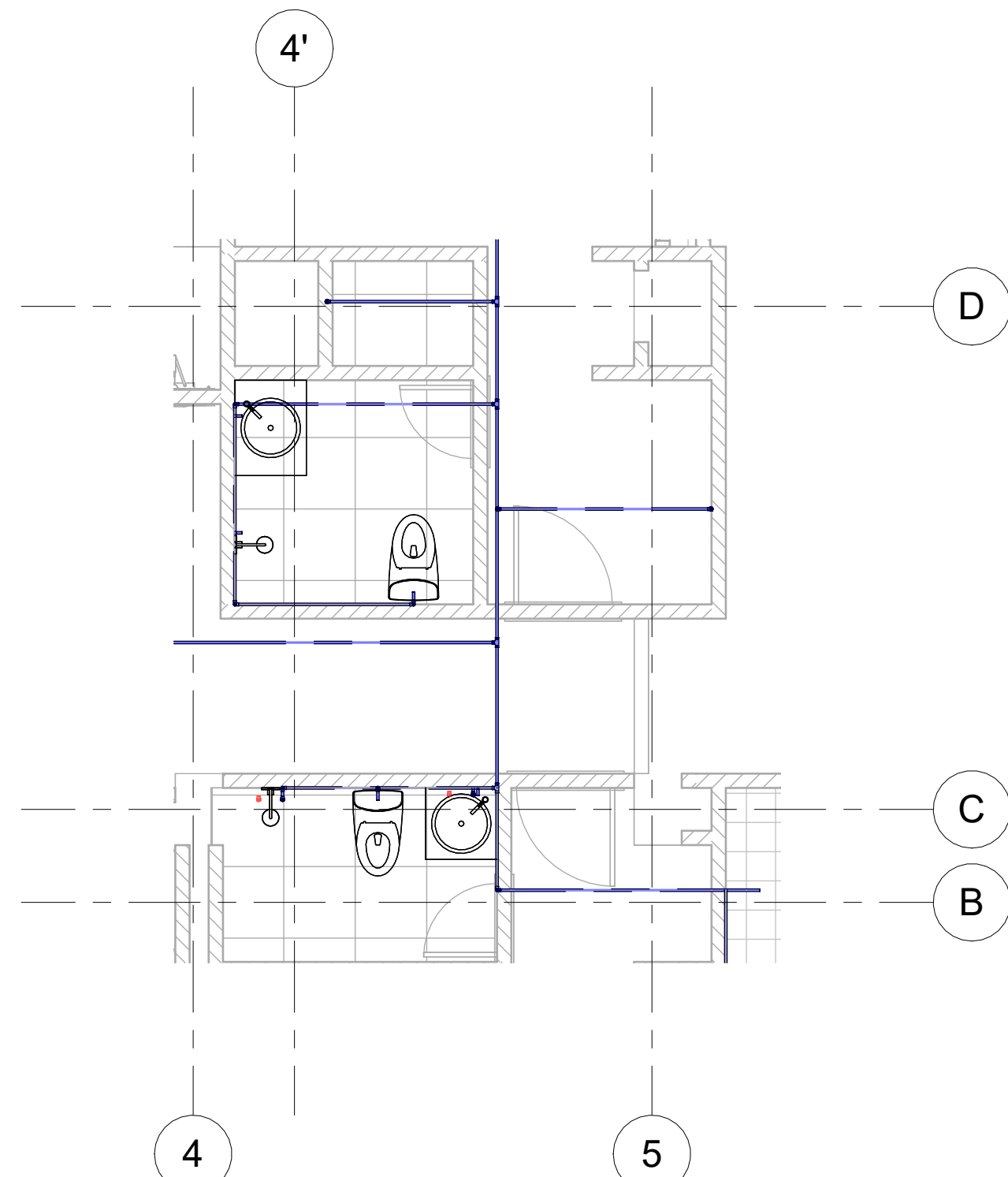
9 CL_PISO 4 - HIDRAULICO_3 1 : 50
