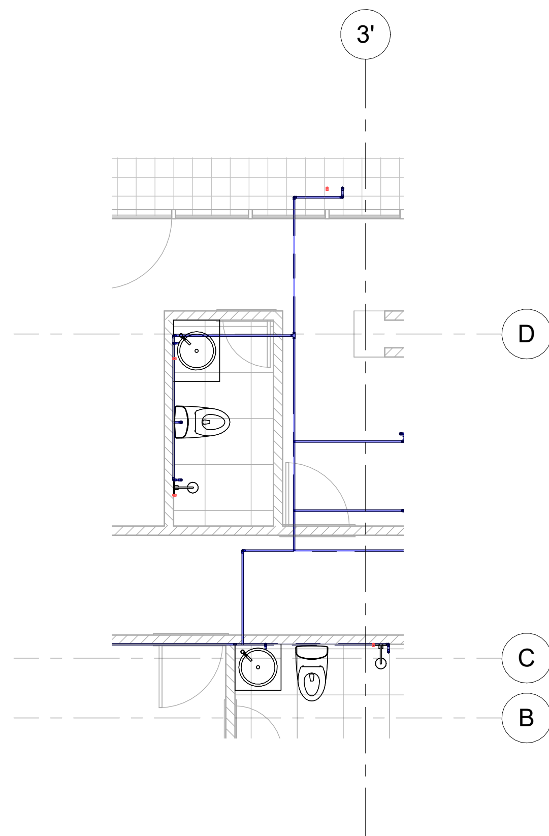
5 CL_PISO 4 - HIDRAULICO_2 1 : 50
