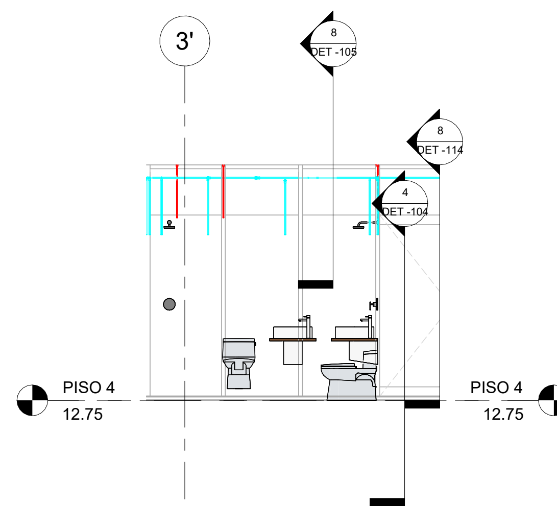
7 SEC_Long_CL_PISO 4 - HIDRAULICO_2 1 : 50
