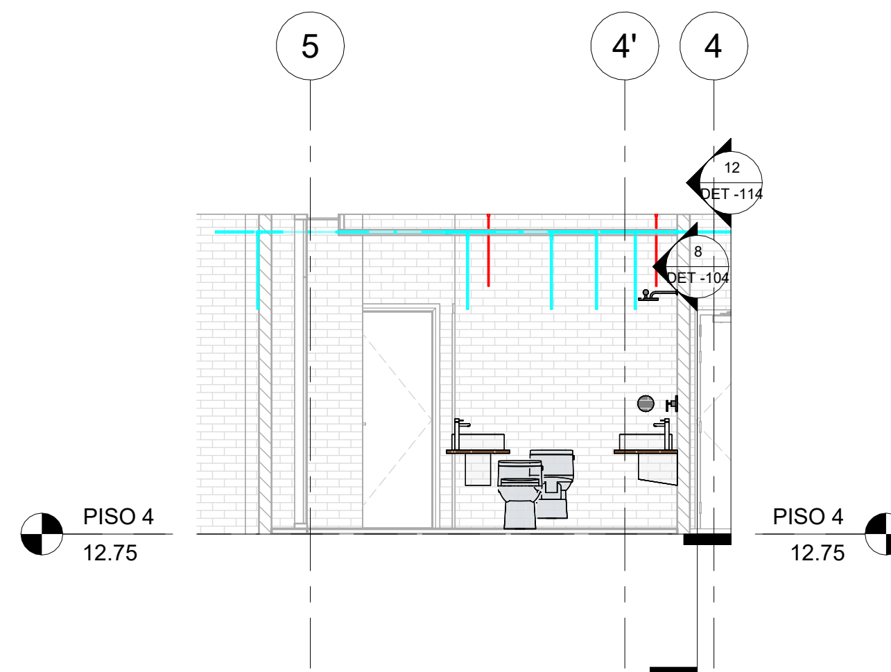
11 SEC_Long_CL_PISO 4 - HIDRAULICO_3 1 : 50
