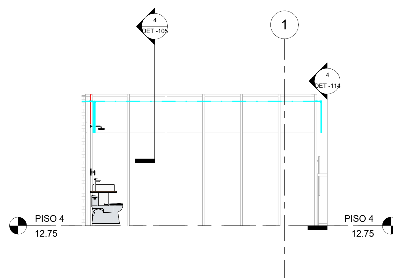
3 SEC_Long_CL_PISO 4 - HIDRAULICO 1 : 50
