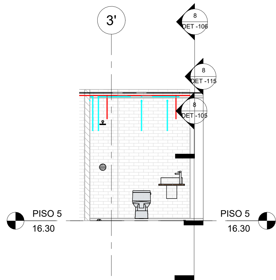
7 SEC_Long_CL_PISO 5 - HIDRAULICO_2 1 : 50
