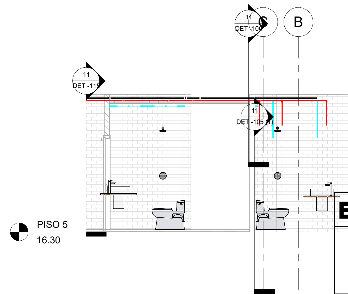
12 SEC_Trans_CL_PISO 5 - HIDRAULICO_3 1 : 50
