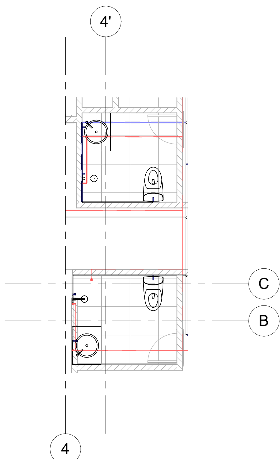
9 CL_PISO 5 - HIDRAULICO_3 1 : 50
