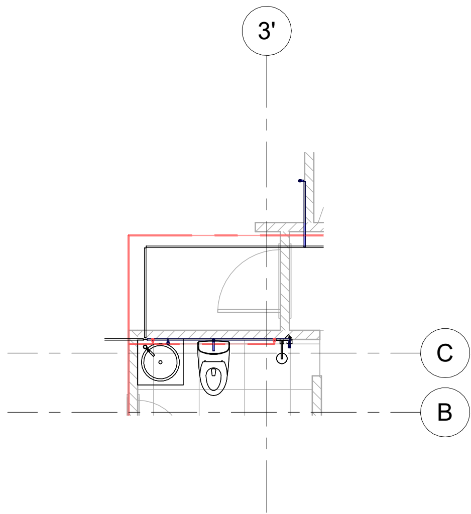
5 CL_PISO 5 - HIDRAULICO_2 1 : 50
