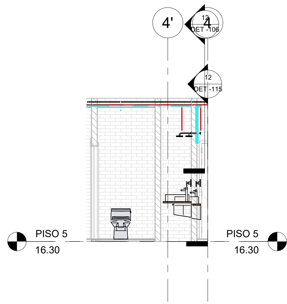
11 SEC_Long_CL_PISO 5 - HIDRAULICO_3 1 : 50
