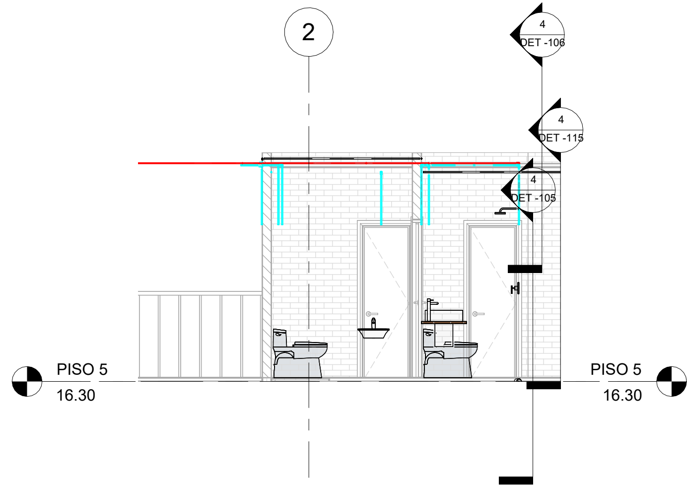
3 SEC_Long_CL_PISO 5 - HIDRAULICO 1 : 50
