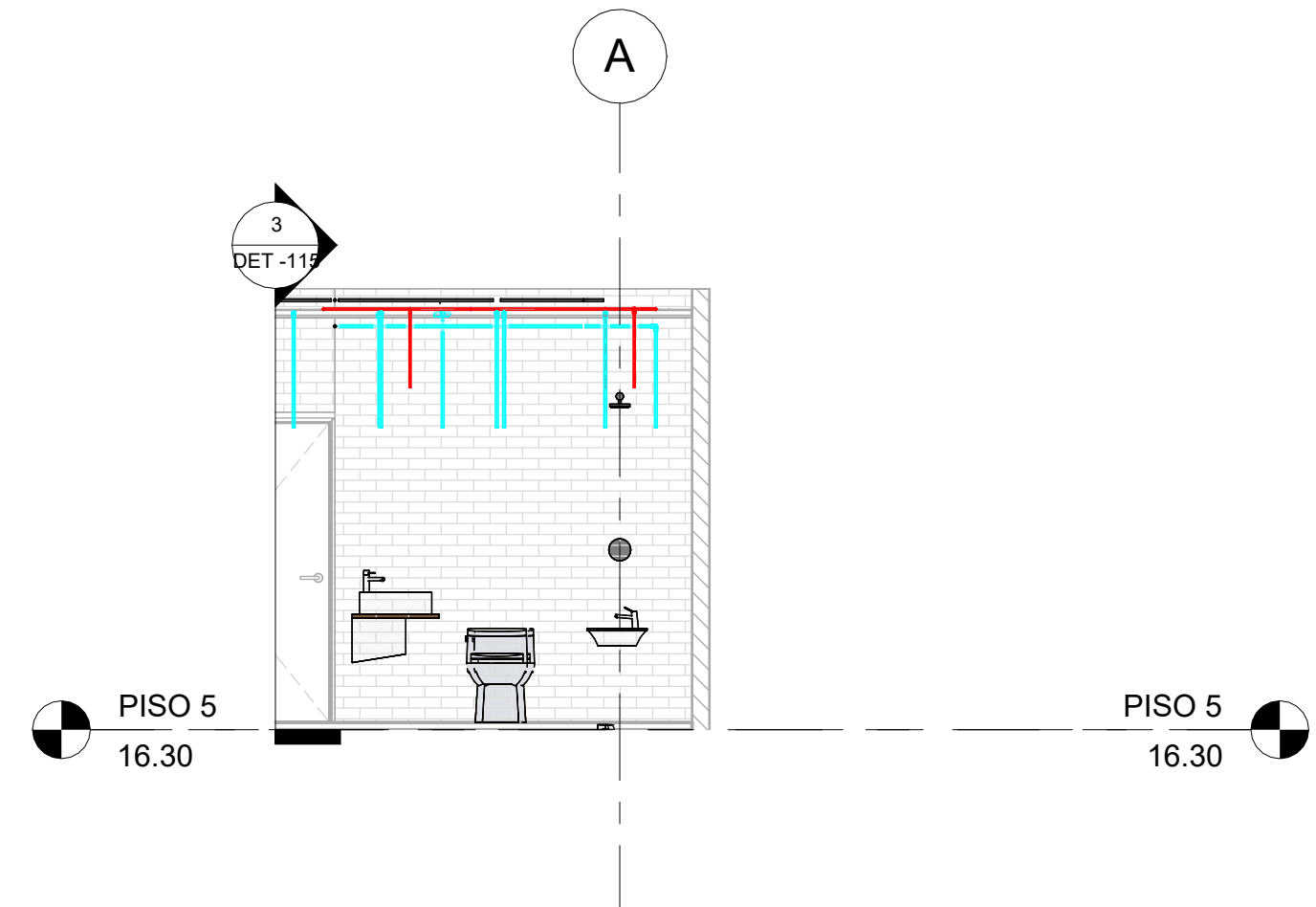
4 SEC_Trans_CL_PISO 5 - HIDRAULICO 1 : 50
