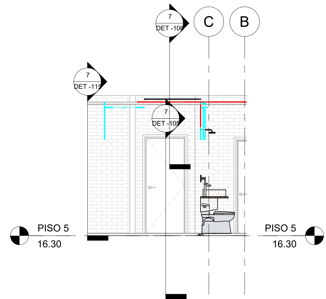
8 SEC_Trans_CL_PISO 5 - HIDRAULICO_2 1 : 50
