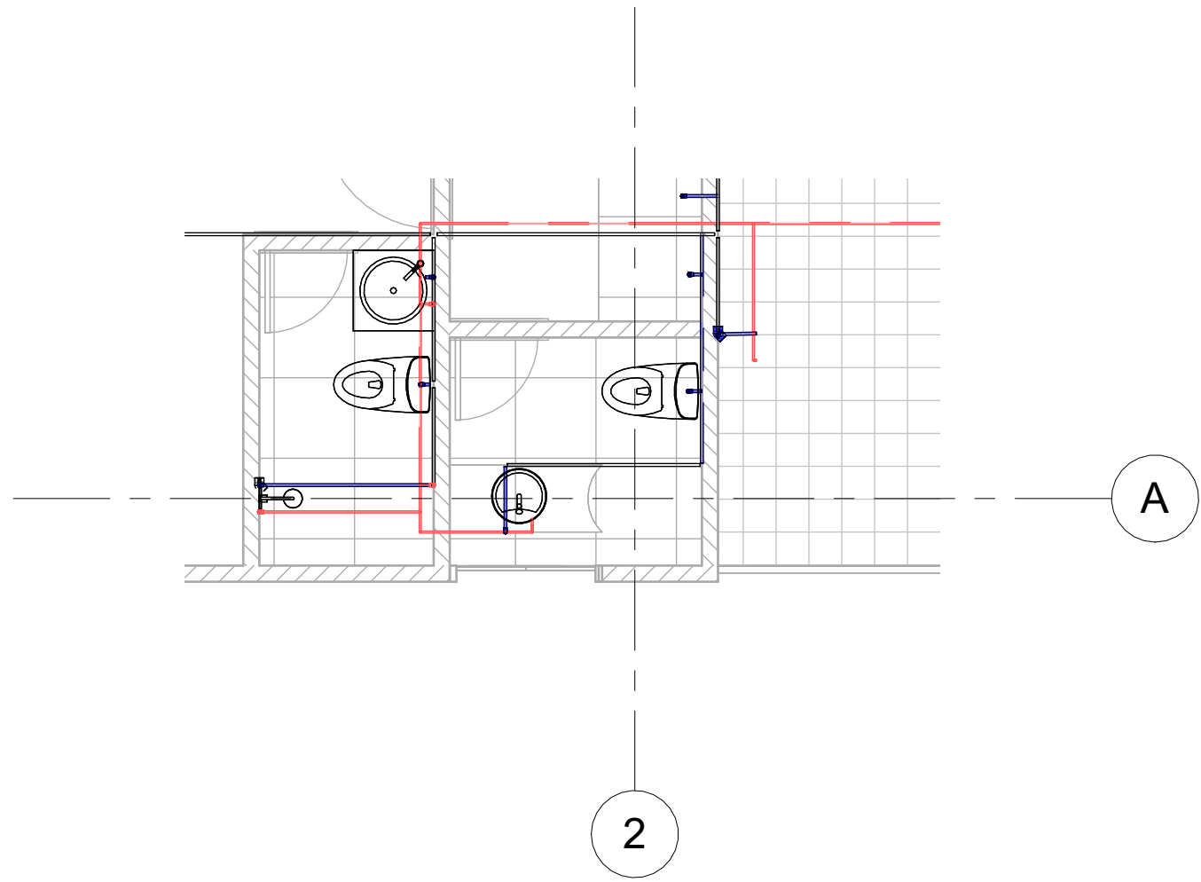
1 CL_PISO 5 - HIDRAULICO 1 : 50
