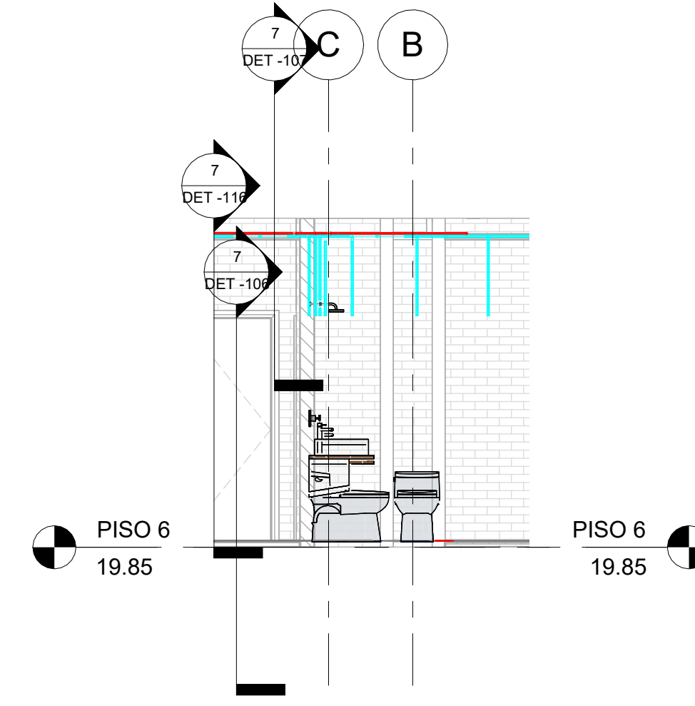
8 SEC_Trans_CL_PISO 6 - HIDRAULICO_2 1 : 50
