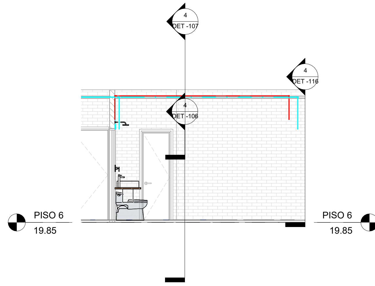
3 SEC_Long_CL_PISO 6 - HIDRAULICO 1 : 50
