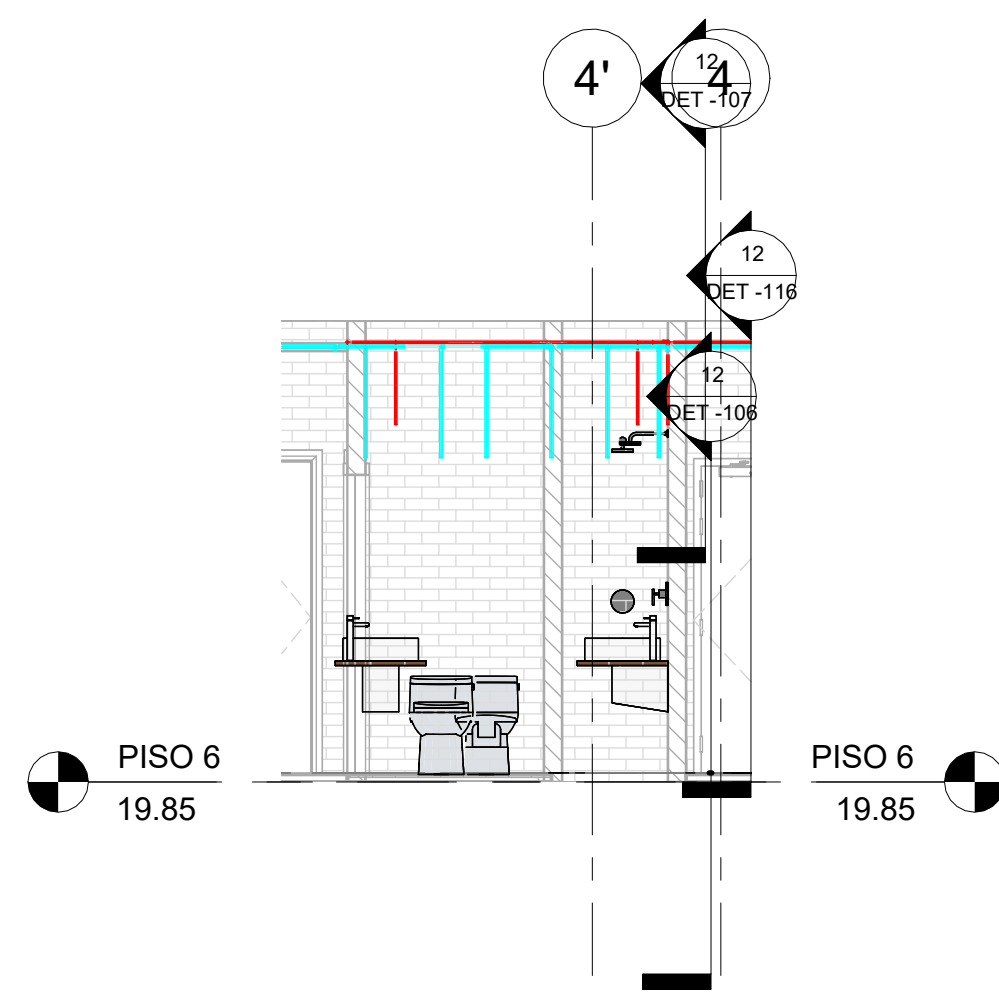
11 SEC_Long_CL_PISO 6 - HIDRAULICO_3 1 : 50
