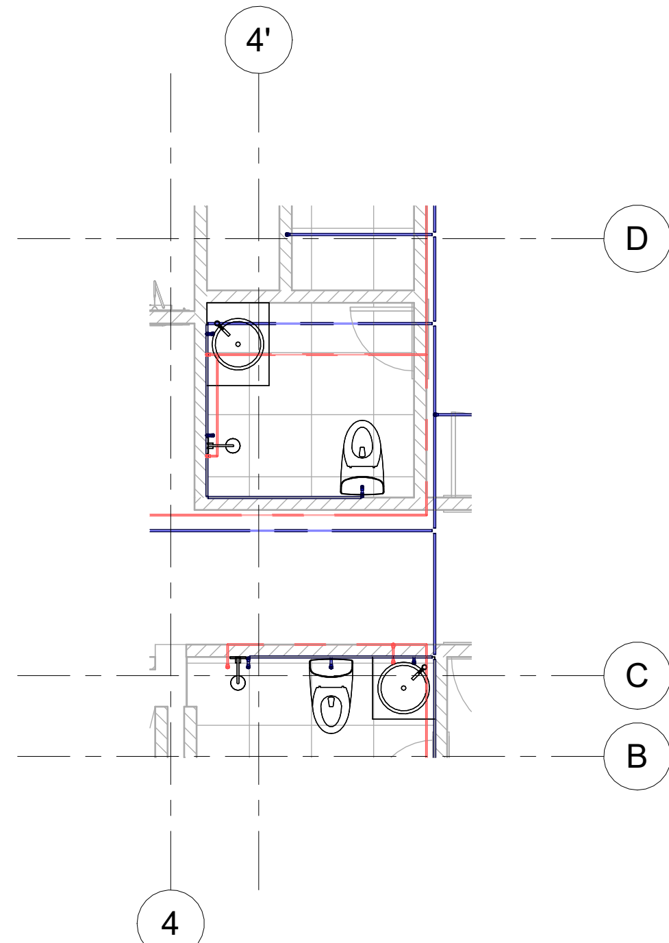
9 CL_PISO 6 - HIDRAULICO_3 1 : 50
