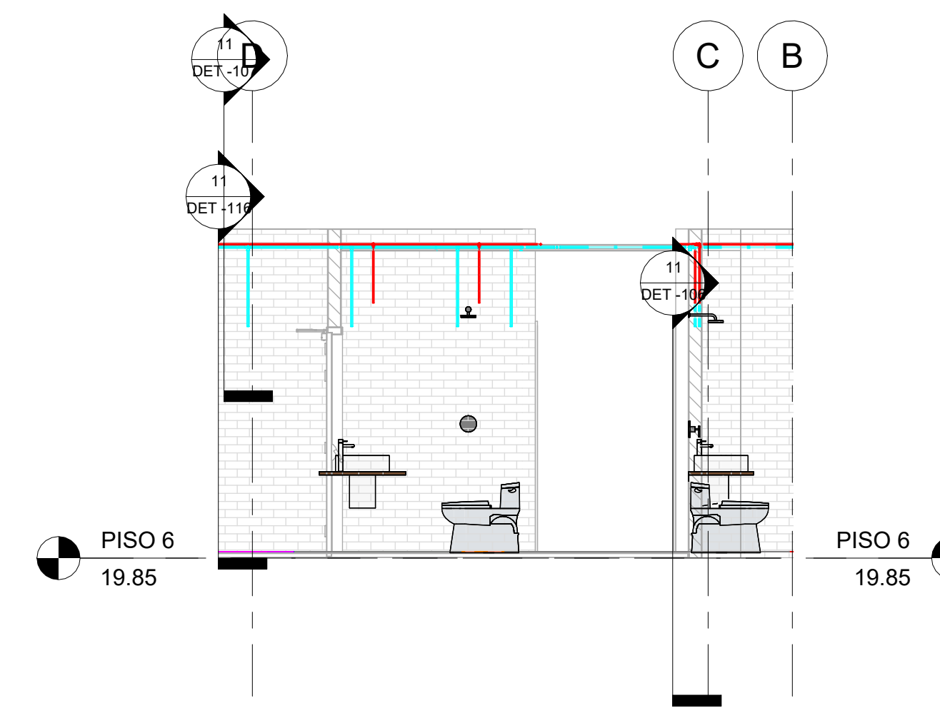
12 SEC_Trans_CL_PISO 6 - HIDRAULICO_3 1 : 50
