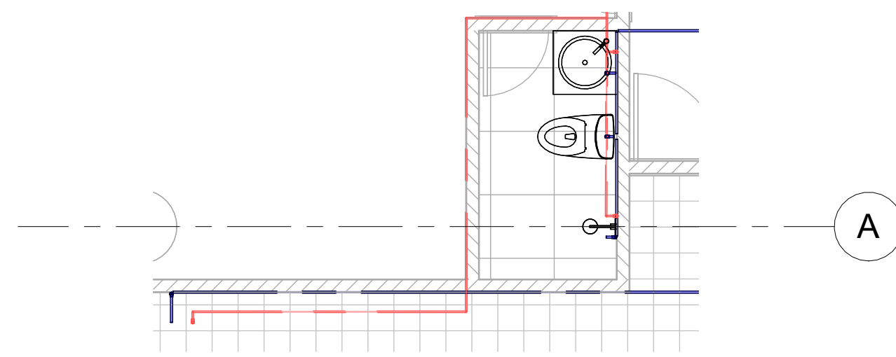
1 CL_PISO 6 - HIDRAULICO 1 : 50
