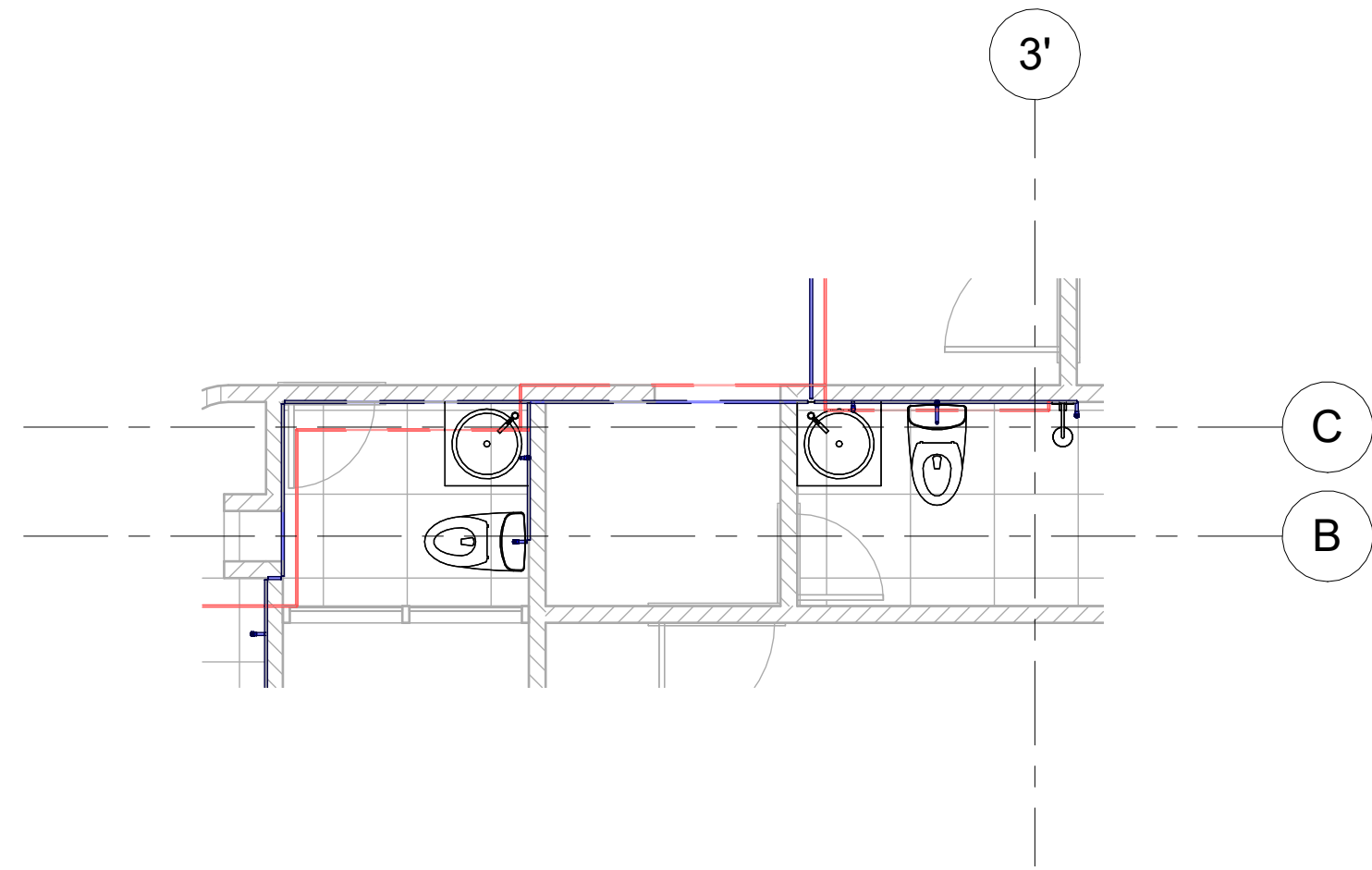
5 CL_PISO 6 - HIDRAULICO_2 1 : 50
