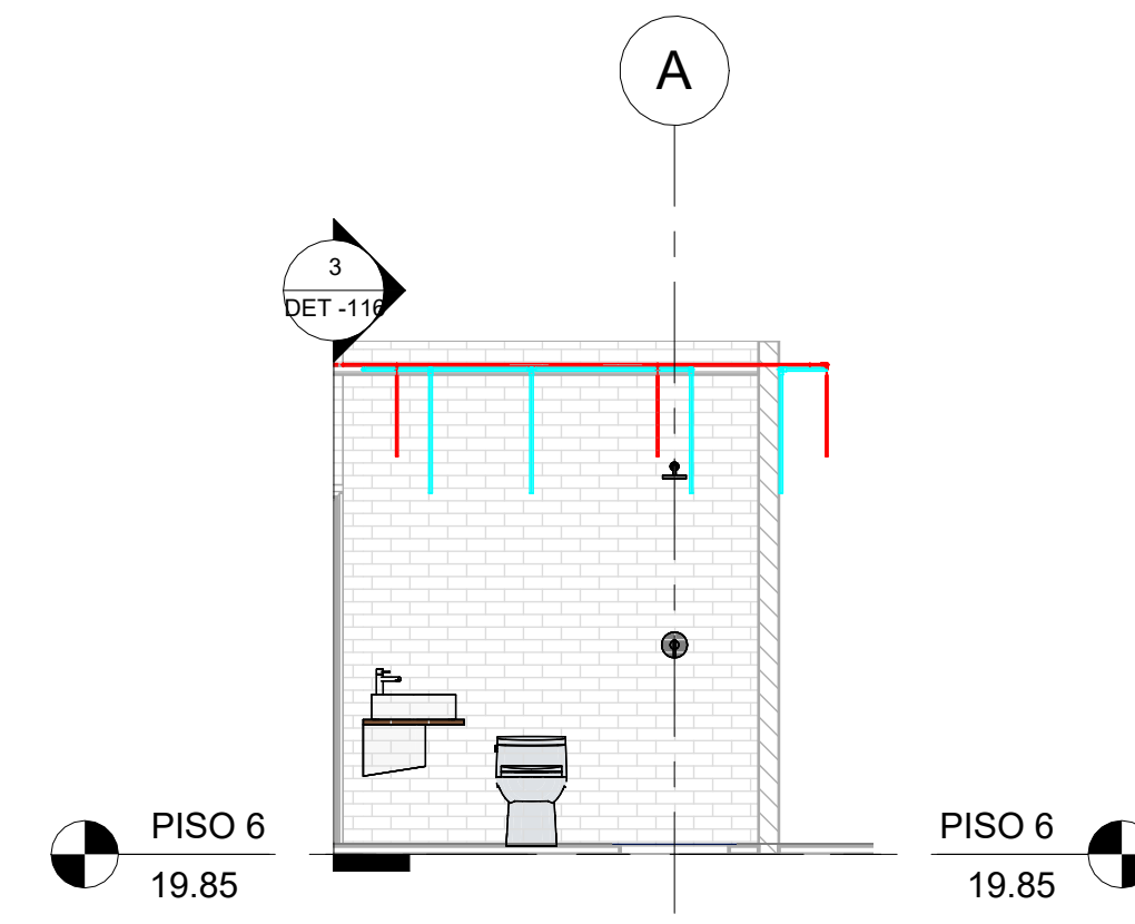
4 SEC_Trans_CL_PISO 6 - HIDRAULICO 1 : 50
