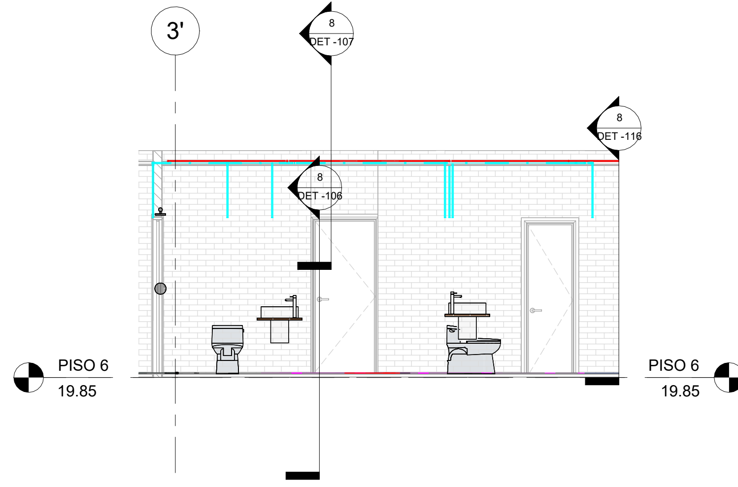
7 SEC_Long_CL_PISO 6 - HIDRAULICO_2 1 : 50
