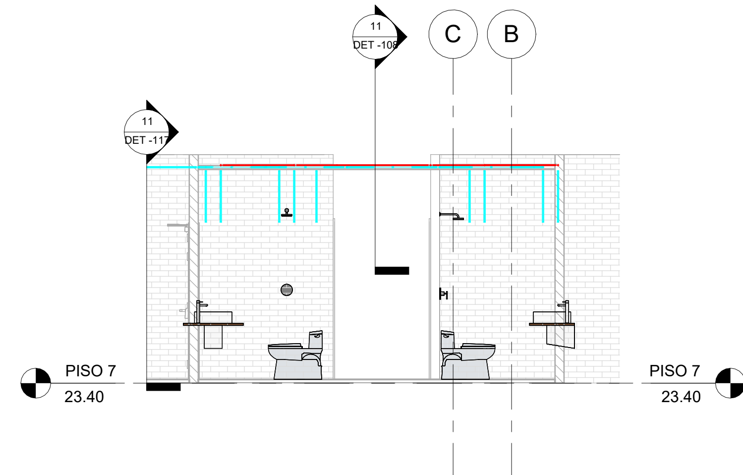
12 SEC_Trans_CL_PISO 7 - HIDRAULICO_3 1 : 50
