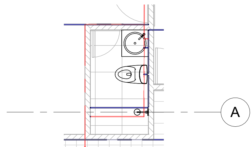
1 CL_PISO 7 - HIDRAULICO 1 : 50
