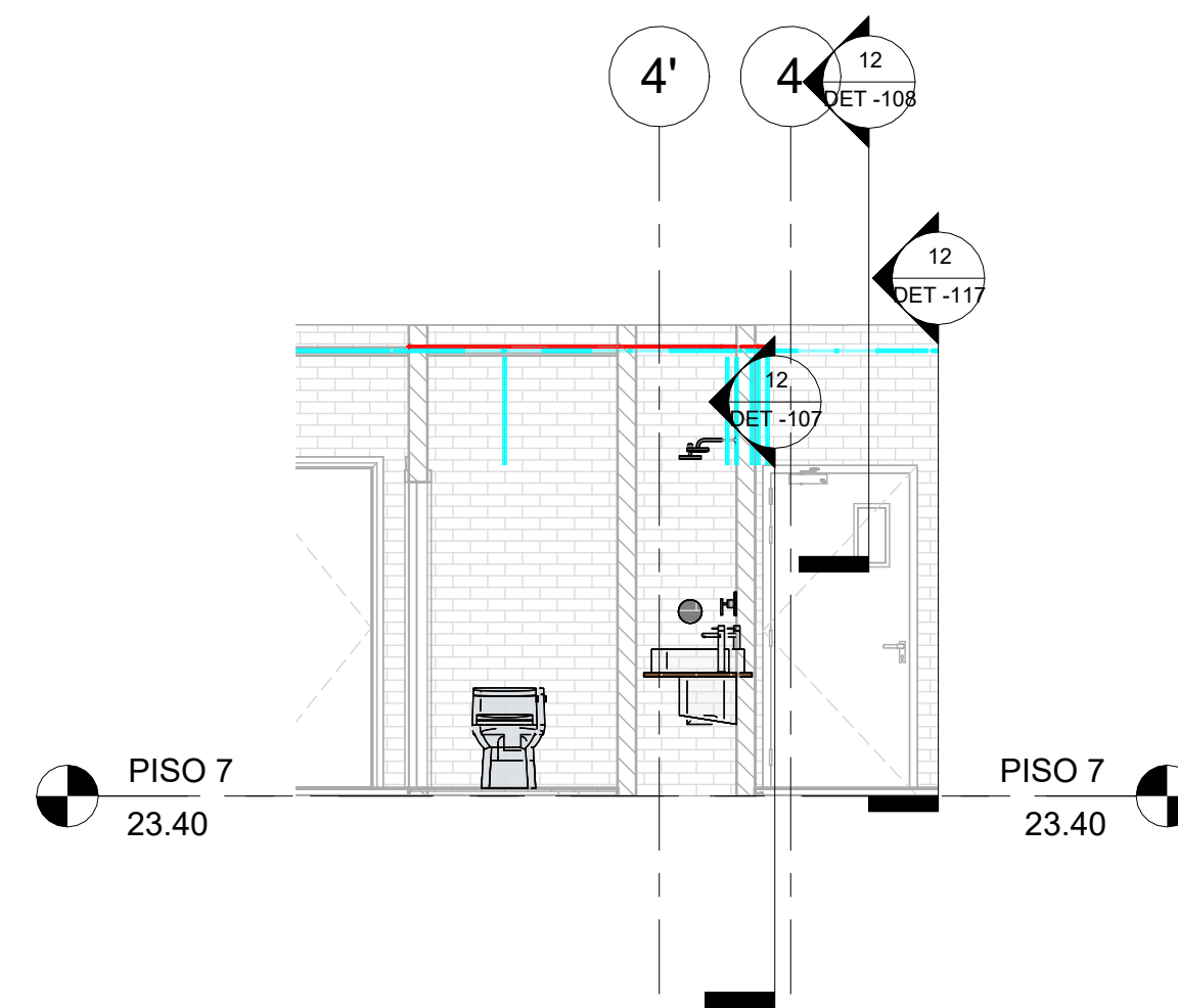
11 SEC_Long_CL_PISO 7 - HIDRAULICO_3 1 : 50
