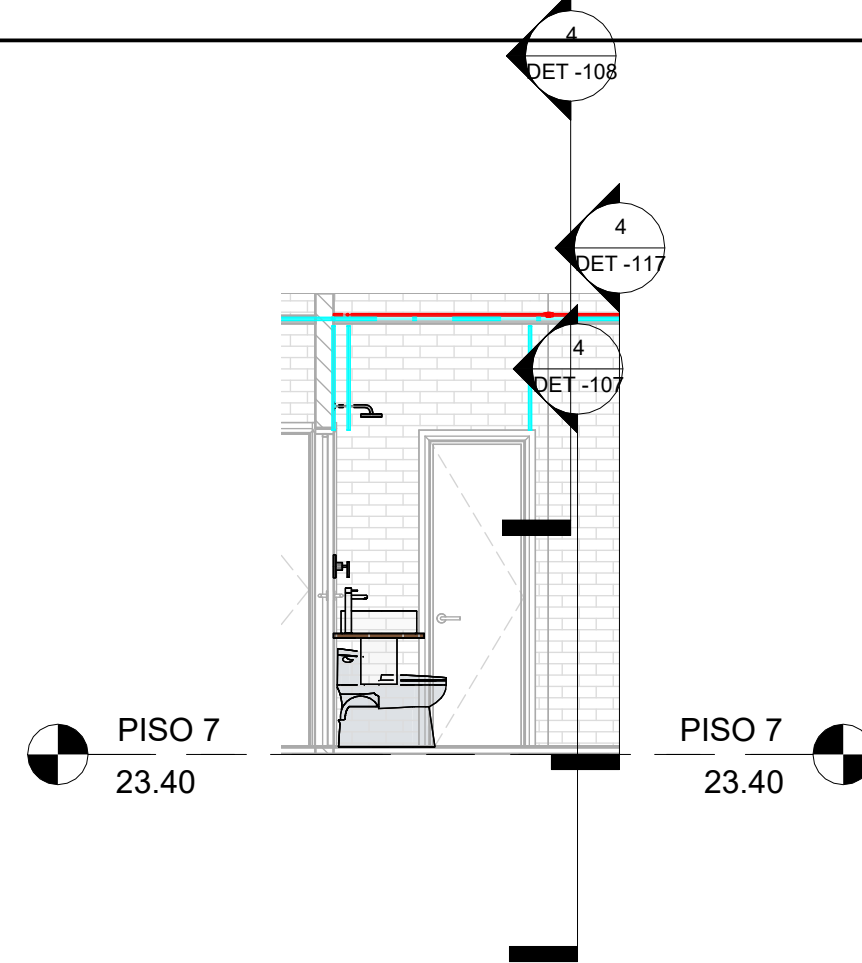
3 SEC_Long_CL_PISO 7 - HIDRAULICO 1 : 50
