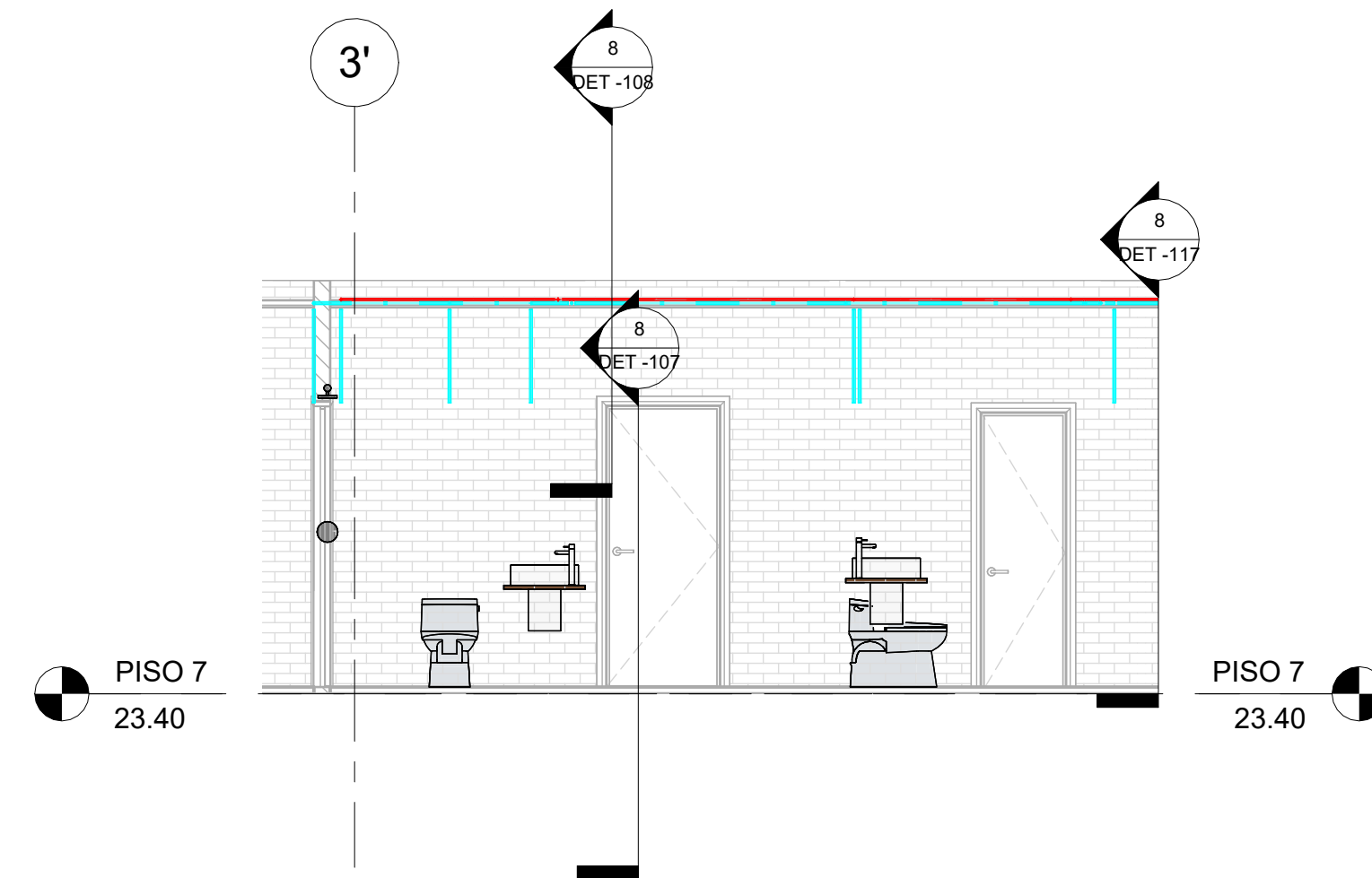
7 SEC_Long_CL_PISO 7 - HIDRAULICO_2 1 : 50
