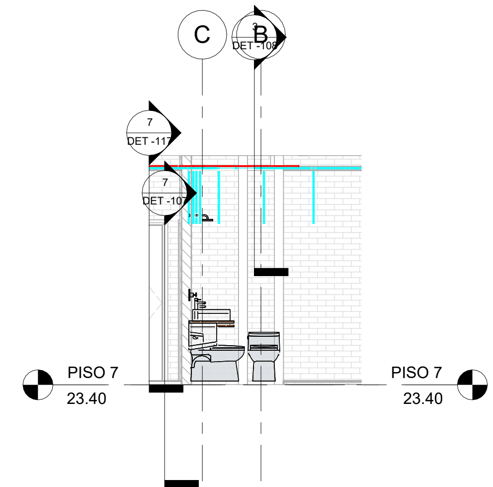
8 SEC_Trans_CL_PISO 7 - HIDRAULICO_2 1 : 50
