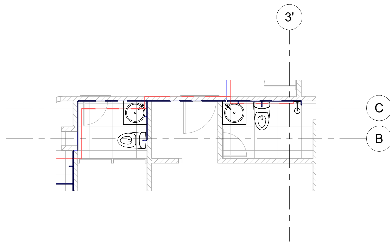
5 CL_PISO 7 - HIDRAULICO_2 1 : 50
