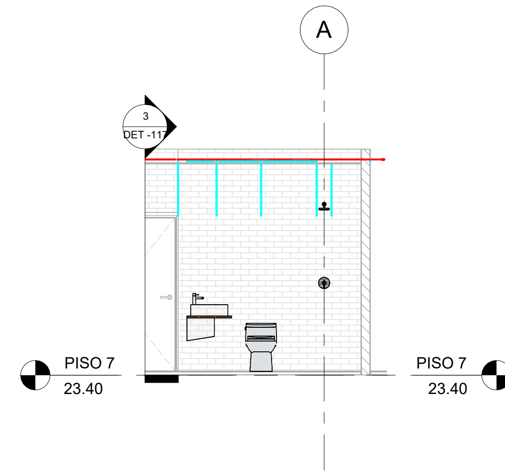
4 SEC_Trans_CL_PISO 7 - HIDRAULICO 1 : 50
