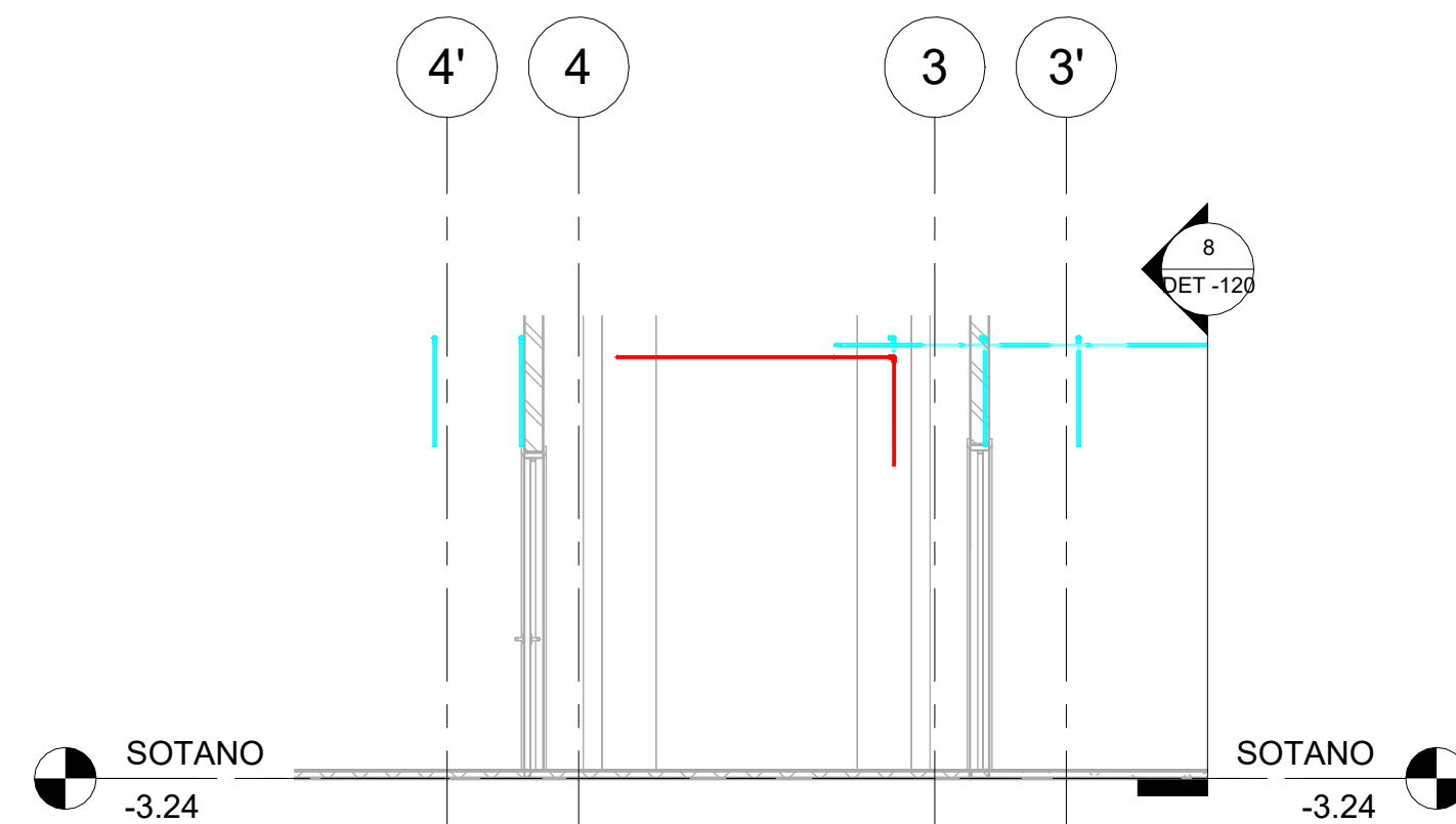
7 SEC_Long_CL_SOTANO - HIDRAULICO_2 1 : 50
