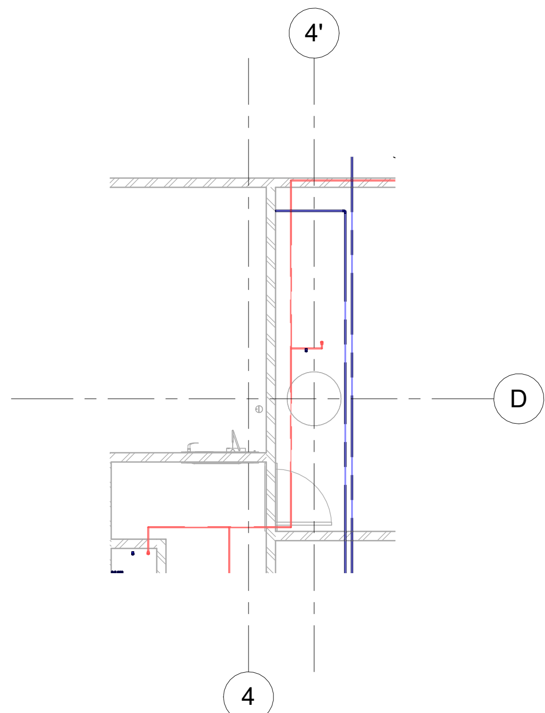
9 CL_SOTANO - HIDRAULICO_3 1 : 50
