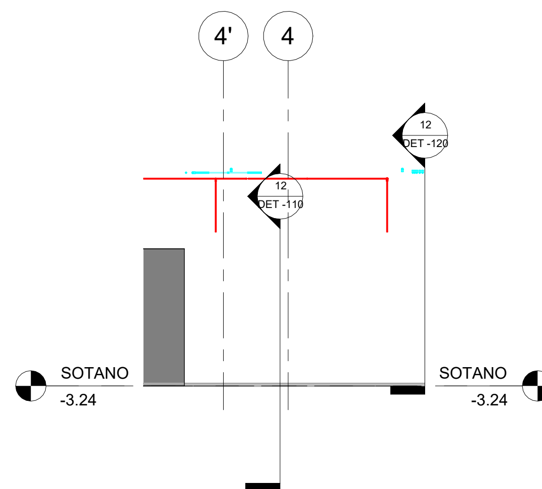
11 SEC_Long_CL_SOTANO - HIDRAULICO_3 1 : 50
