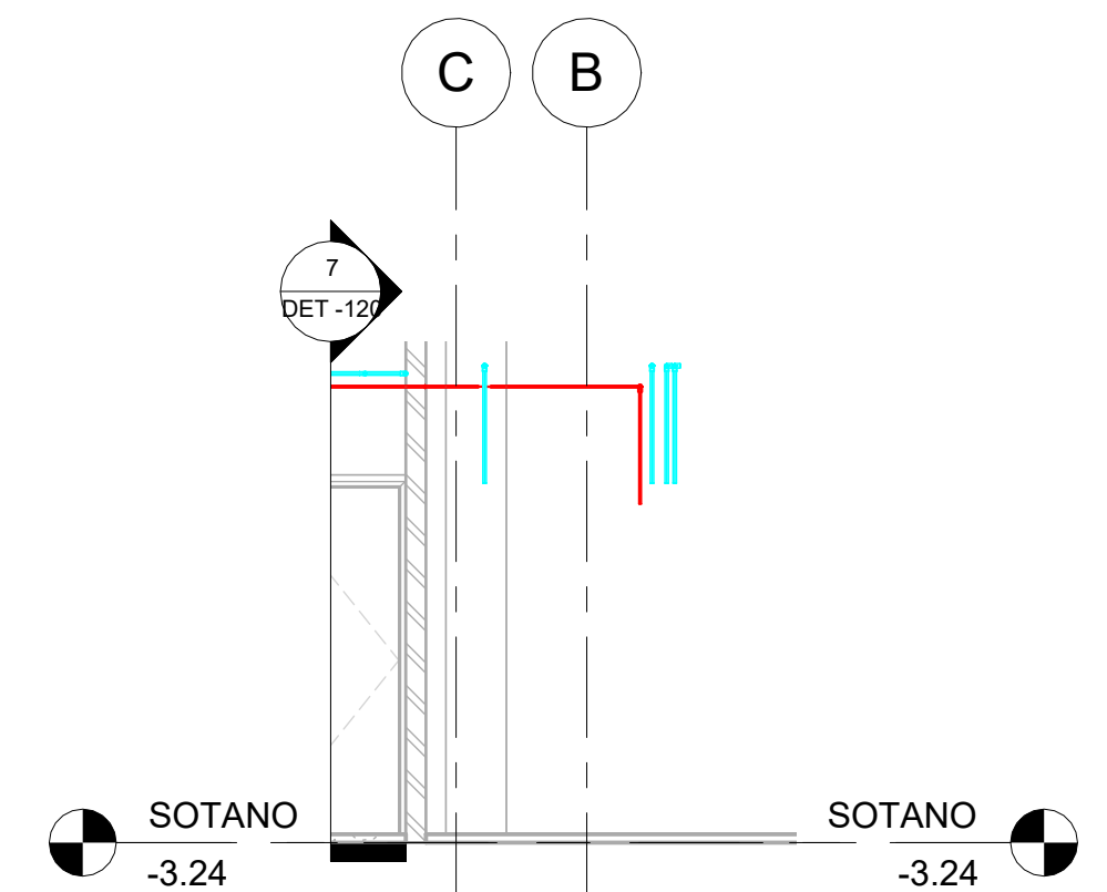
8 SEC_Trans_CL_SOTANO - HIDRAULICO_2 1 : 50
