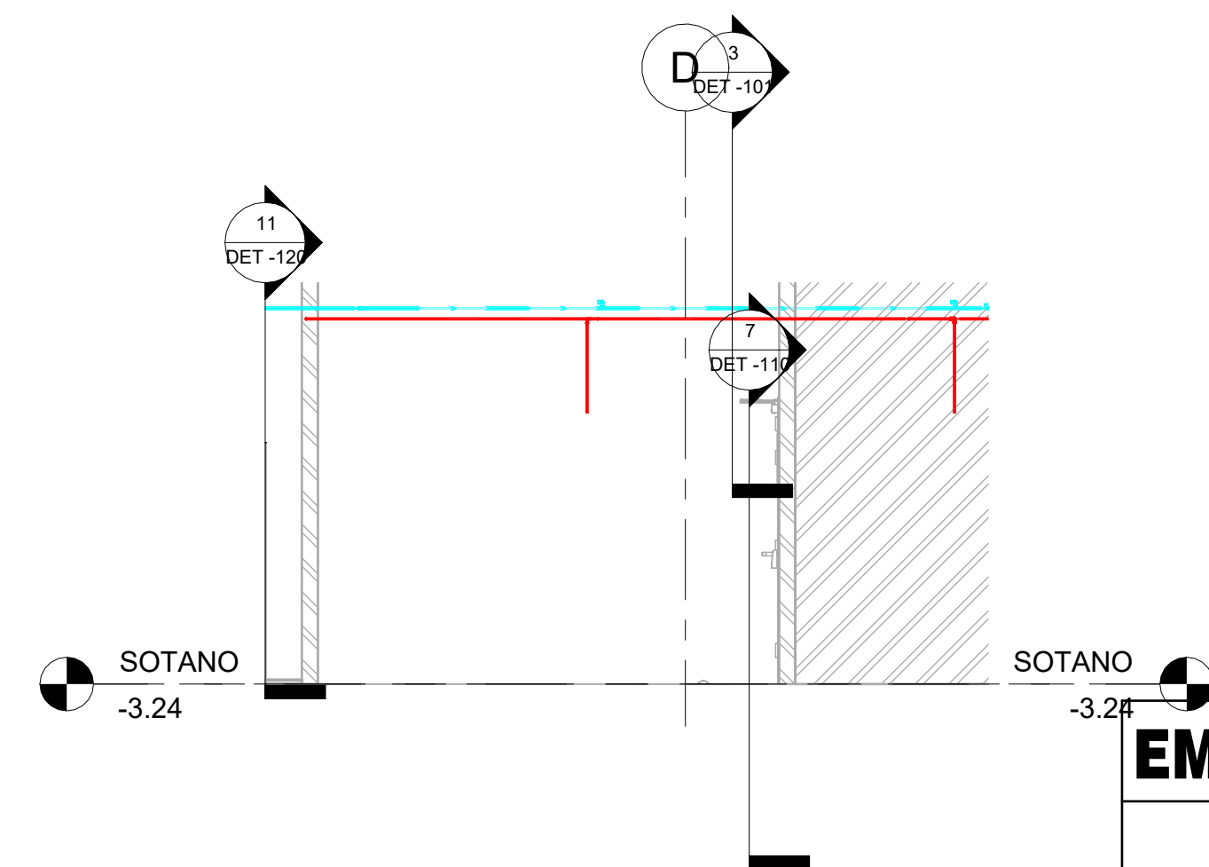
7 SEC_Long_CL_SOTANO - HIDRAULICO_2 1 : 50
