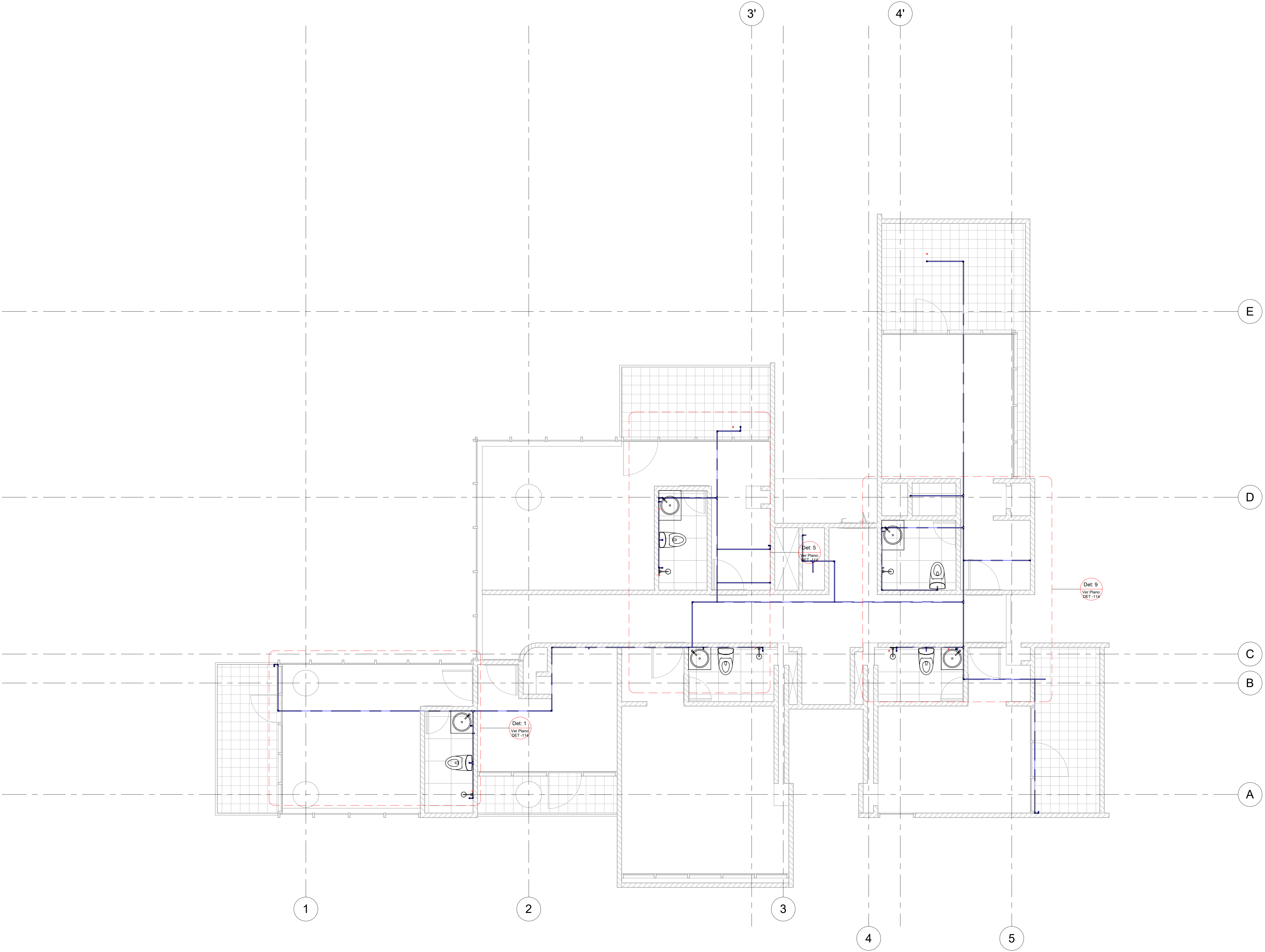
1 PISO 4 - HIDRAULICO 1 : 50
