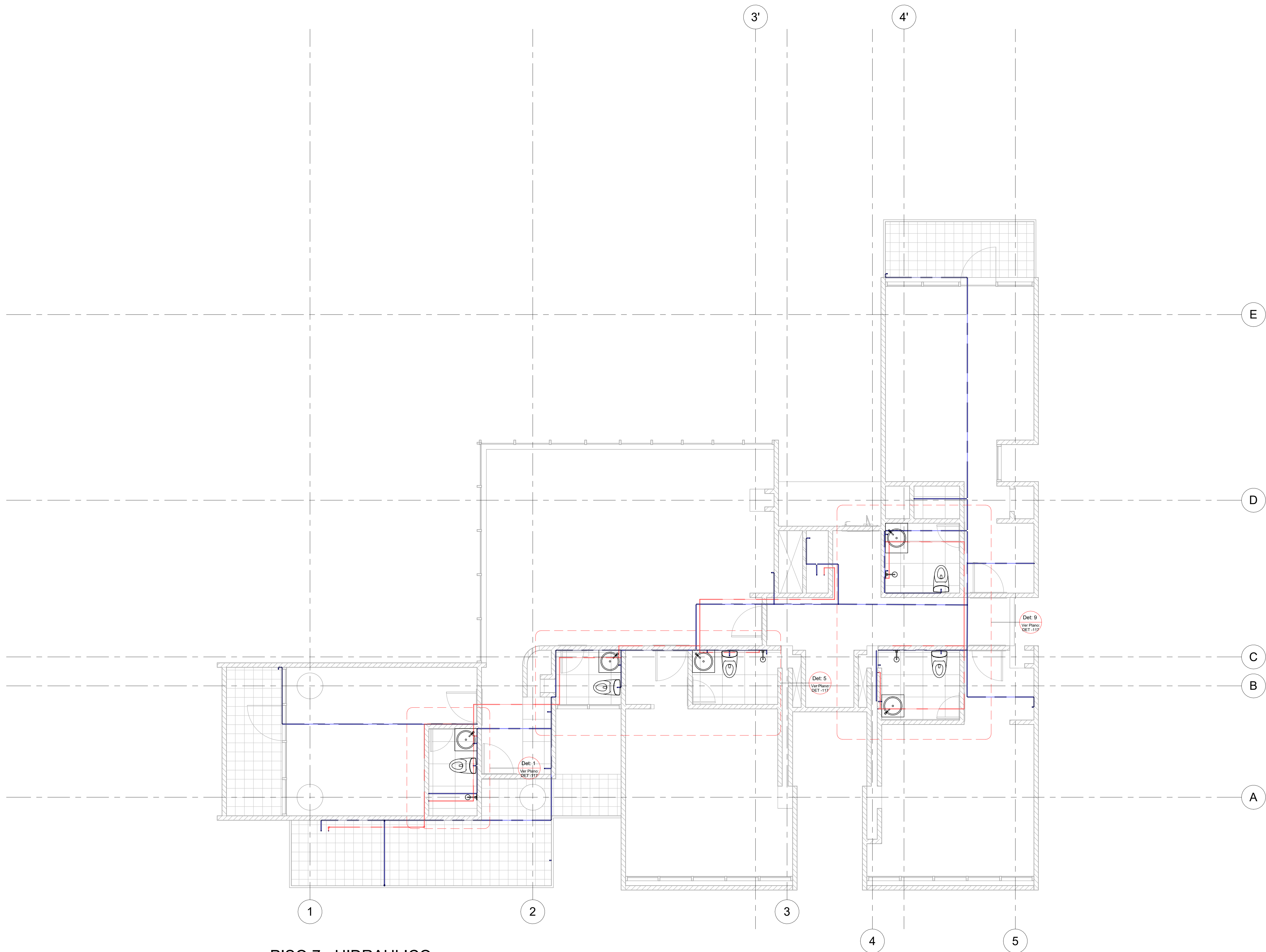
1 PISO 7 - HIDRAULICO 1 : 50
