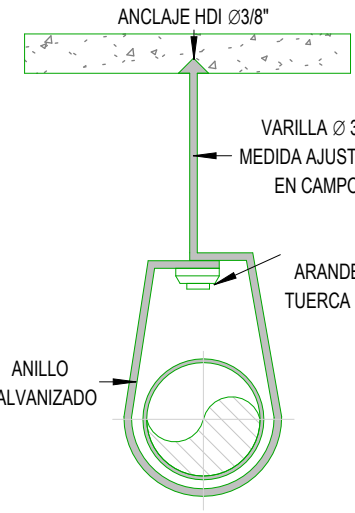
DETALLE SOPORTE TIPO PERA 1 : 20
