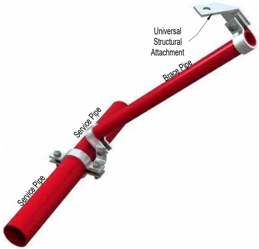
DETALLE SOPORTE SISMORESISTENTE LATERAL 1 : 125
