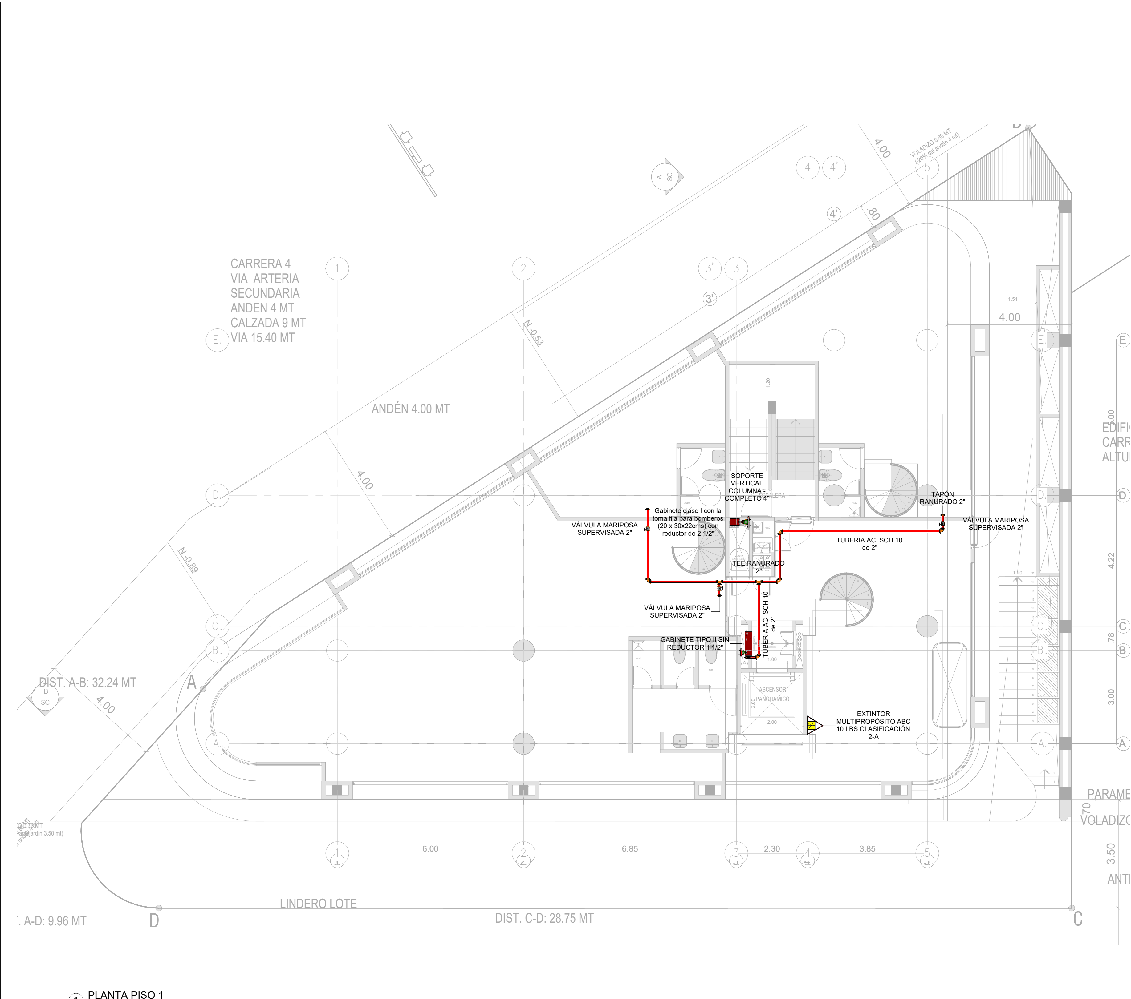
1 PLANTA PISO 1 1 : 75
