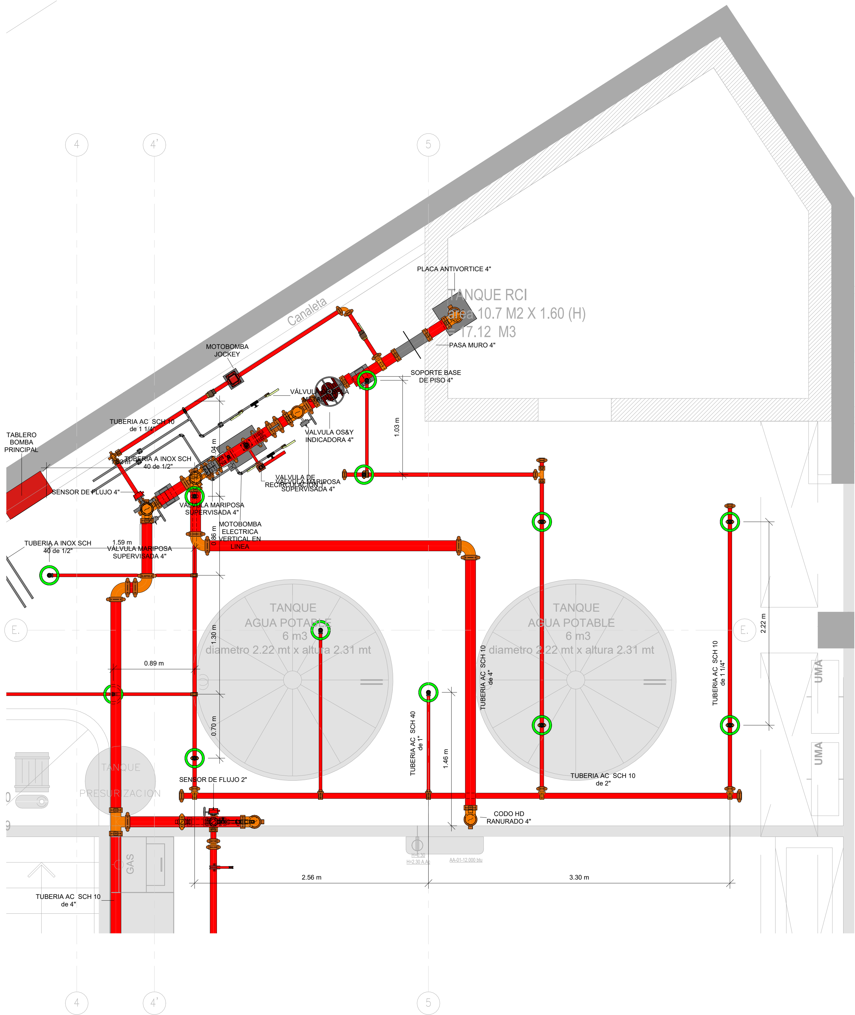
1 PLANTA CUARTO DE BOMBAS RCI 1 : 25
