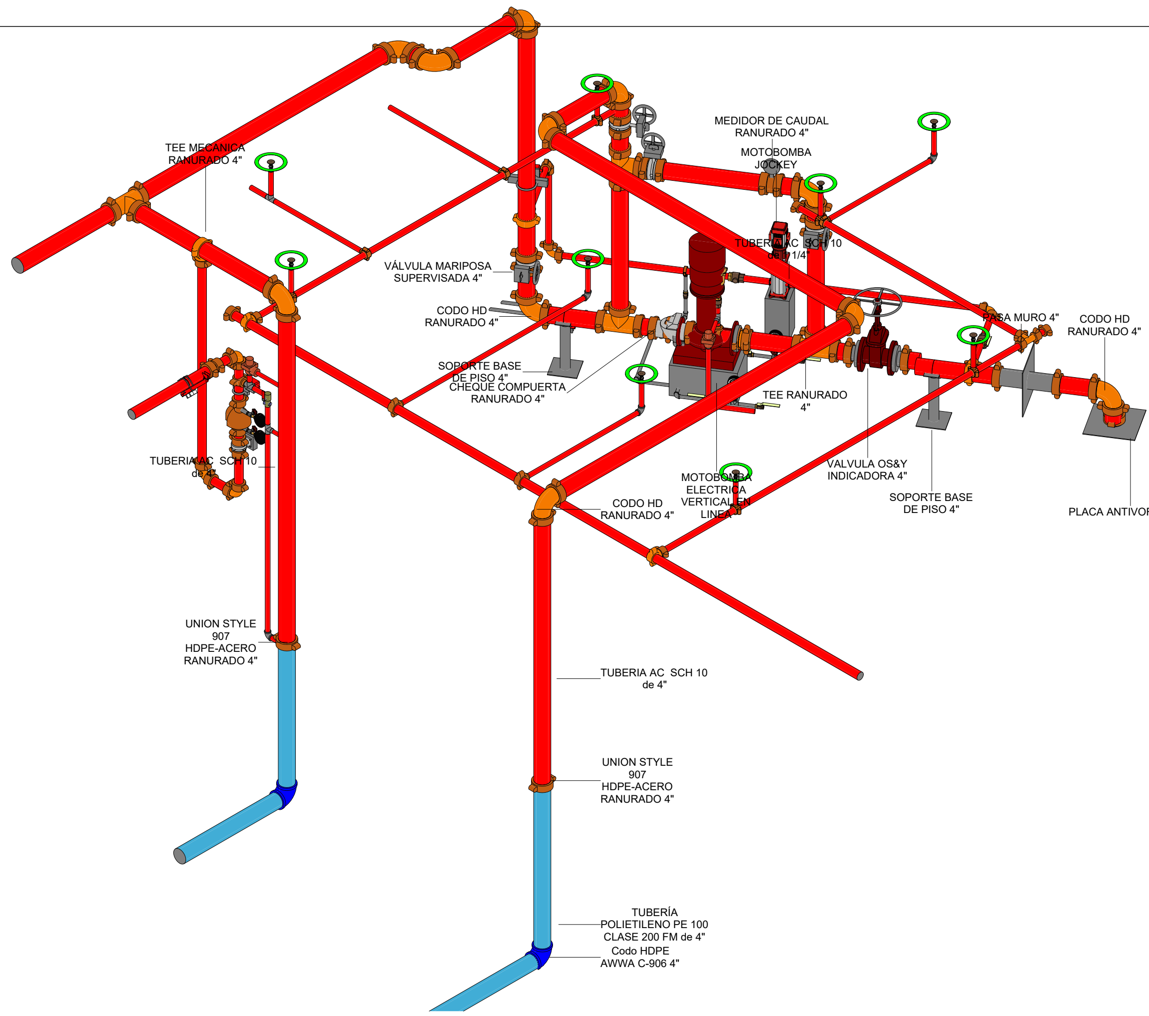
2 ISOMETRÍA CUARTO DE BOMBAS RCI
