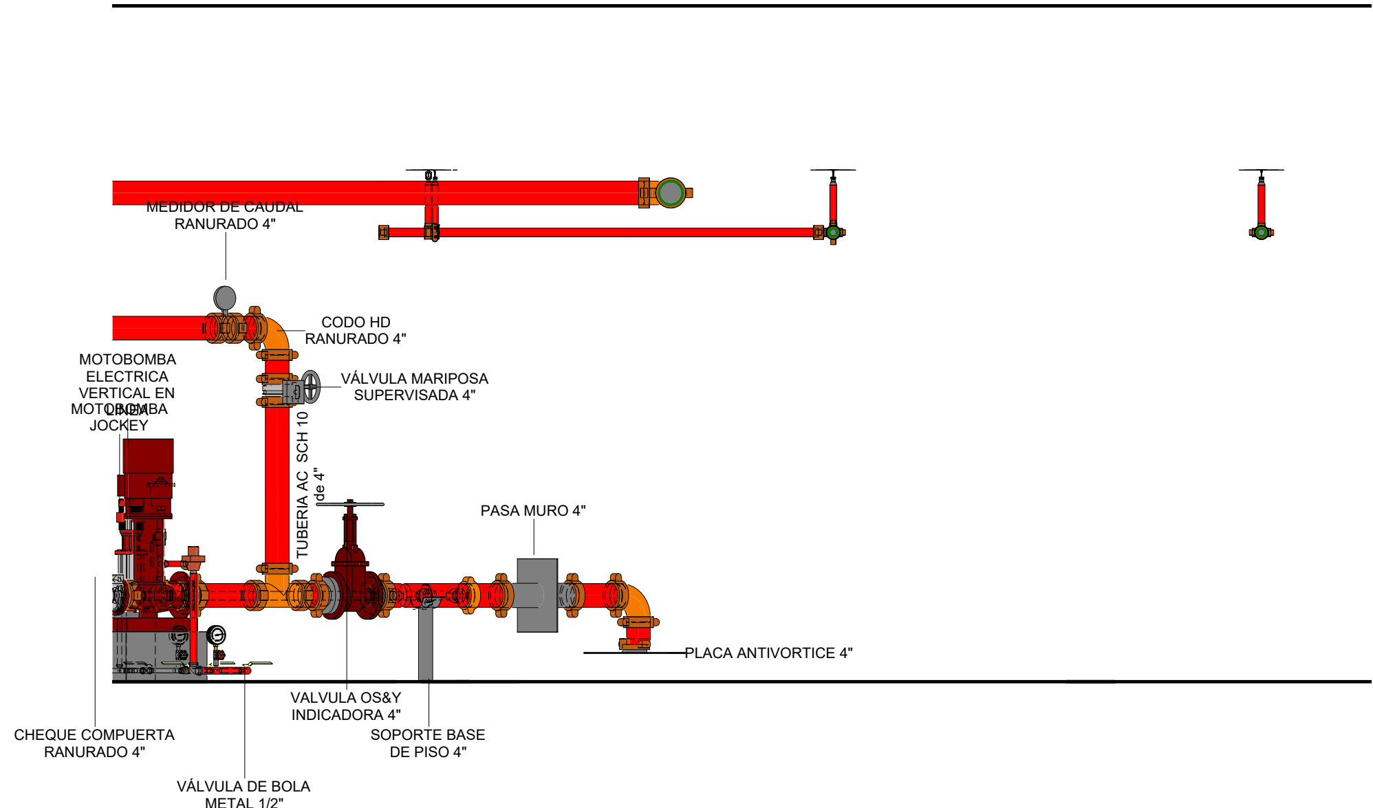
3 SECCIÓN CUARTO DE BOMBAS RCI 1 : 25
