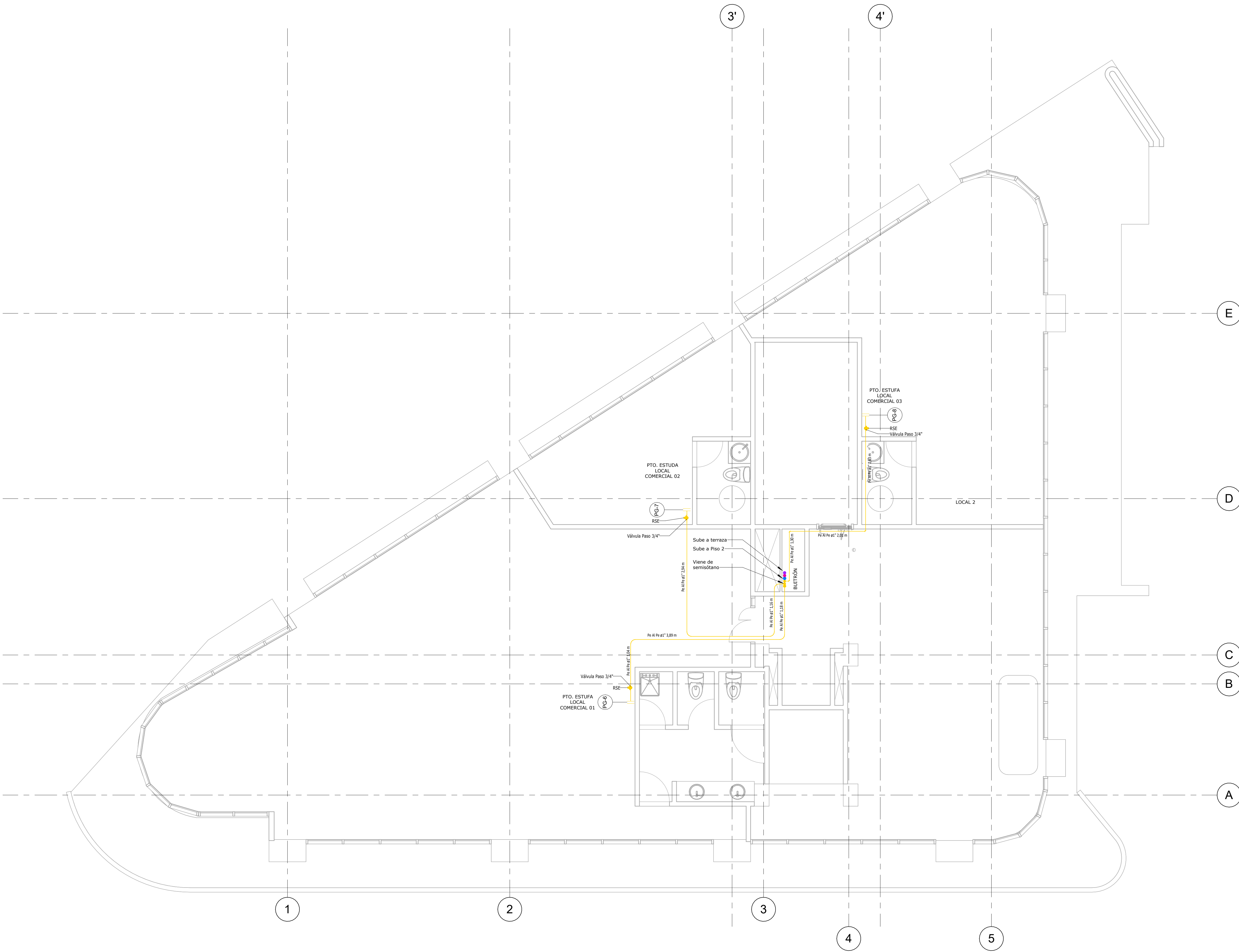
PLANTA DE PRIMER PISO RED DE GAS NATURAL 1:50
