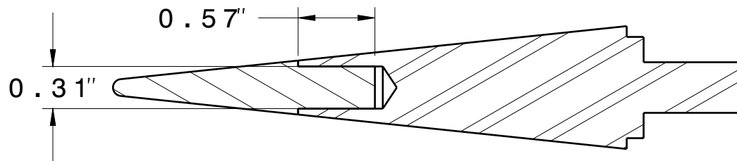
Section view A-A Scale: 1:1
