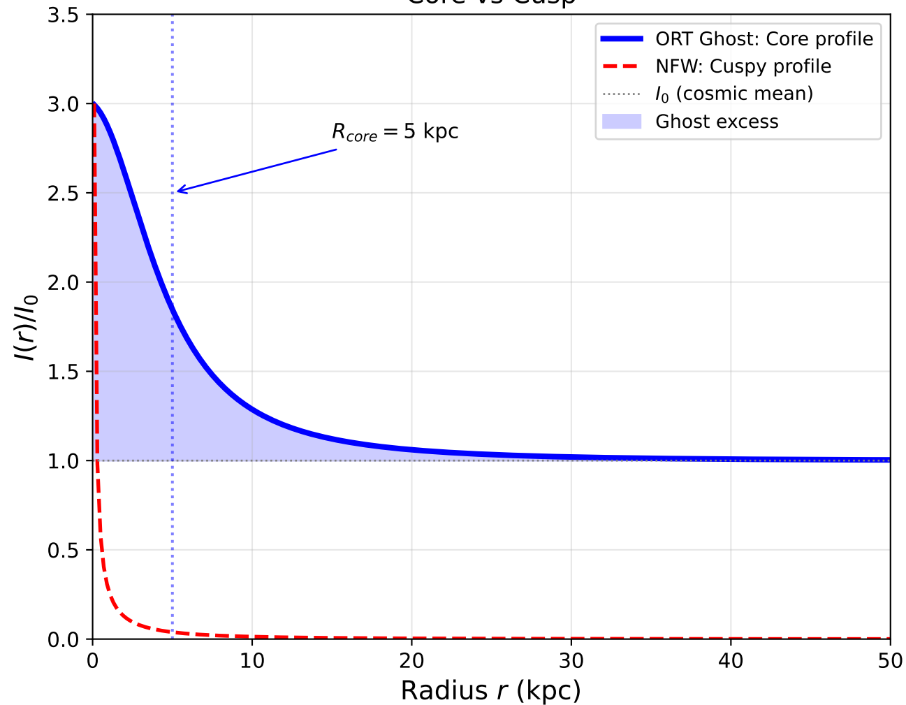
Inner Region (Linear Scale) Core vs Cusp
