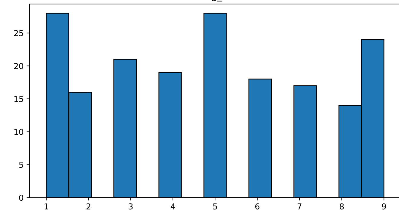
Aptitude_Test_Score
