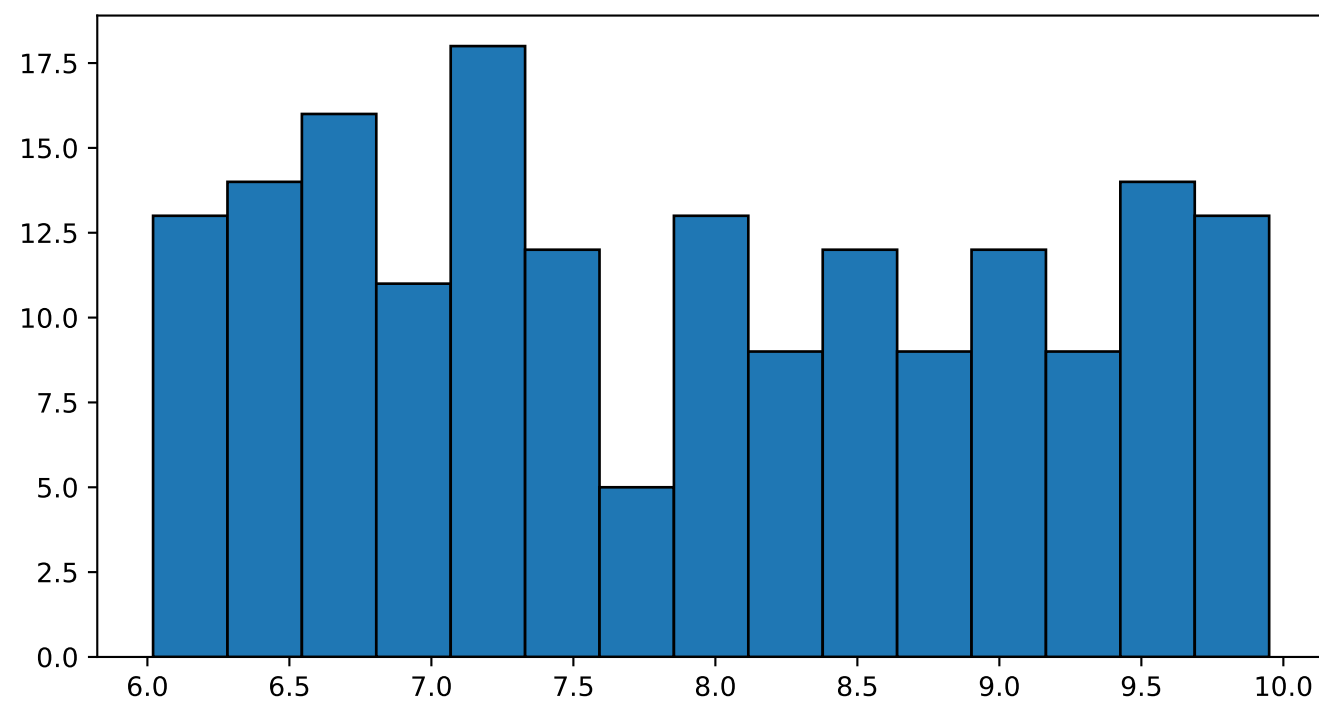
Coding_Skills
