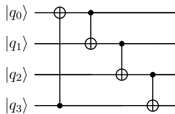
Figura 2.11. Topología de entrelazamiento circular ( circular ) sobre un circuito de 4 cúbits.
