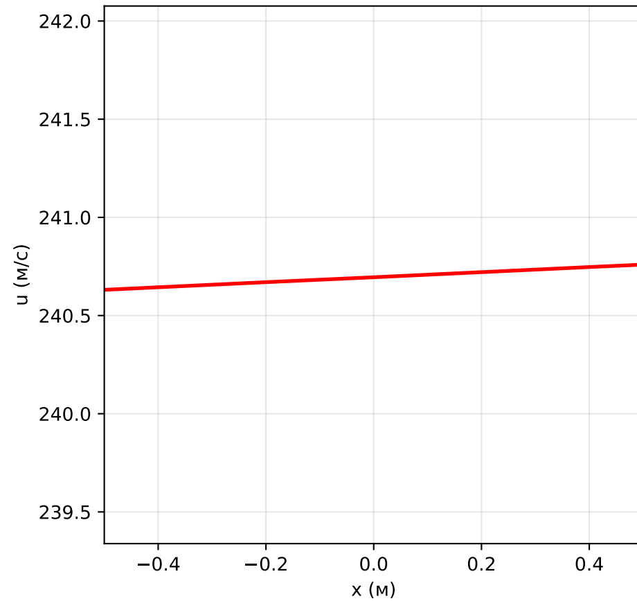
Скорость, t=0.0200 с
