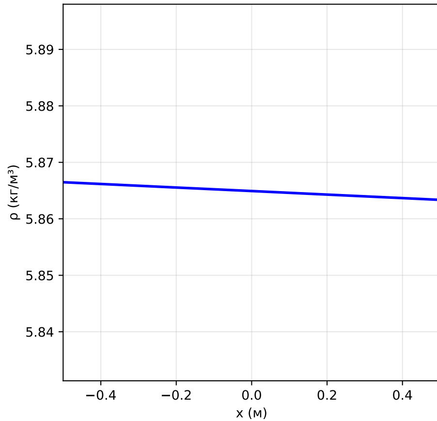
Плотность, t=0.0200 с
