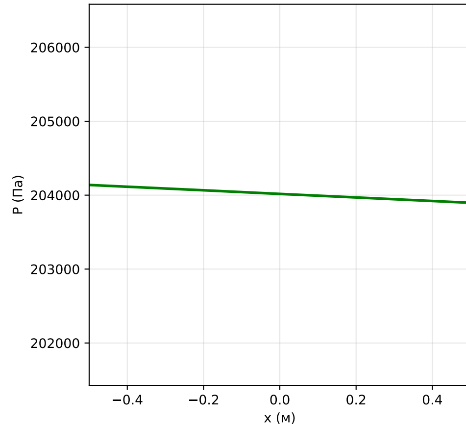
Давление, t=0.0200 с
