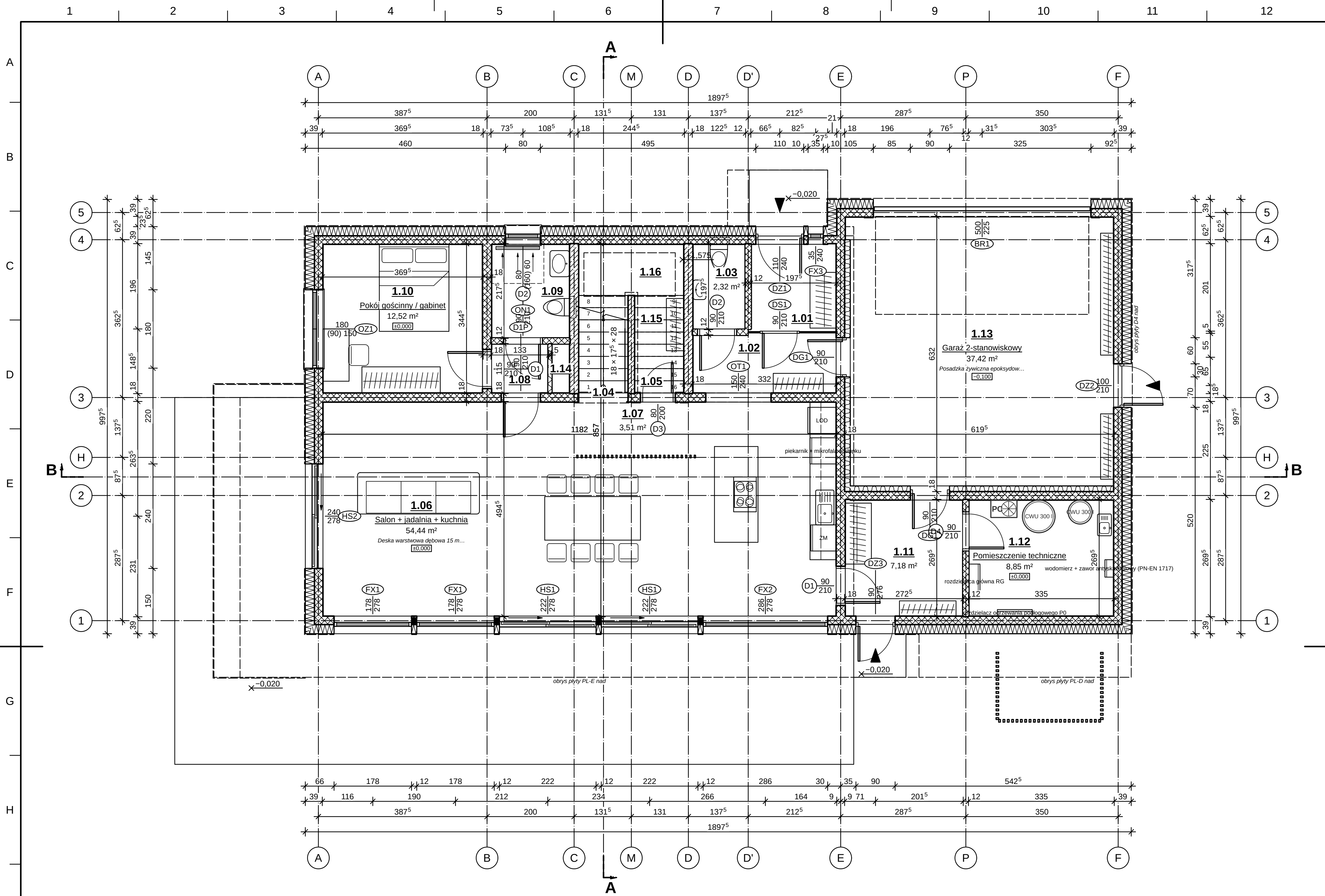
RZUT PARTERU 1:50
