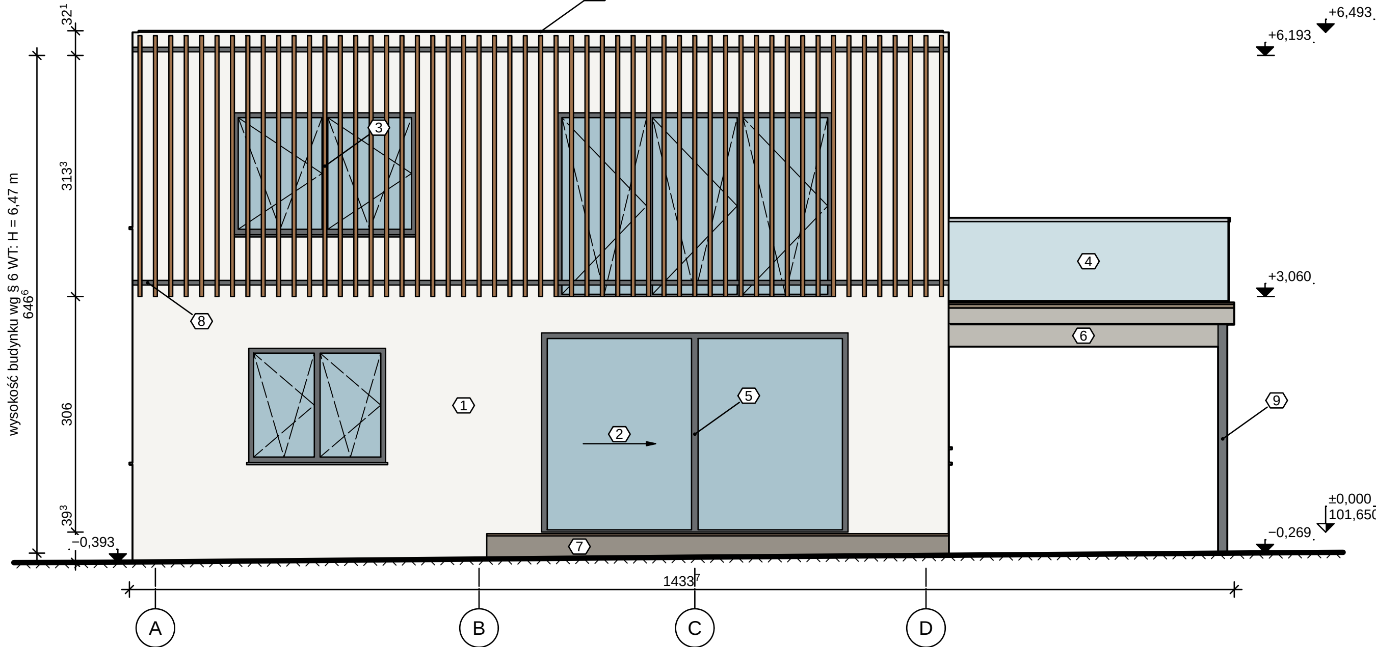
ELEWACJA POŁUDNIOWA 1:50
