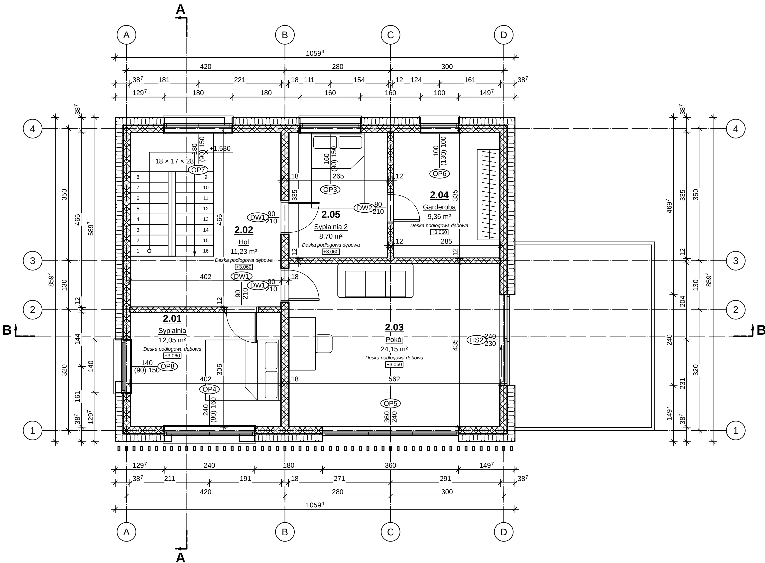
RZUT PIĘTRA 1:50
