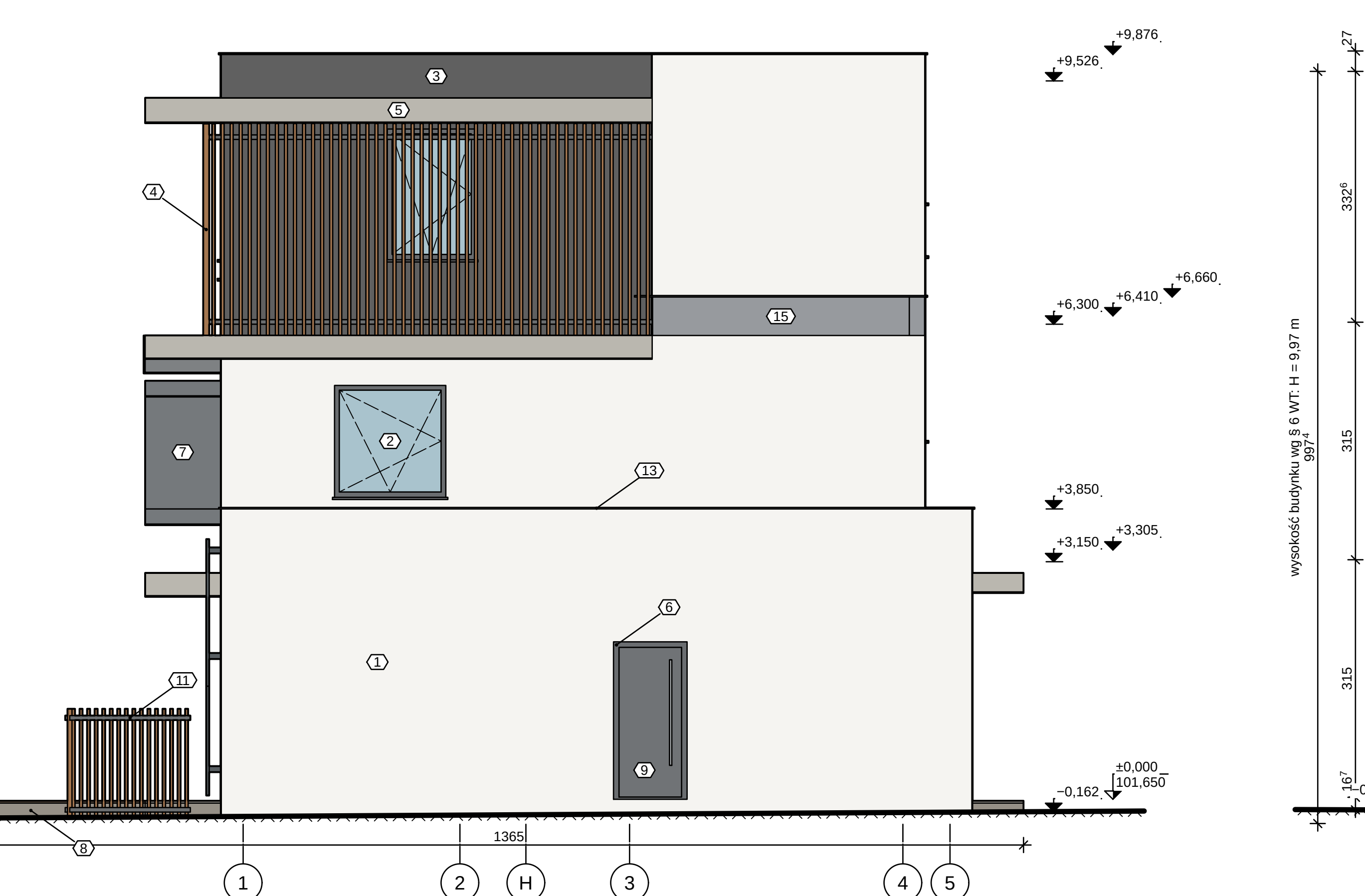
ELEWACJA WSCHODNIA 1:50
