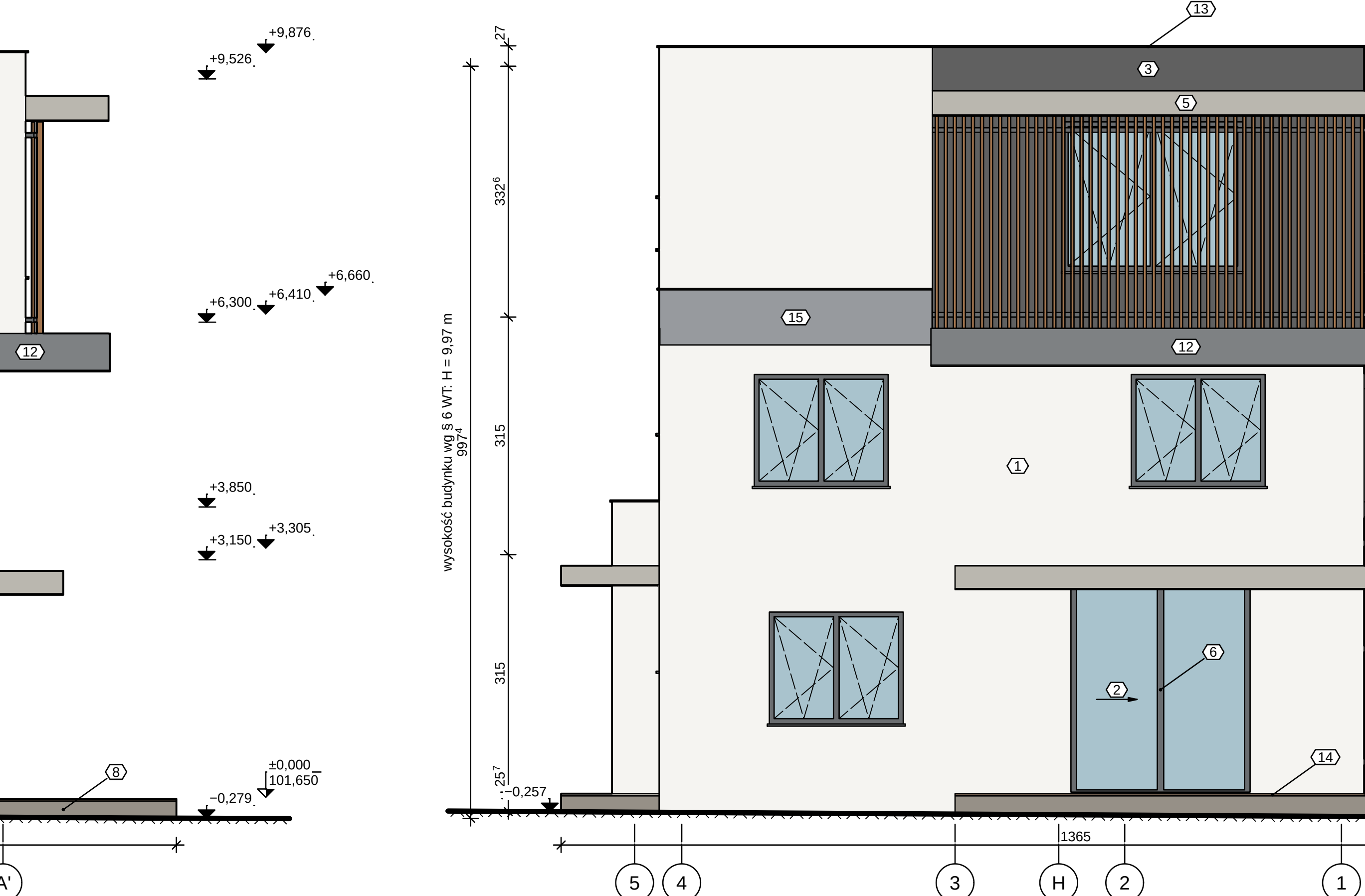
ELEWACJA ZACHODNIA 1:50
